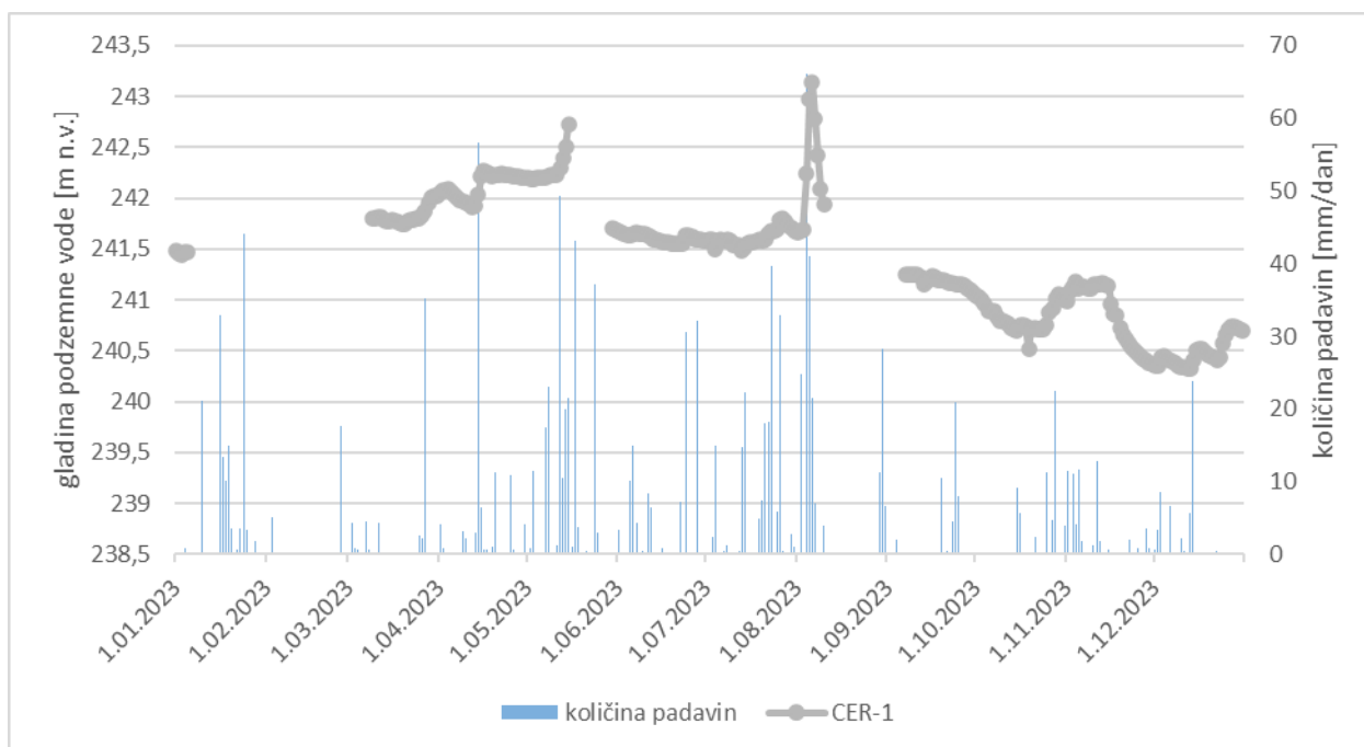
Slika 4-07: Grafični prikaz avtomatskih meritev gladin podzemne vode na merilnem mestu CER-1 (Ceršak) ter količina padavin izmerjenih na meteorološki postaji Vrbski plato v letu 2023
