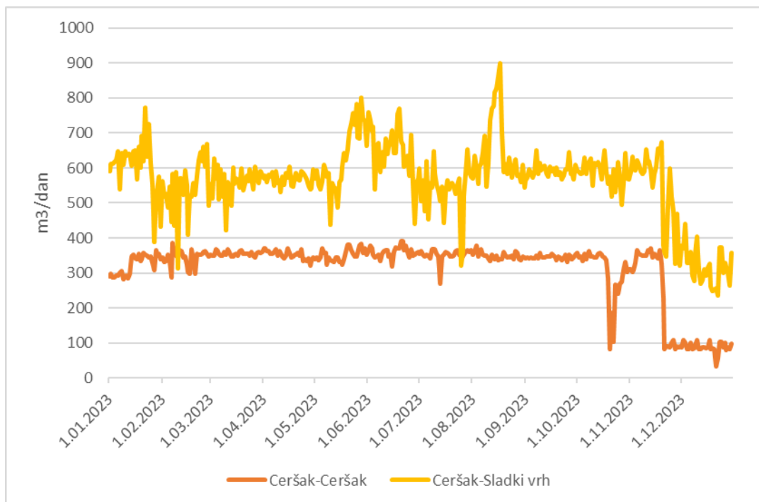
Slika 4-09: Grafični prikaz črpanih količin na območju črpališča Ceršak v letu 2023
