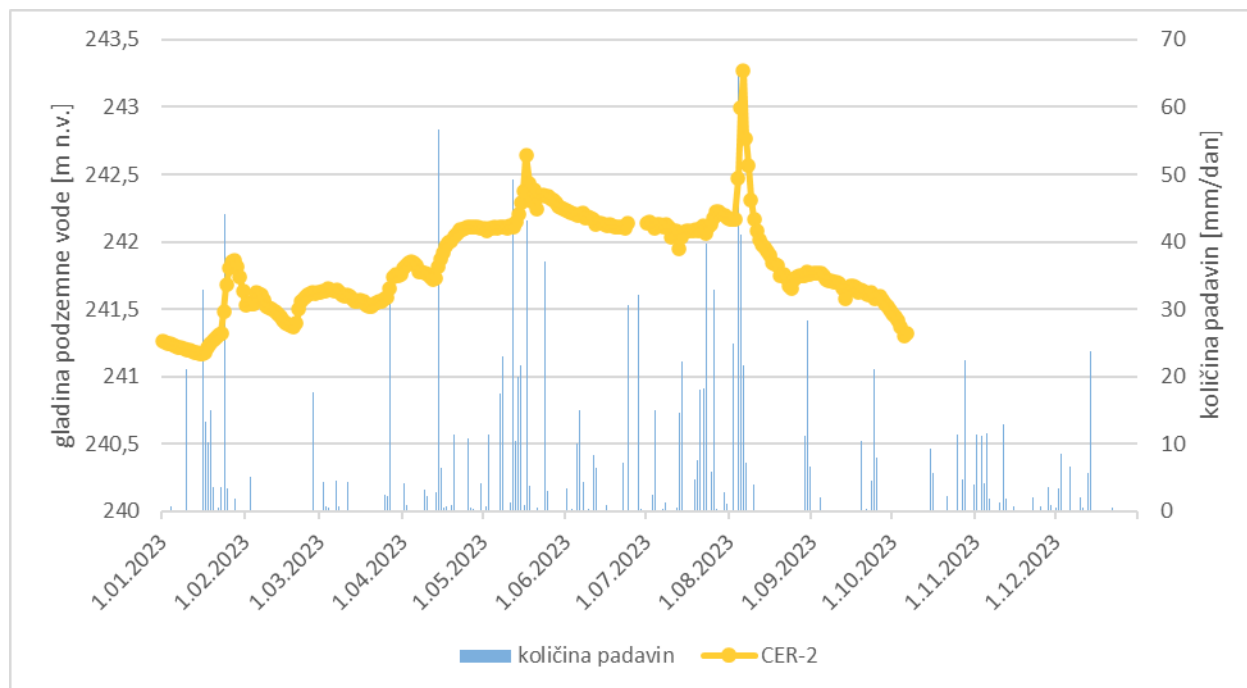
Slika 4-08 : Grafični prikaz avtomatskih meritev gladin podzemne vode na merilnem mestu CER-2 (Ceršak) ter količina padavin izmerjenih na meteorološki postaji Vrbanski plato v letu 2023
