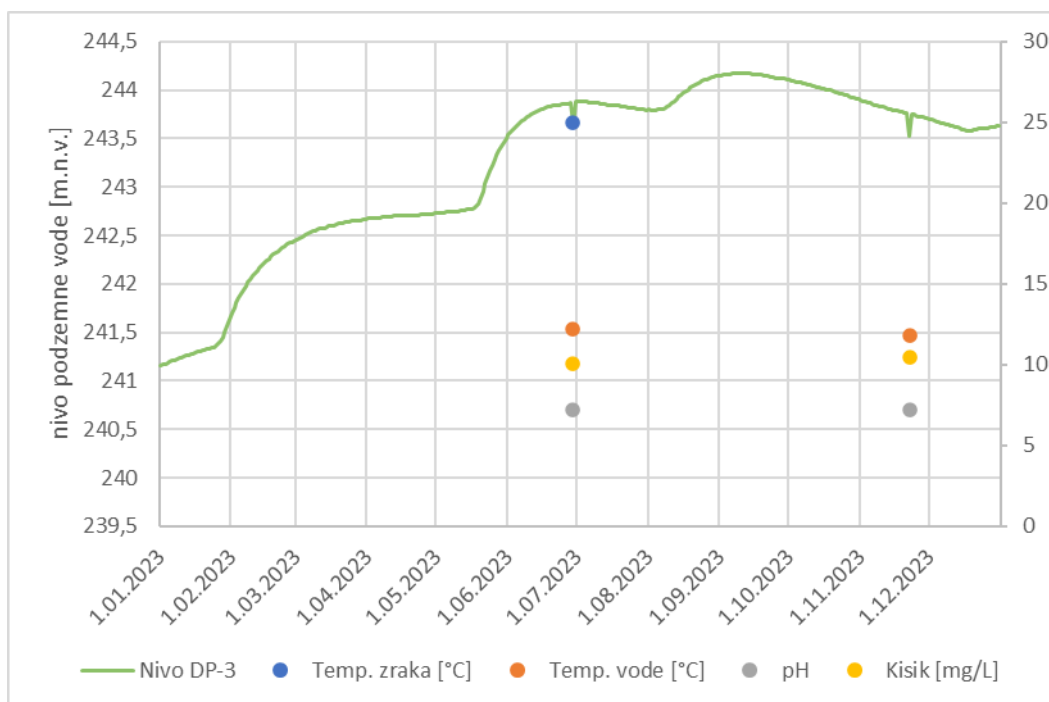
Slika 3-85: Grafični prikaz avtomatskih meritev nivojev podzemne vode na merilnem mestu VP22 ter osnovnih parametrov podzemne vode (temperatura vode, temperatura zraka, pH, kisik)
