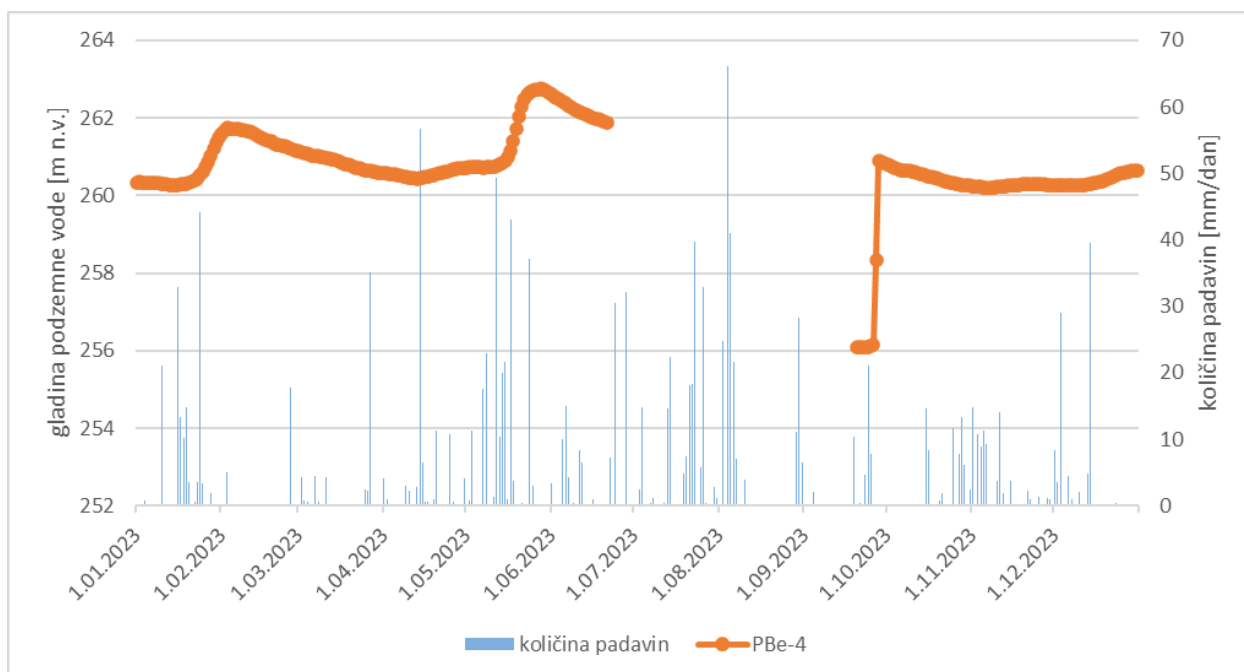
Slika 3-63: Grafični prikaz avtomatskih meritev gladin podzemne vode na merilnem mestu PBe-4 ter količine padavin izmerjenih na meteorološki postaji Letališče Edvarda Rusjana v letu 2023
