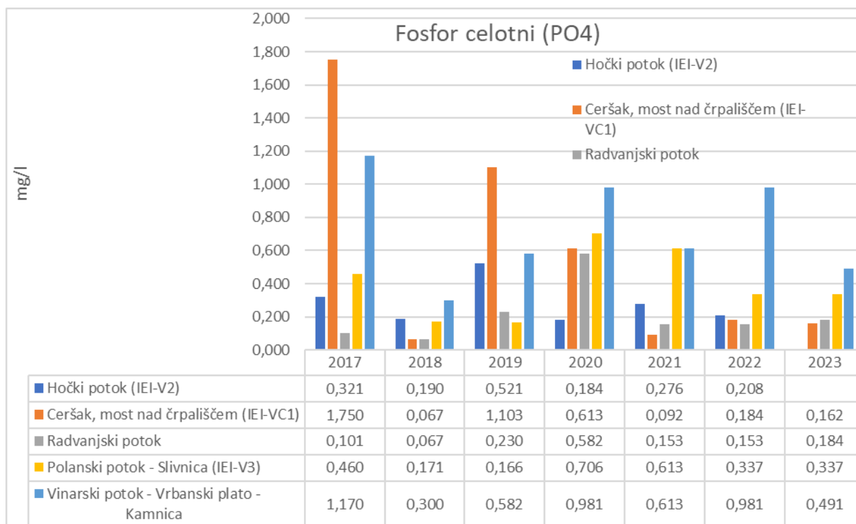
Slika 4-18: Prikaz obremenitev površinskih voda s skupnim fosforjem v letih 2017-2023
