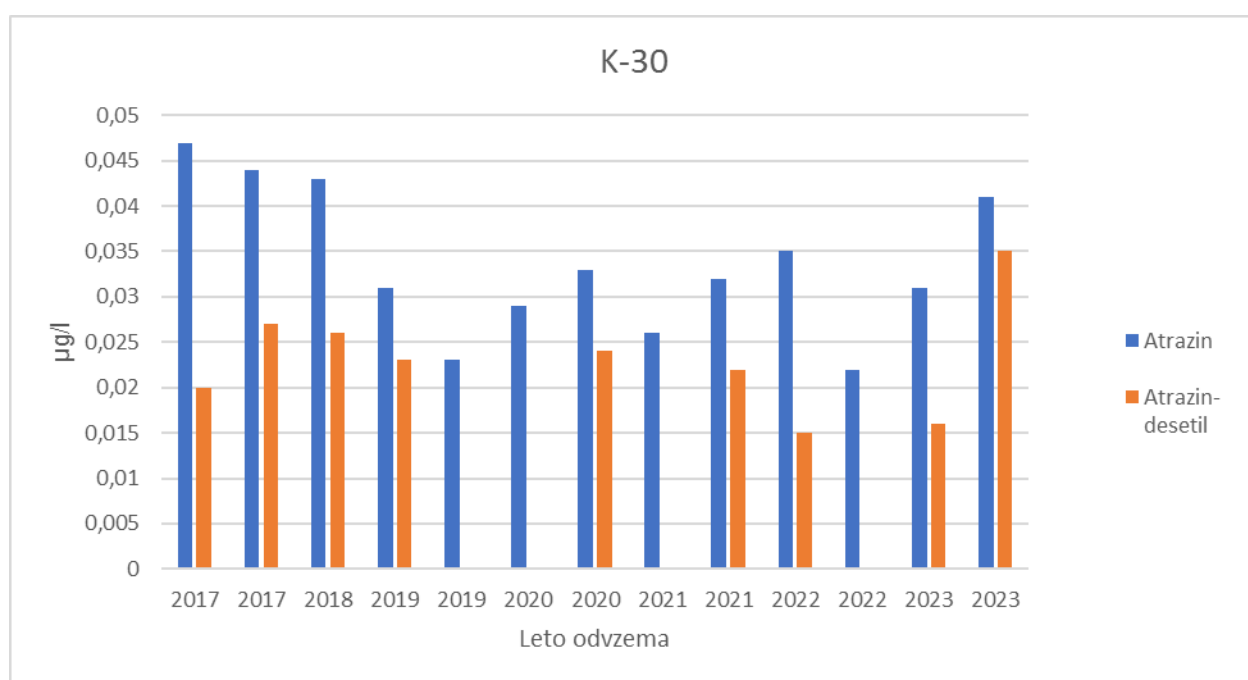
Slika 3-53: Prikaz koncentracij pesticidov (µg/l) v letih 2017-2023 na merilnem mestu K-30
