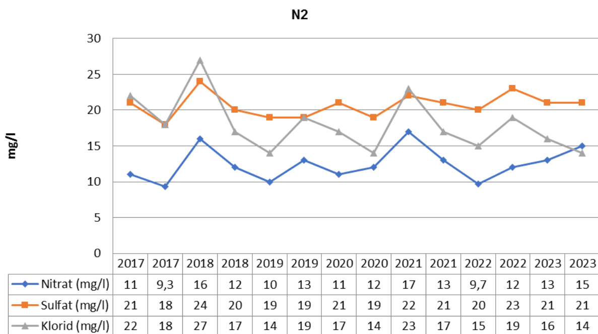
Slika 3-60: Vsebnost nitrata, sulfata in klorida (mg/l) v podzemni vodi na merilnem mestu N-2 v letih 2017-2023
