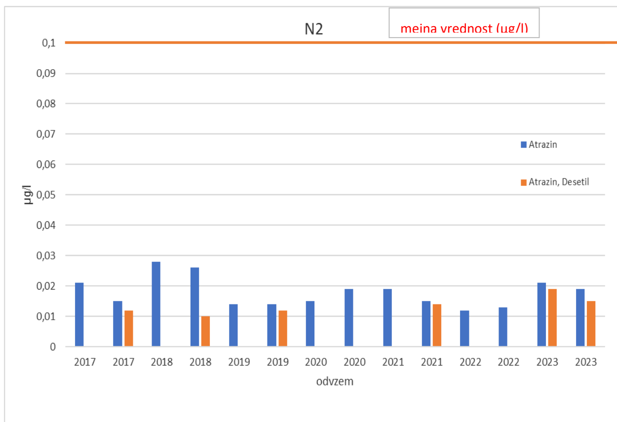
Slika 3-61: Vsebnost pesticidov (µg/l) v podzemni vodi na merilnem mestu N-2 v letih 2017-2023
