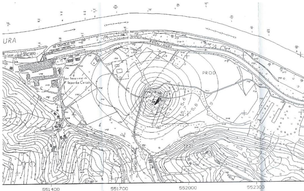
Slika 4-06: Ocenjene hidroizohipse na območju črpališča v Ceršaku
