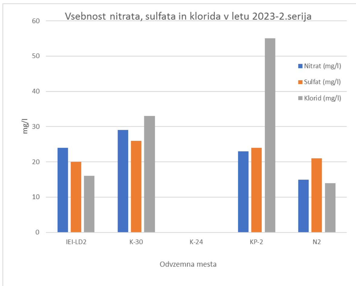
Slika 3-47: Vsebnosti nitrata, sulfata in klorida(mg/l) v jesenskem vzorčenju 2023
