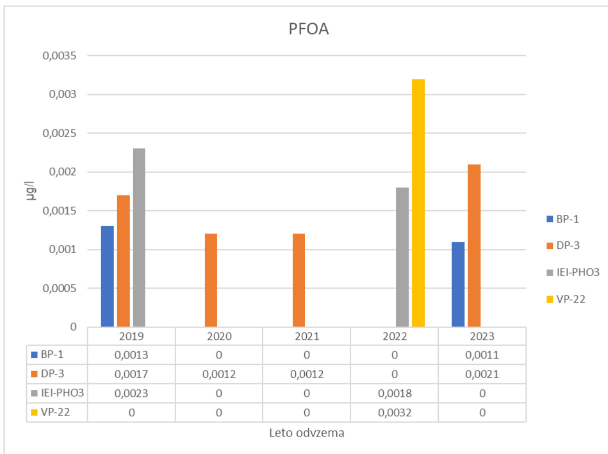
Slika 3-94: Izmerjene koncentracije PFOA na odzemnih mestih BP-1, DP-3, IEI-PHO3 ter VP-22 v letih 2019-2023
