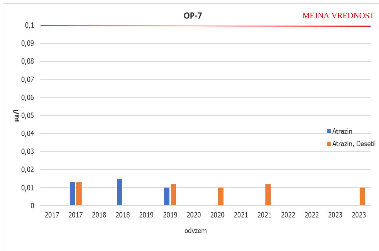
Slika 3-71: Vsebnost pesticidov atrazina in desetil-atrazina (µg/l) v podzemni vodi na merilnem mestu OP-7 v letih 2017-2023
