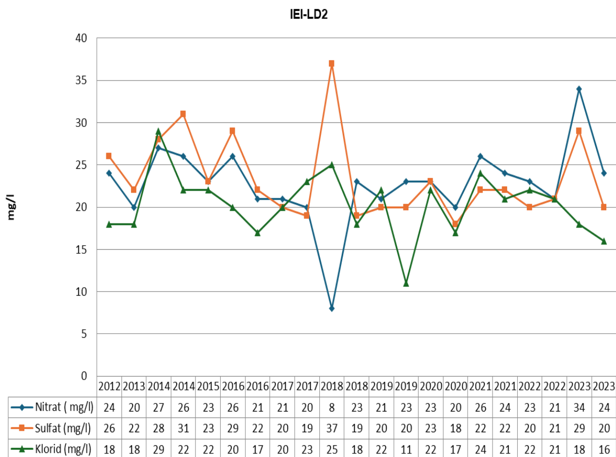
Slika 3-54: Vsebnost nitrata, sulfata in klorida (mg/l) v podzemni vodi na merilnem mestu IEI-LD2 v letih 2012-2023
