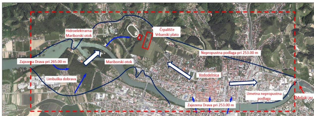
Slika 3-35: Vodonosnik Vrbanskega platoja (Kopač, Vremec, 2017)
