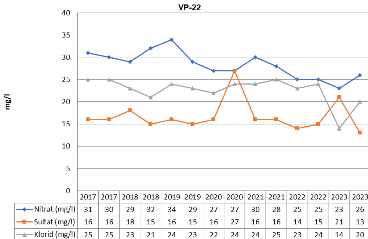
Slika 3-89: Vsebnost nitrata, sulfata in klorida (mg/l) v podzemni vodi na opazovalni vrtini VP-22 v letih 2017-2023
