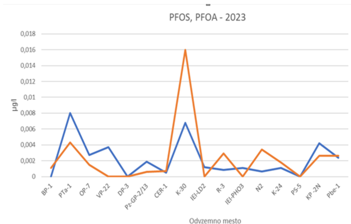
Slika 2-9: Ugotovljena prisotnost PFOS in PFOA v letu 2023
