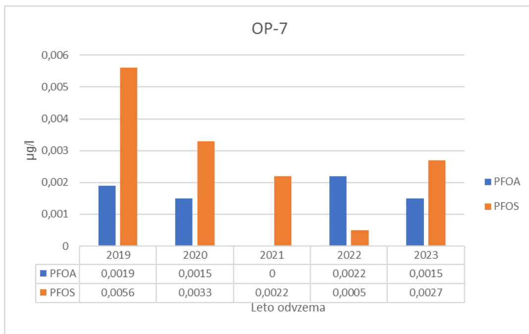
Slika 3-68: Izmerjene koncentracije PFOA in PFOS na odvzemnem mestu OP-7 v letih 2019-2023
