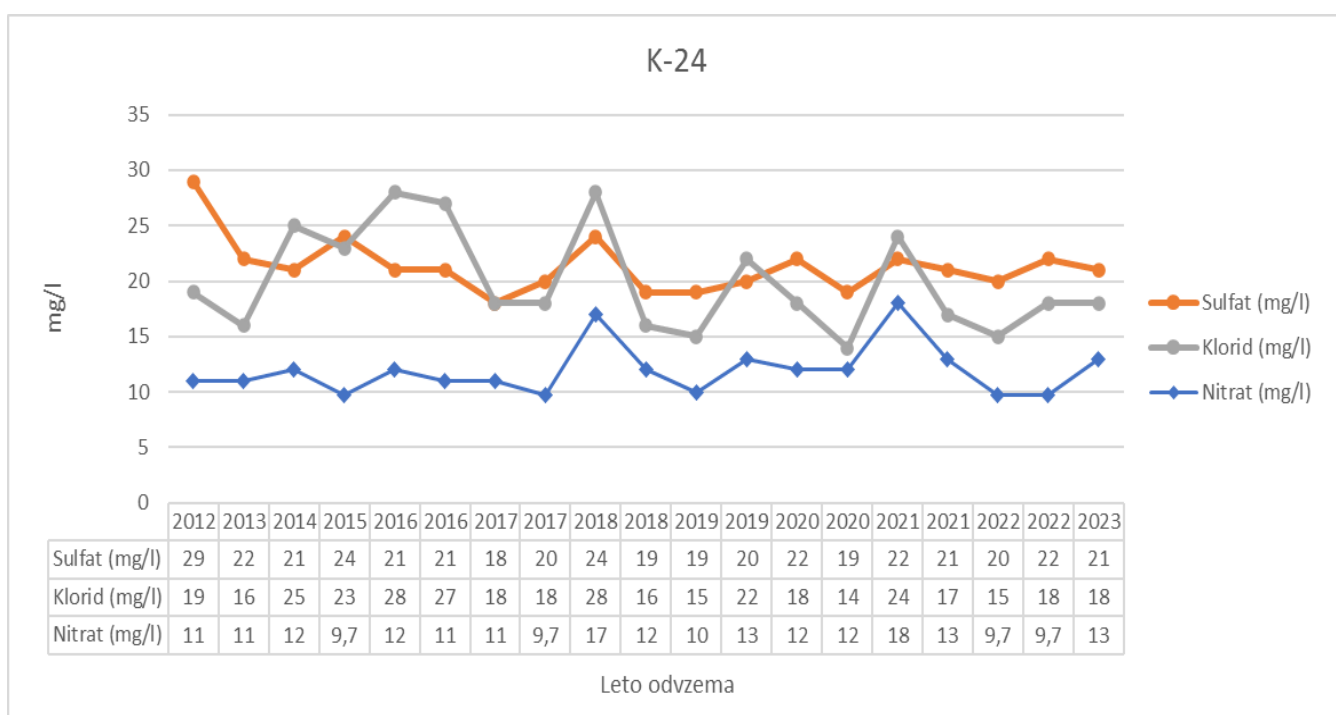
Slika 3-48: Vsebnost nitrata, sulfata in klorida (mg/l) v podzemni vodi na merilnem mestu K-24 v letih 2012-2023
