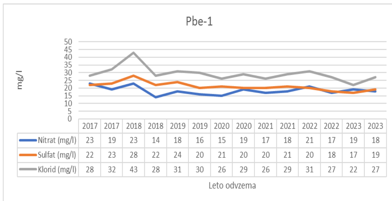
Slika 3-67: Nihanje vsebnosti nitrata in klorida (mg/l) na merilnem mestu Pbe-1 v letih 2017-2023
