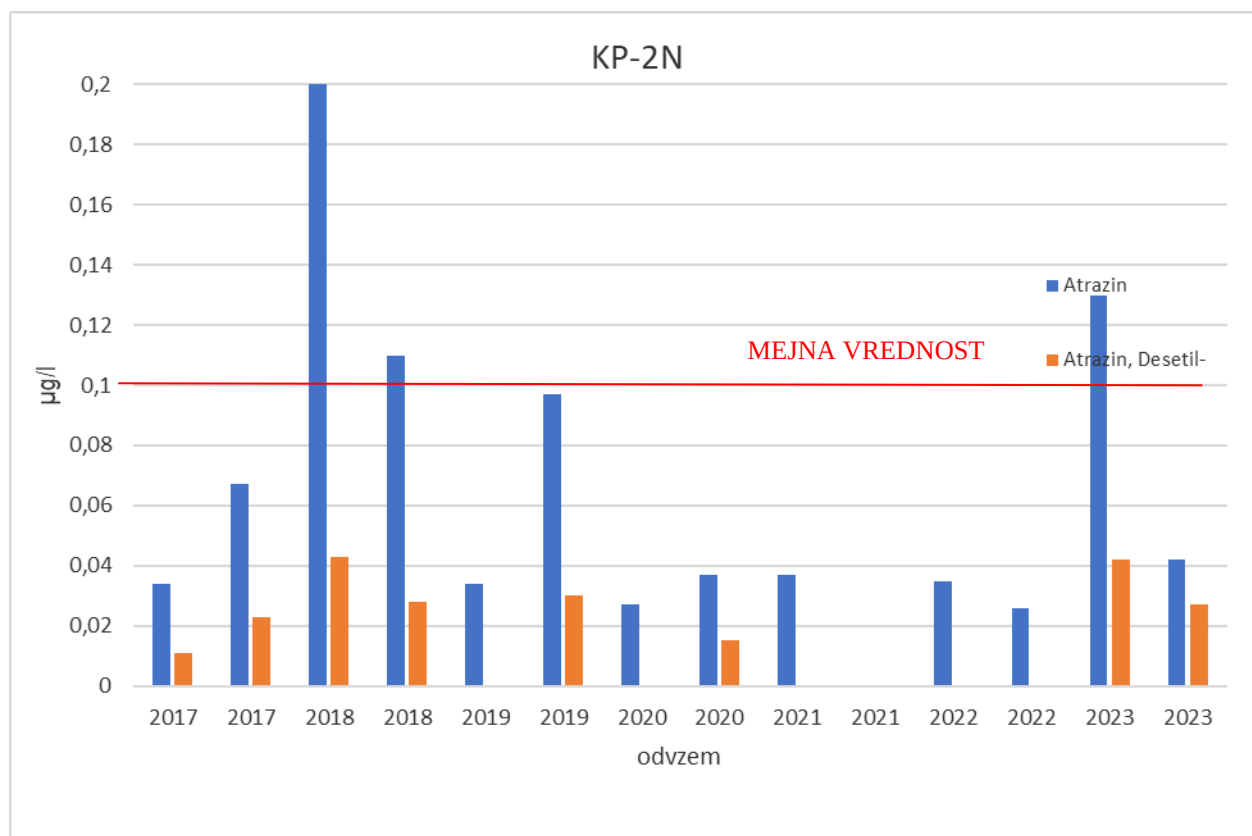
Slika 3-58: Vsebnost pesticidov (µg/l) v podzemni vodi na merilnem mestu KP-2N v letih 2017-2023
