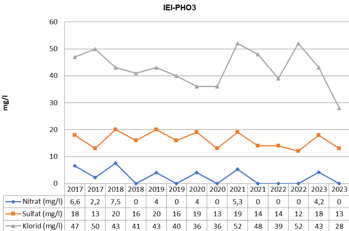
Slika 3-88: Vsebnost nitrata, sulfata in klorida (mg/l) v podzemni vodi na opazovalni vrtini IEI-PHO3 v letih 2017-2023
