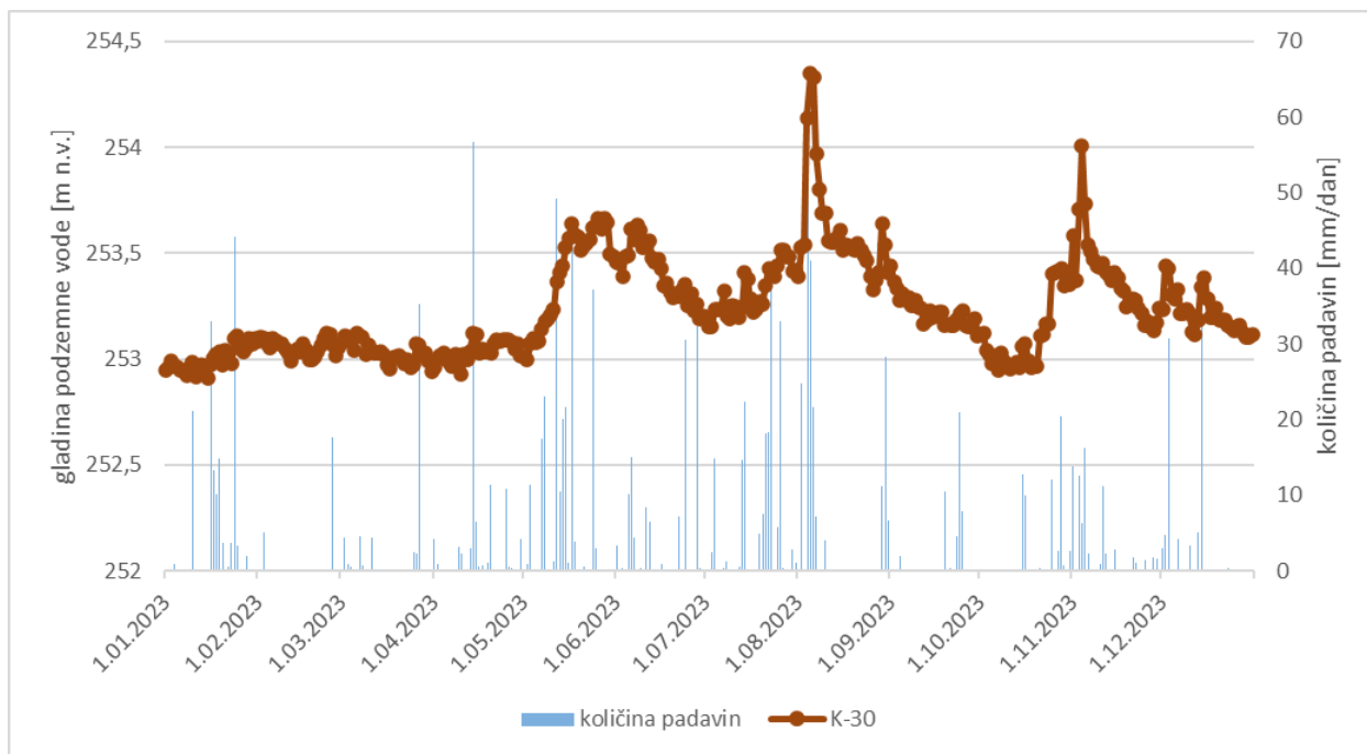
Slika 3-37: Grafični prikaz avtomatskih meritev gladin podzemne vode na merilnem mestu K-30 ter količine padavin izmerjenih na meteorološki postaji Vrbanski plato v letu 2023
