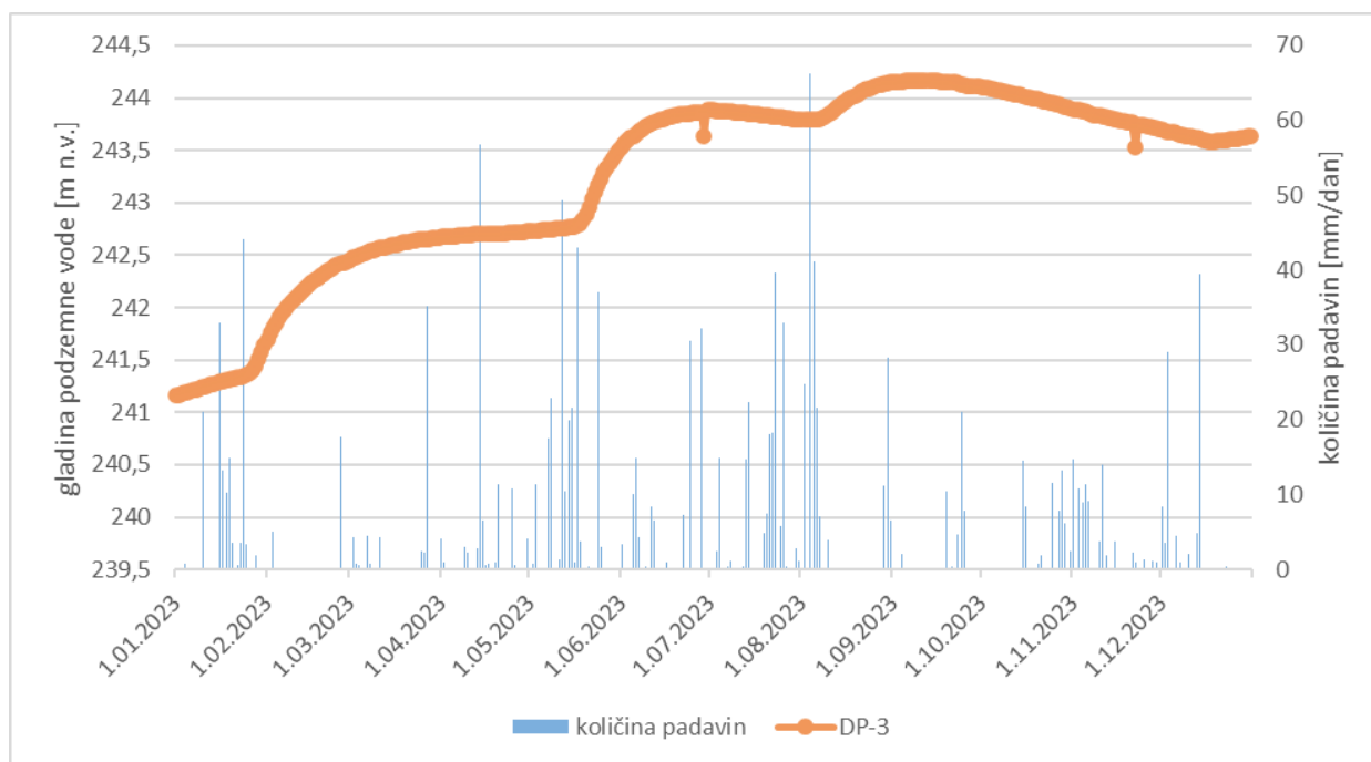
Slika 4-03: Grafični prikaz avtomatskih meritev gladin podzemne vode na merilnem mestu DP-3 (Dobrovce) ter količine padavin izmerjenih na meteorološki postaji Vrbanski plato v letu 2023
