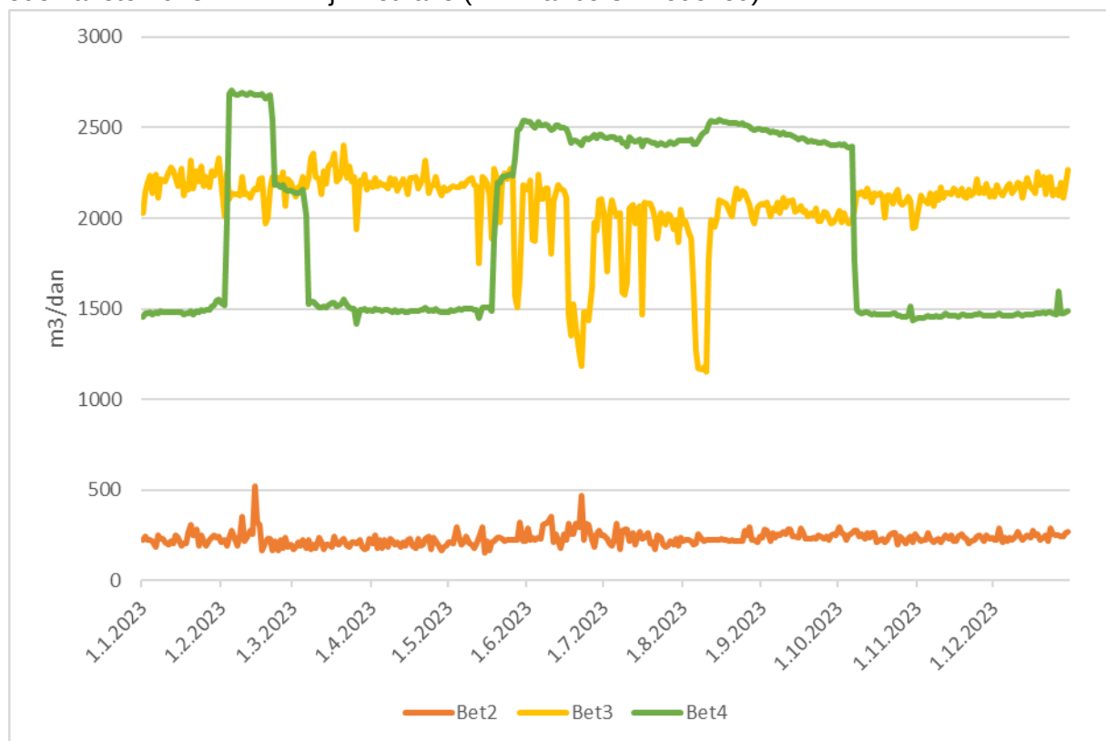
Slika 3-75: Grafični prikaz črpanih količin podzemne vode na območju črpališča Betnava v letu 2023
