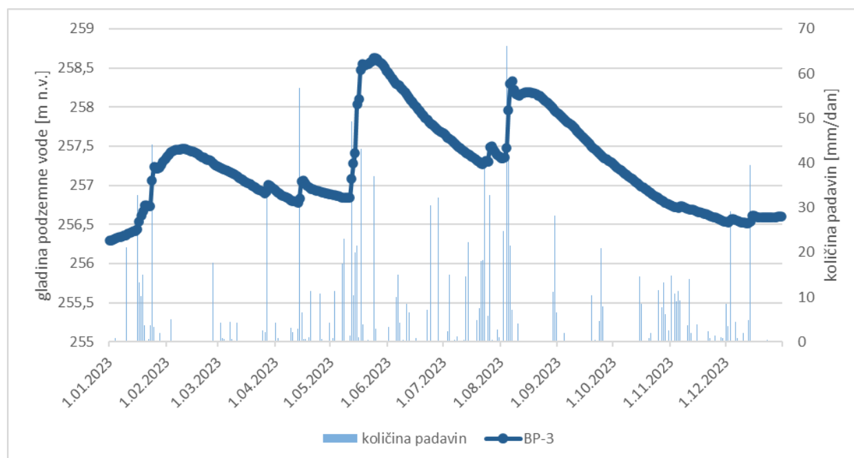
Slika 4-02: Grafični prikaz avtomatskih meritev gladin podzemne vode na merilnem mestu BP-3 (Bohova) ter količine padavin izmerjenih na meteorološki postaji letališče Vrbanjski plato v letu 2023
