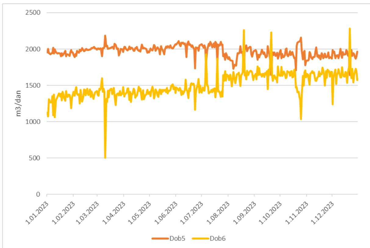
Slika 3-99: Grafični prikaz črpanih količin podzemne vode na območju črpališča Dobrovci v letu 2023
