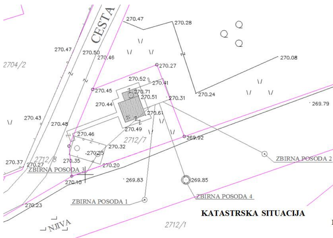
Slika 3-14: Objekti lizimetske postaje Tezno
