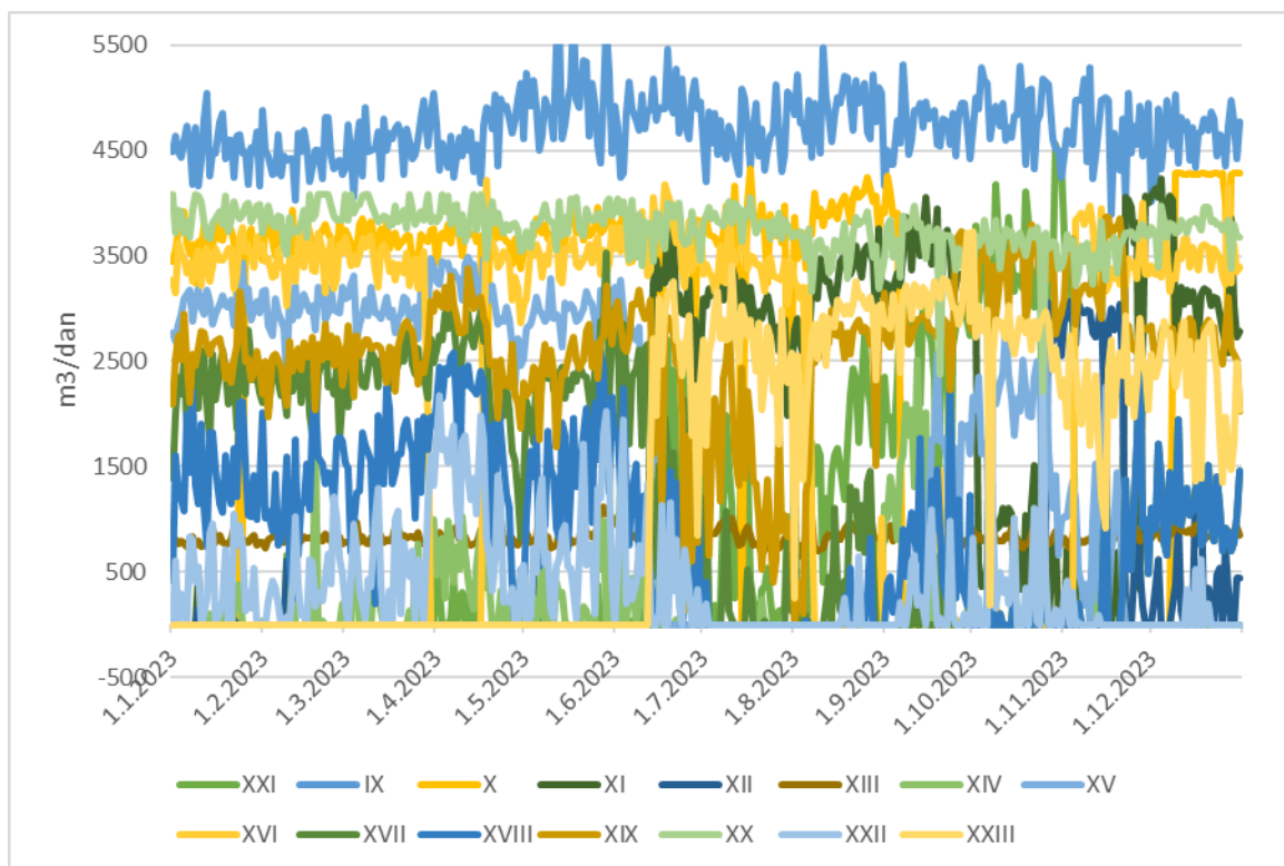
Slika 3-39: Grafični prikaz črpanih količin podzemne vode na območju črpališča Vrbanski Plato
