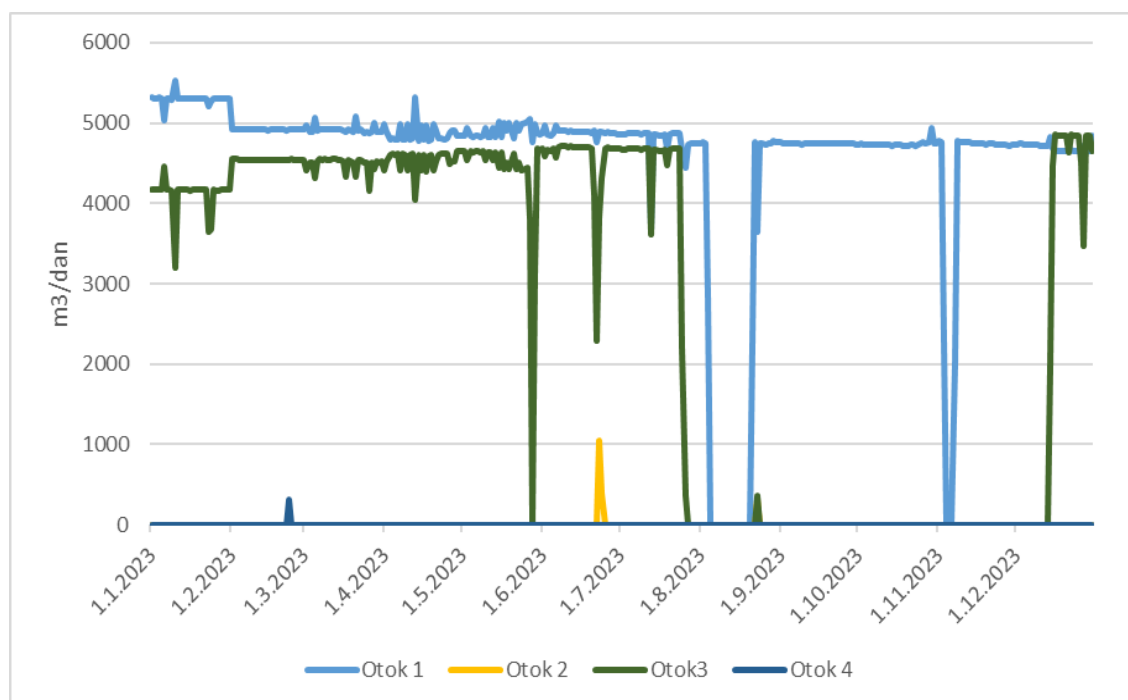
Slika 3-41: Grafični prikaz črpanih količin podzemne vode na območju Mariborskega otoka
