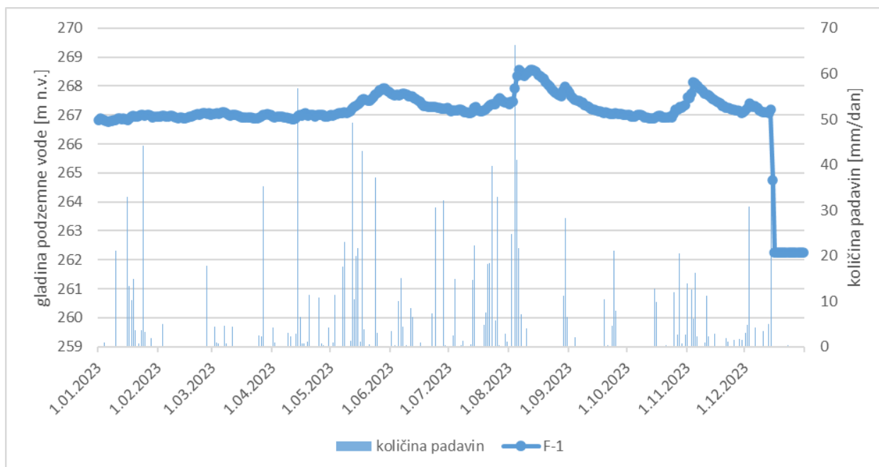
Slika 3-21: Grafični prikaz avtomatskih meritev gladin podzemne vode na merilnem mestu F-1 in količina padavin izmerjenih na meteorološki postaji Vrbanski plato v letu 2023
