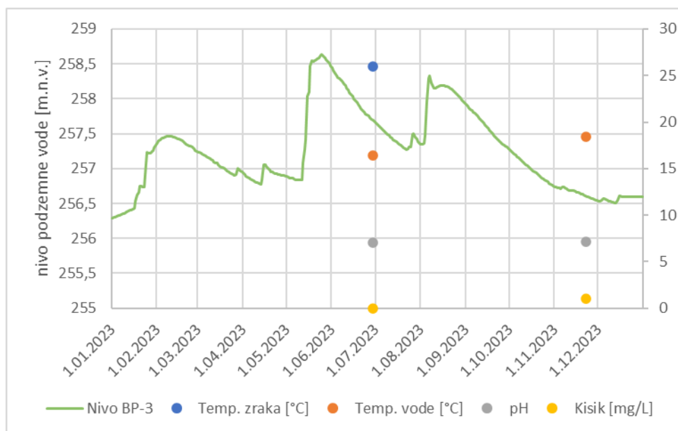
Slika 3-81: Grafični prikaz avtomatskih meritev nivojev podzemne vode na merilnem mestu BP-1 ter osnovnih parametrov podzemne vode (temperatura vode, temperatura zraka, pH, kisik)
