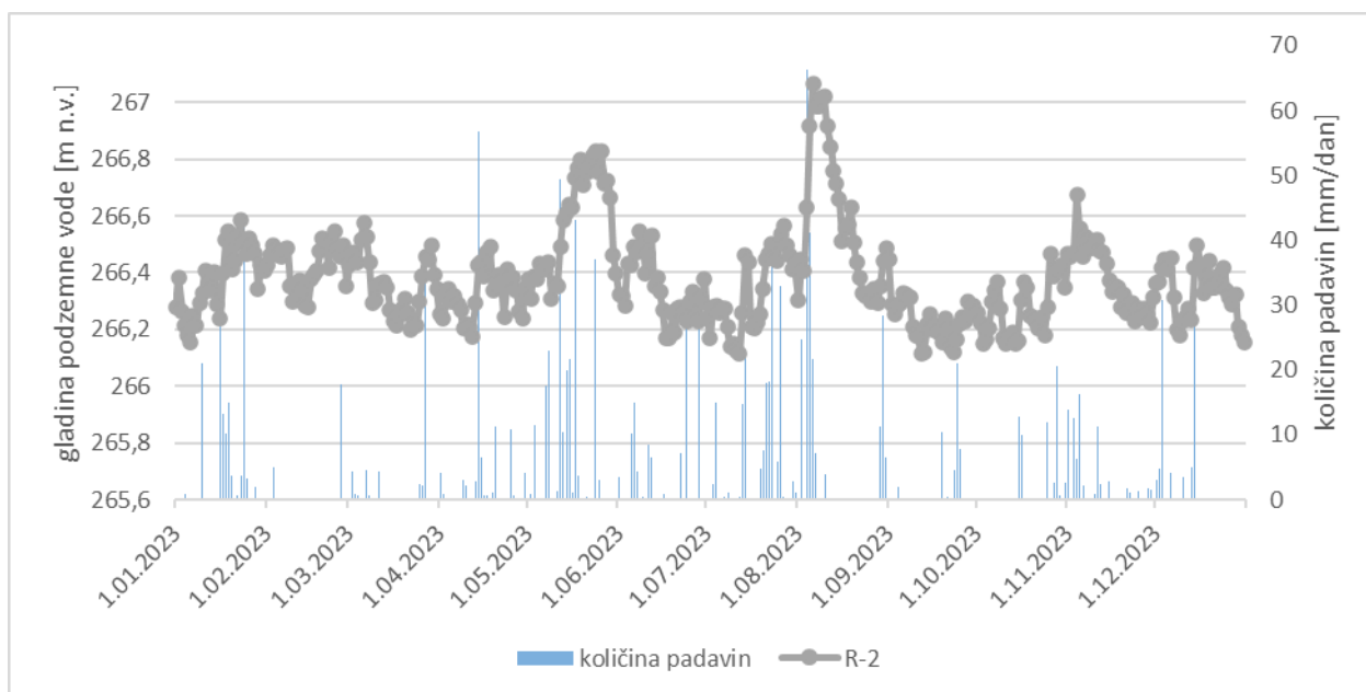
Slika 3-2: Grafični prikaz avtomatskih meritev gladin podzemne vode na merilnem mestu R-2 (Ruše) in količina padavin izmerjenih na meteorološki postaji Vrbanski plato v letu 2023
