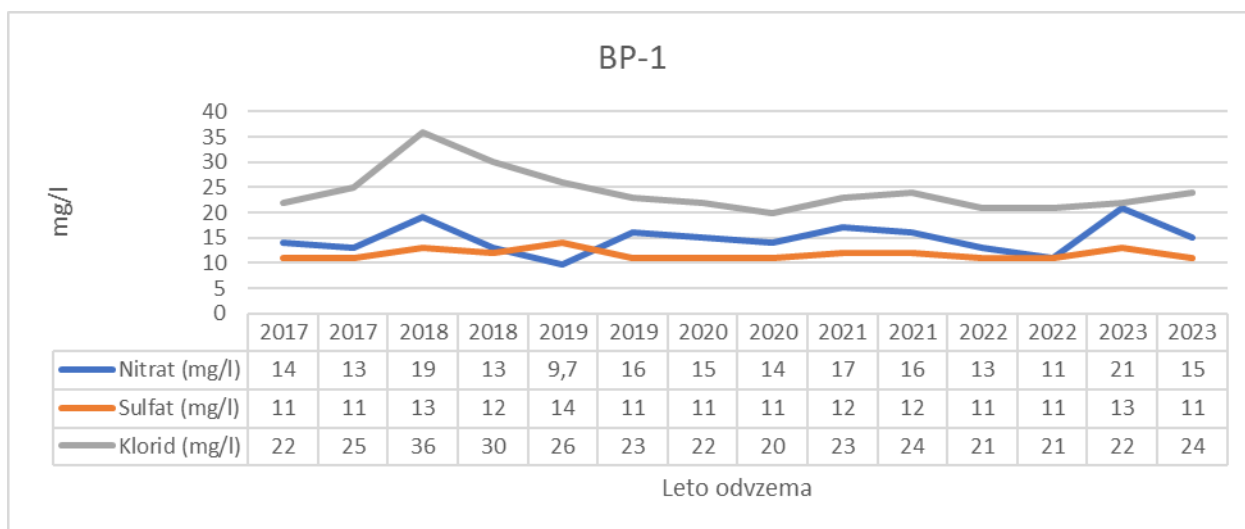
Slika 3-86: Vsebnost nitrata, sulfata in klorida (mg/l) v podzemni vodi na opazovalni vrtini BP-1 v letih 2017-2023
