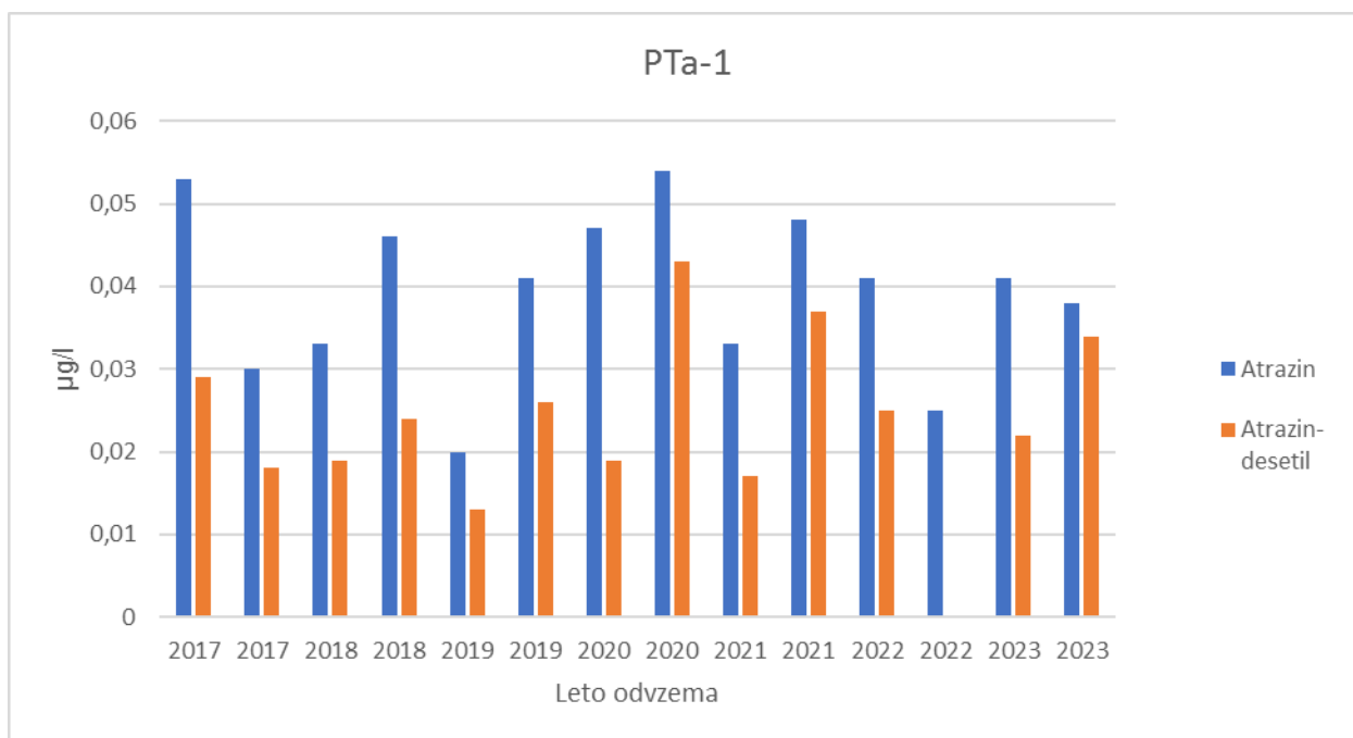
Slika 3-73: Vsebnost pesticidov atrazina, desetil-atrazina ( \mu\text{g/l} ) v podzemni vodi na merilnem mestu PTa-1 v letih 2017-2023
