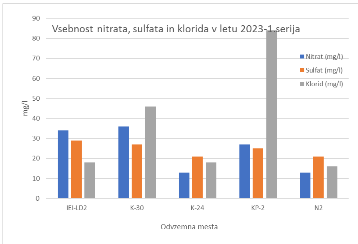
Slika 3-46: Vsebnosti nitrata, sulfata in klorida(mg/l) v spomladanskem vzorčenju 2023
