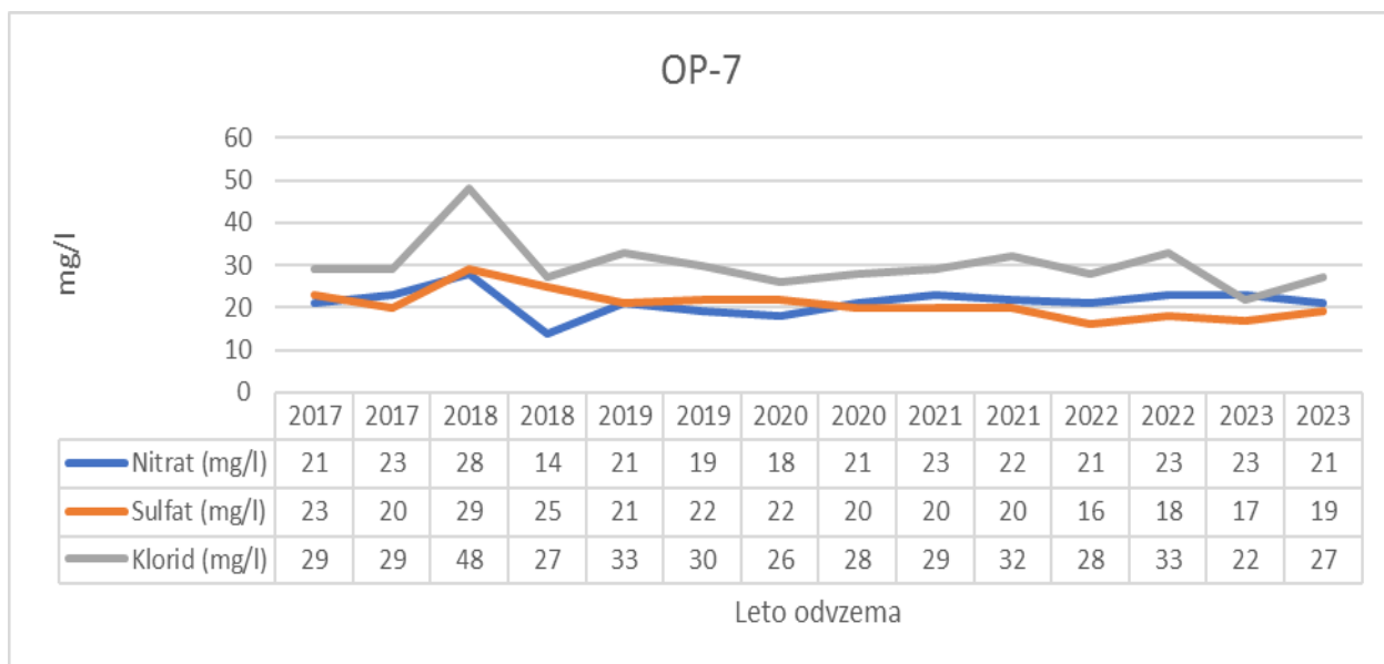
Slika 3-65: Nihanje vsebnosti nitrata, klorida in sulfata (mg/l) na merilnem mestu OP-7 v letih 2017-2023
