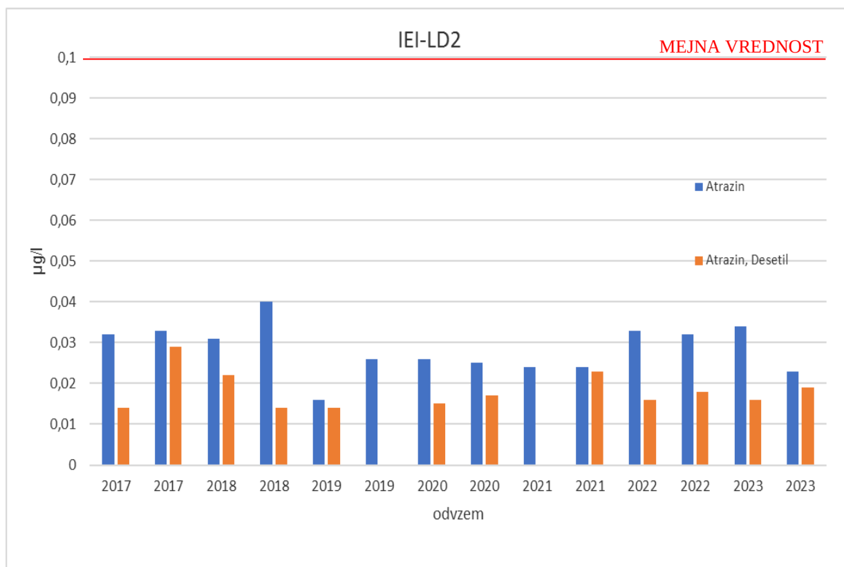
Slika 3-55 Izmerjene vrednosti atrazina in desetil-atrazina v letih 2017-2023 na odzemnem mestu IEI-LD2
