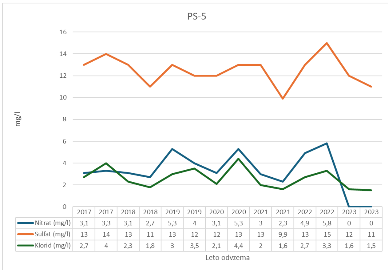
Slika 3-25: Vsebnost nitrata, sulfata in klorida (mg/l) v podzemni vodi na merilnem mestu PS-5 v letih 2017-2023
