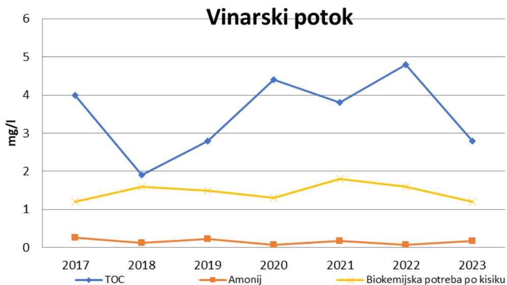
Slika 4-23: Prikaz nihanja osnovnih kemijskih parametrov na odvzemnem mestu Vinarski potok v letih 2017-2023
