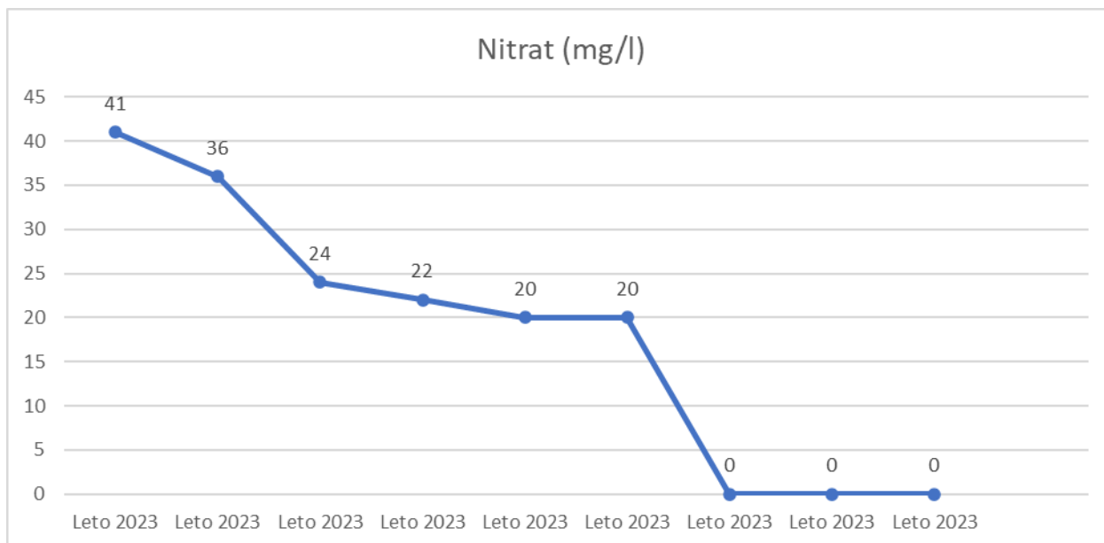
Slika 3-15: izmerjene vsebnosti nitrata (mg/l) v vzorcih odvzetih na lizimeterski postaji Tezno v letu 2023
