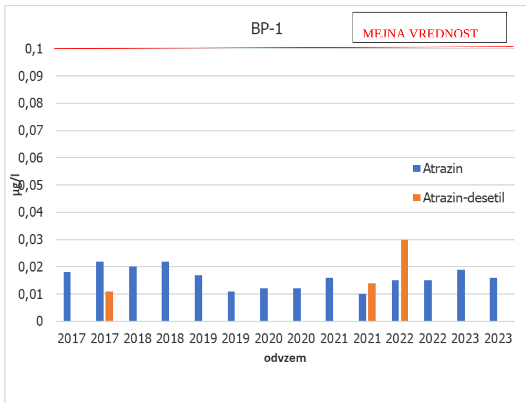
Slika 3-90: Vsebnost atrazina in atrazin-desetila (µg/l) v podzemni vodi na opazovalni vrtini BP-1 v letih 2017-2023
