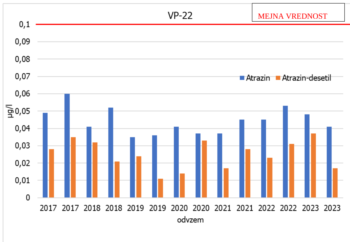
Slika 3-93: Vsebnost atrazina, atrazin-desetila, terbutilazina ter metabolita metolaklor OXA in metaloklor ESA (µg/l) v podzemni vodi na opazovalni vrtini VP-22 v letih 2017-2023
