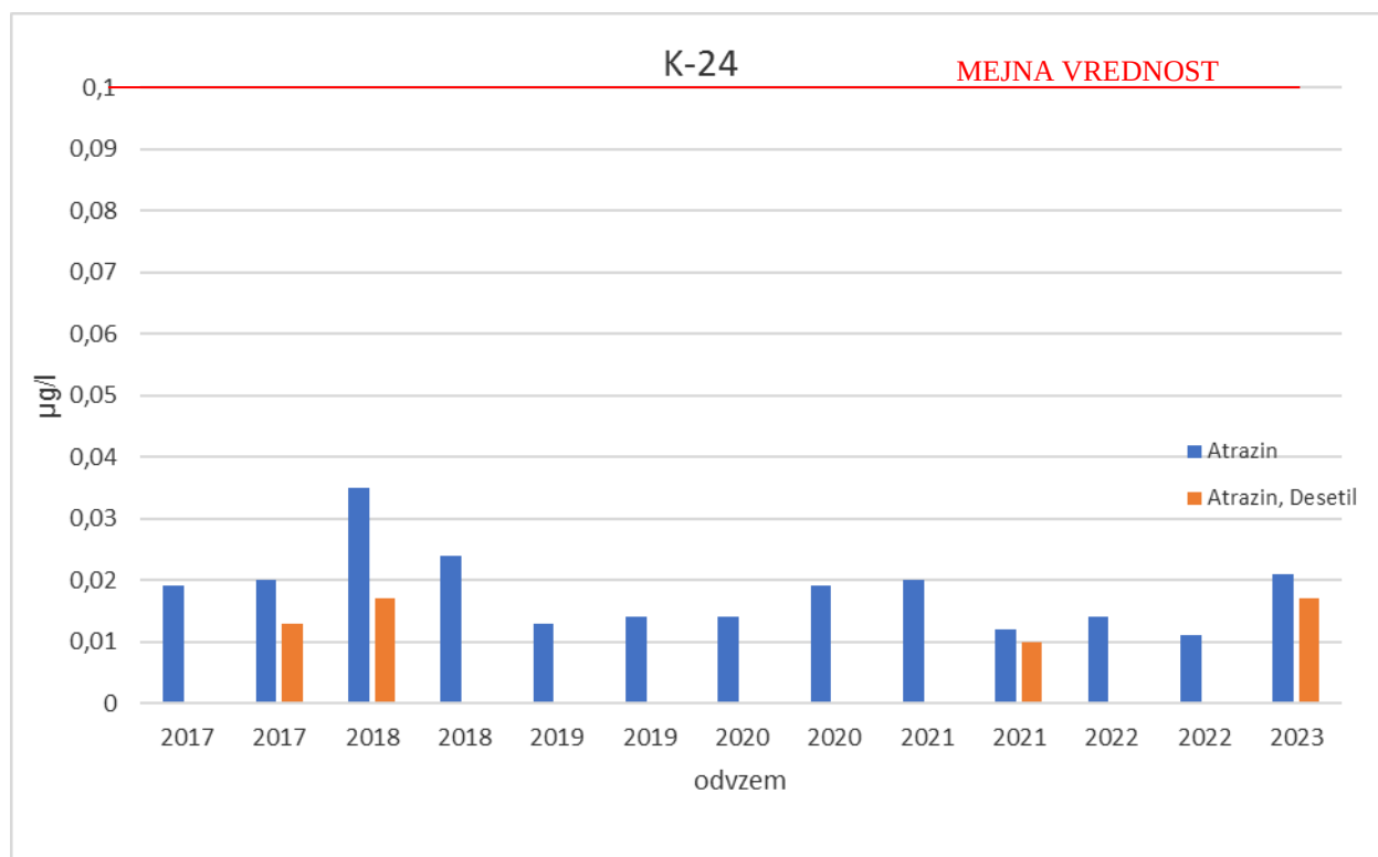
Slika 3-49: Prisotnost pesticidov atrazina in desetil-atrazina v letih 2017-2023 (µg/l) na merilnem mestu K-24
