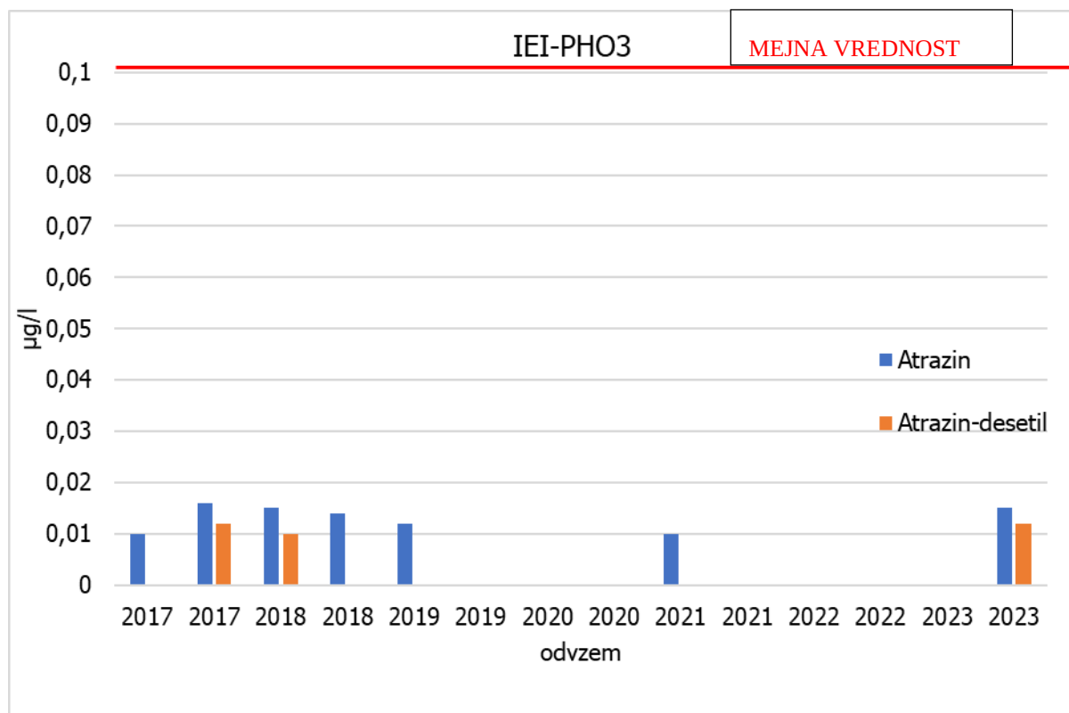
Slika 3-92: Vsebnost atrazina, atrazin-desetilain metabolita metolaklor ESA (µg/l) v podzemni vodi na opazovalni vrtini IEI-PHO3 v letih 2017-2023
