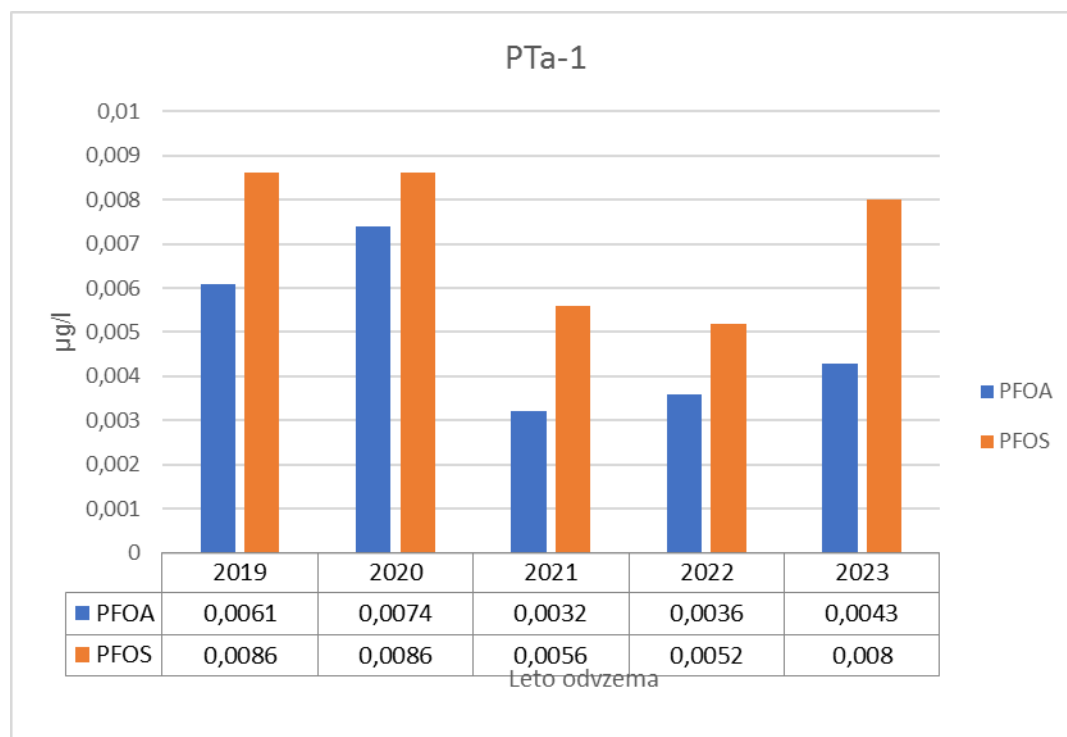
Slika 3-70: Izmerjene koncentracije PFOA in PFOS na odvzemnem mestu PTa-1 v letih 2019-2023
