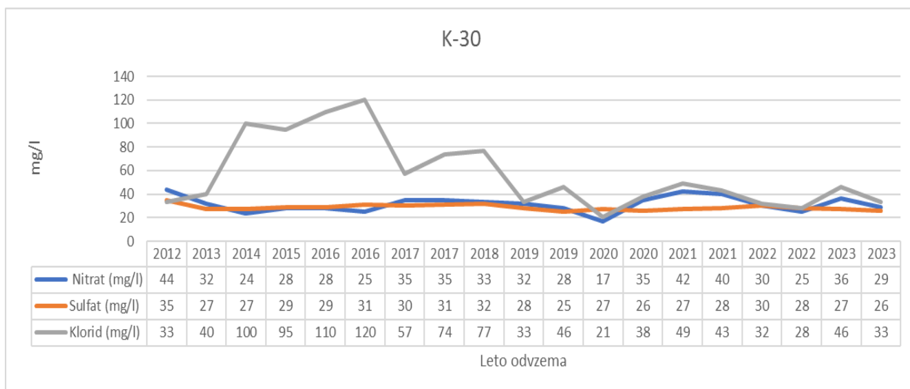
Slika 3-51: Vsebnost nitrata, sulfata in klorida (mg/l) v podzemni vodi namerilnem mestu K-30 v letih 2012-2023
