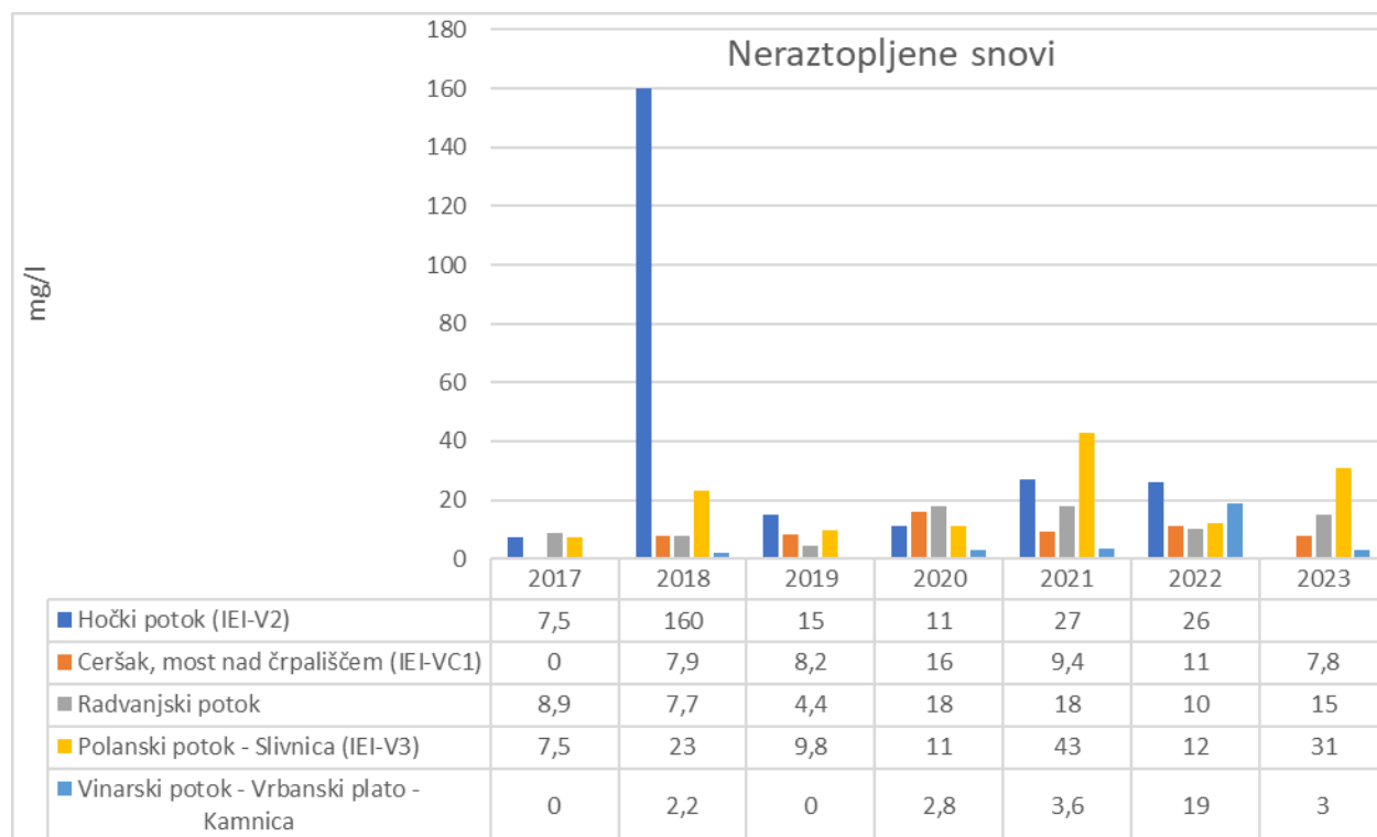
Slika 4-16: Prikaz obremenitev površinskih voda z neraztopljenimi snovmi v letih 2017-2023. Vrednosti 0 označujejo meritve, kjer je bila izmerjena vrednost pod mejo detekcije uporabljene metode
