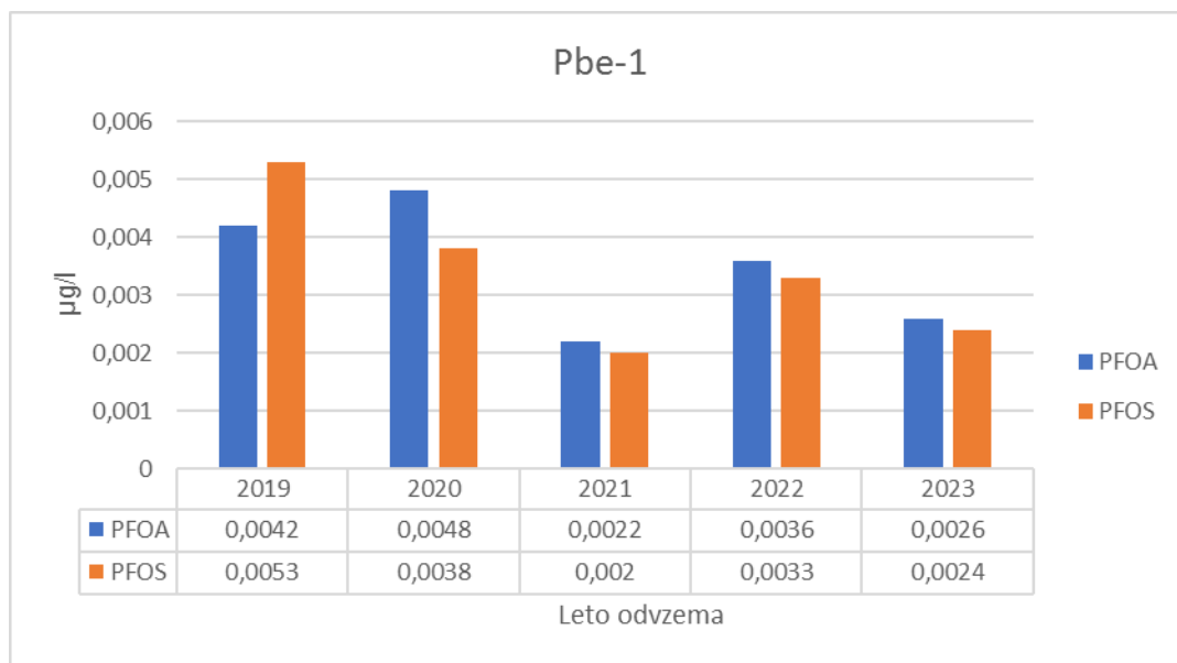
Slika 3-69: Izmerjene koncentracije PFOA in PFOS na odvzemnem mestu Pbe-1 v letih 2019-2023
