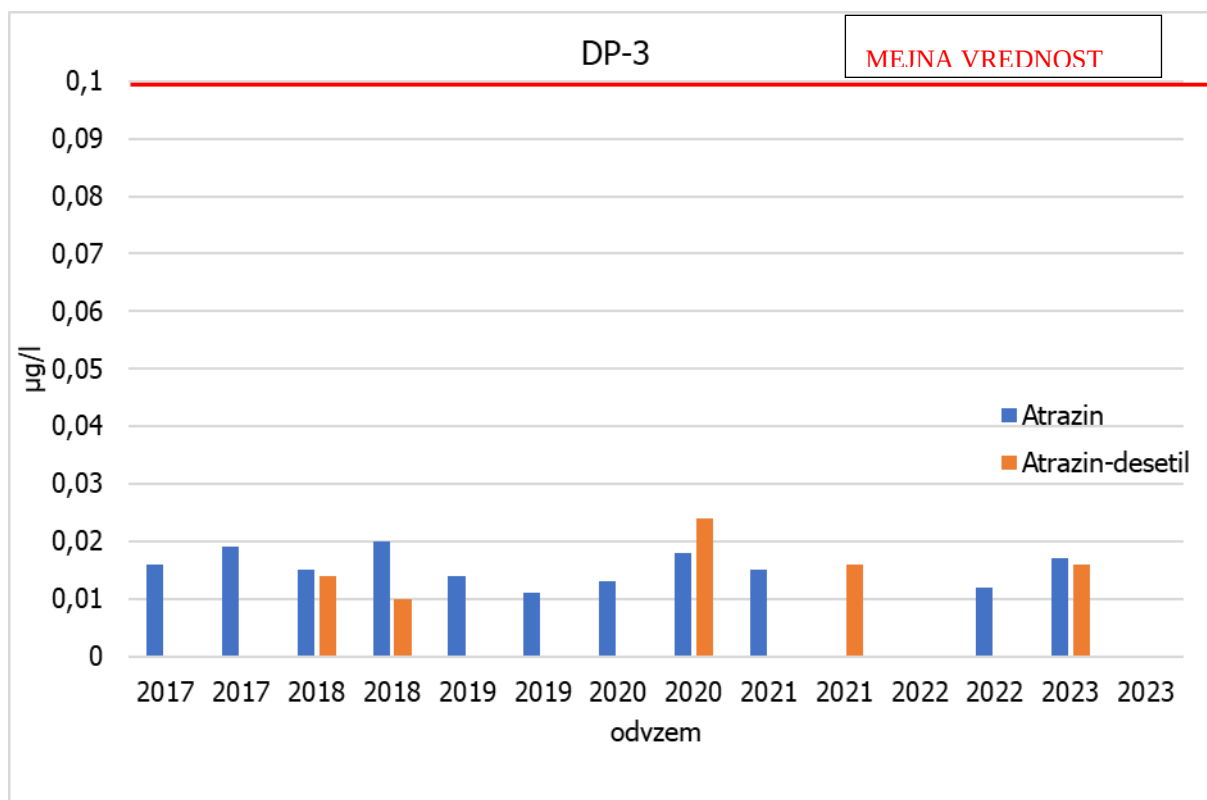
Slika 3-91: Vsebnosti atrazina in atrazin-desetila (µg/l) v podzemni vodi na opazovalni vrtini DP-3 v letih 2017-2023
