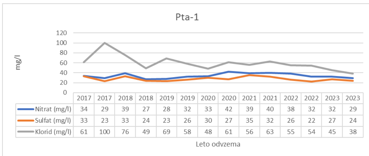
Slika 3-66: Nihanje vsebnosti nitrata in klorida (mg/l) na merilnem mestu Pta-1 v letih 2017-2023
