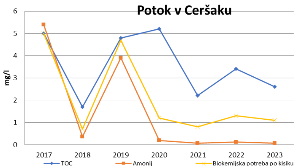
Slika 4-20: Prikaz nihanja osnovnih kemijskih parametrov na odvzemnem mestu Potok v Ceršaku v letih 2017-2023
