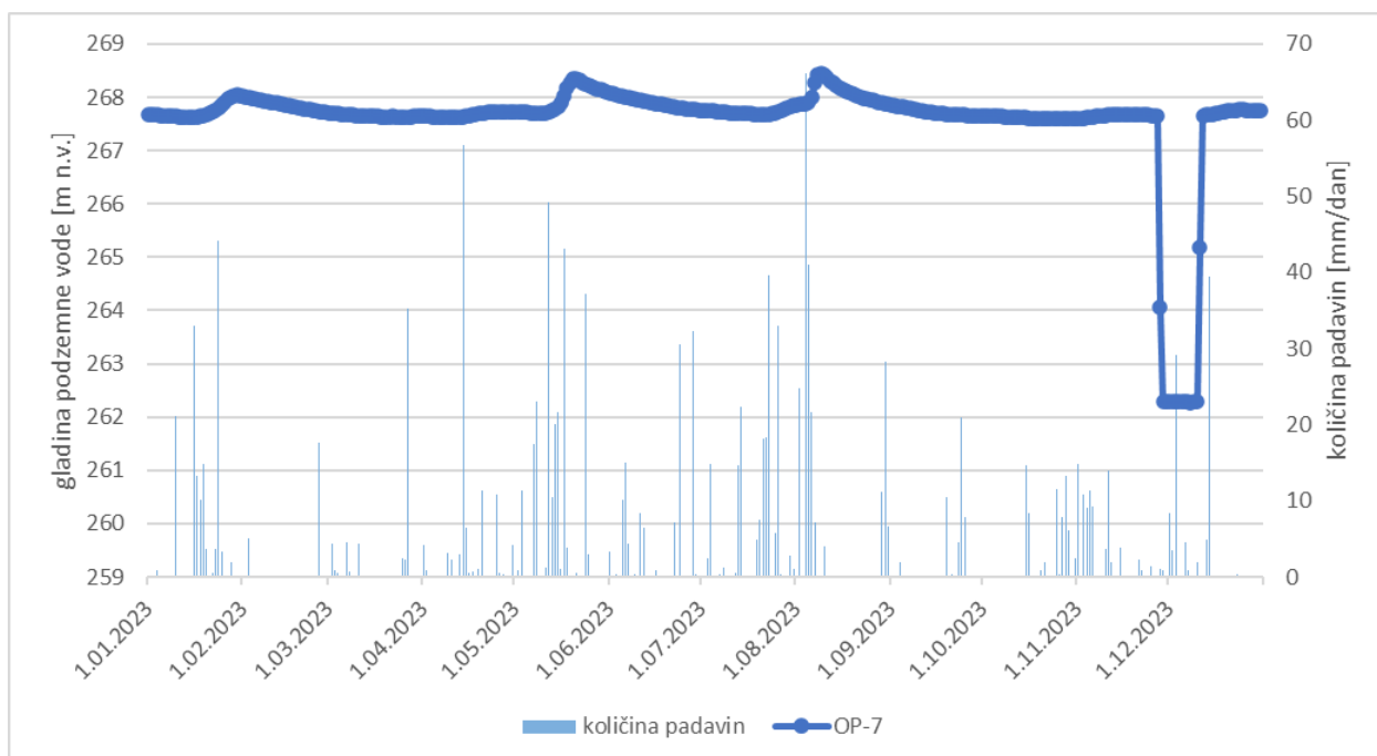
Slika 3-64: Grafični prikaz avtomatskih meritev gladin podzemne vode na merilnem mestu OP-7 ter količine padavin izmerjenih na meteorološki postaji Letališče Edvarda Rusjana v letu 2023
