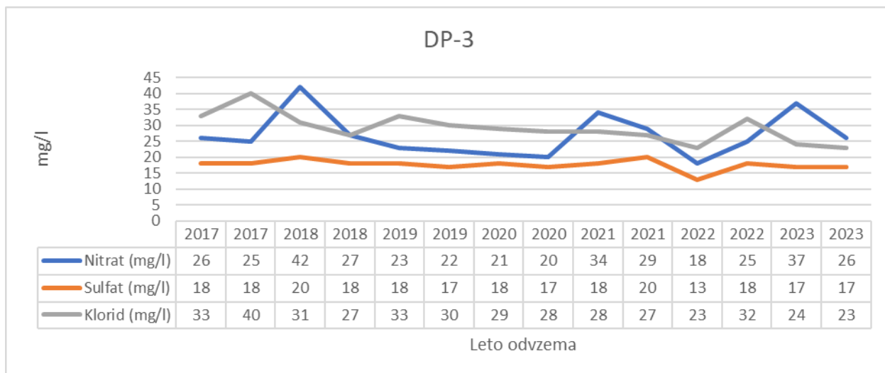
Slika 3-87: Vsebnost nitrata, sulfata in klorida (mg/l) v podzemni vodi na opazovalni vrtini DP-3 v letih 2017-2023
