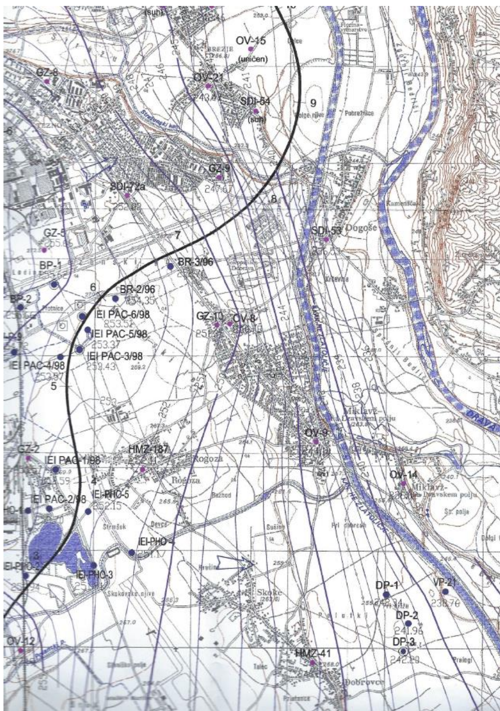
Slika 3-79: Ocenjen tok podzemne vode na območju črpališča Bohova in Dobrovce (vir: GeoZS)
