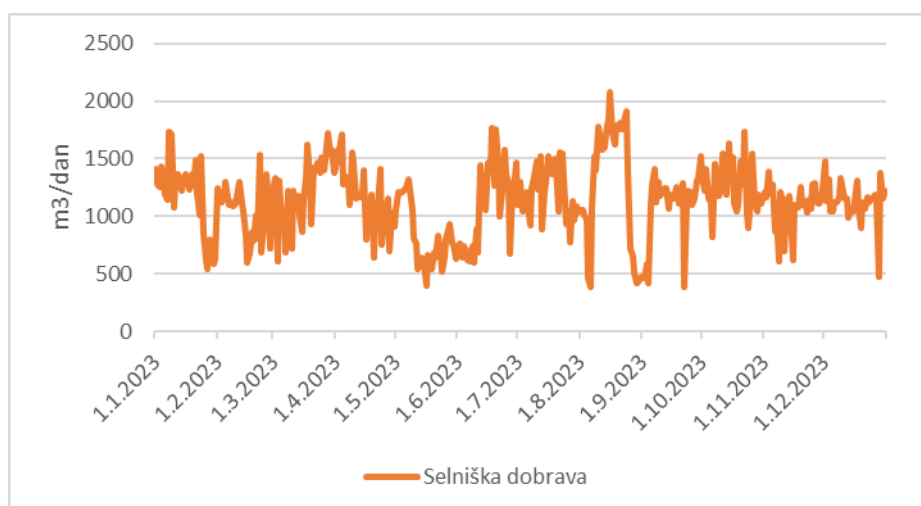
Slika 3-23: Grafični prikaz črpanih količin podzemne vode na območju črpališča Selniška dobrava
