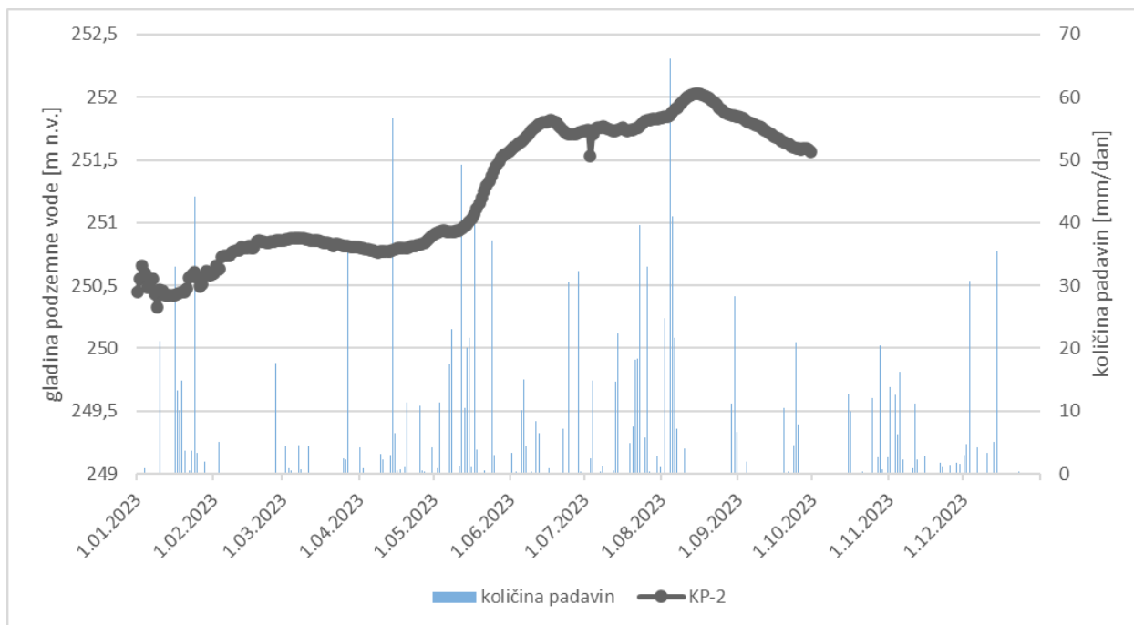
Slika 3-38: Grafični prikaz avtomatskih meritev gladin podzemne vode na merilnem mestu KP-2N ter količine padavin izmerjenih na meteorološki postaji Vrbanski plato v letu 2023
