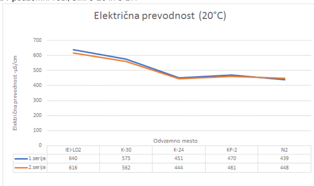
Slika 3-25: Prikaz električne prevodnosti ( \mu\text{S}/\text{cm} ) v letu 2022 na območju Vrbanskega platoja
