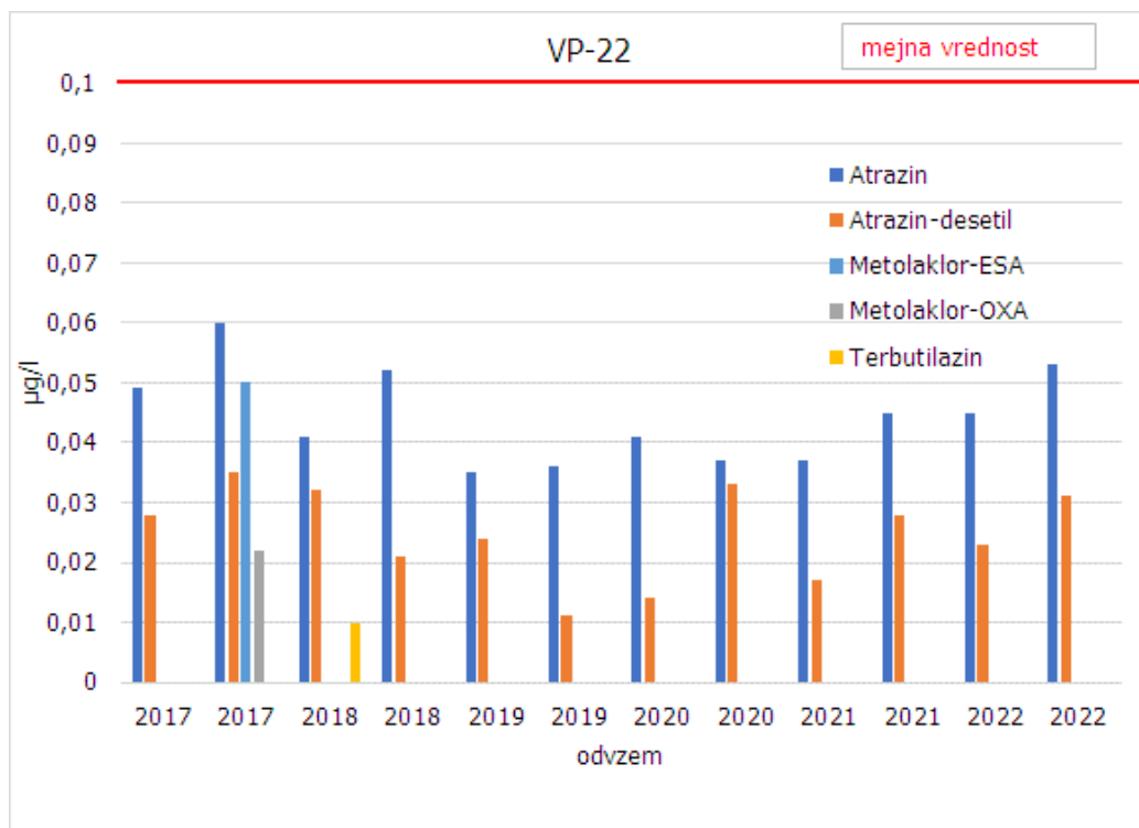
Slika 3-80: Vsebnost atrazina, atrazin-desetila, terbutilazina ter metabolita metolaklor OXA in metaloklor ESA (µg/l) v podzemni vodi na opazovalni vrtini VP-22 v letih 2017-2022
