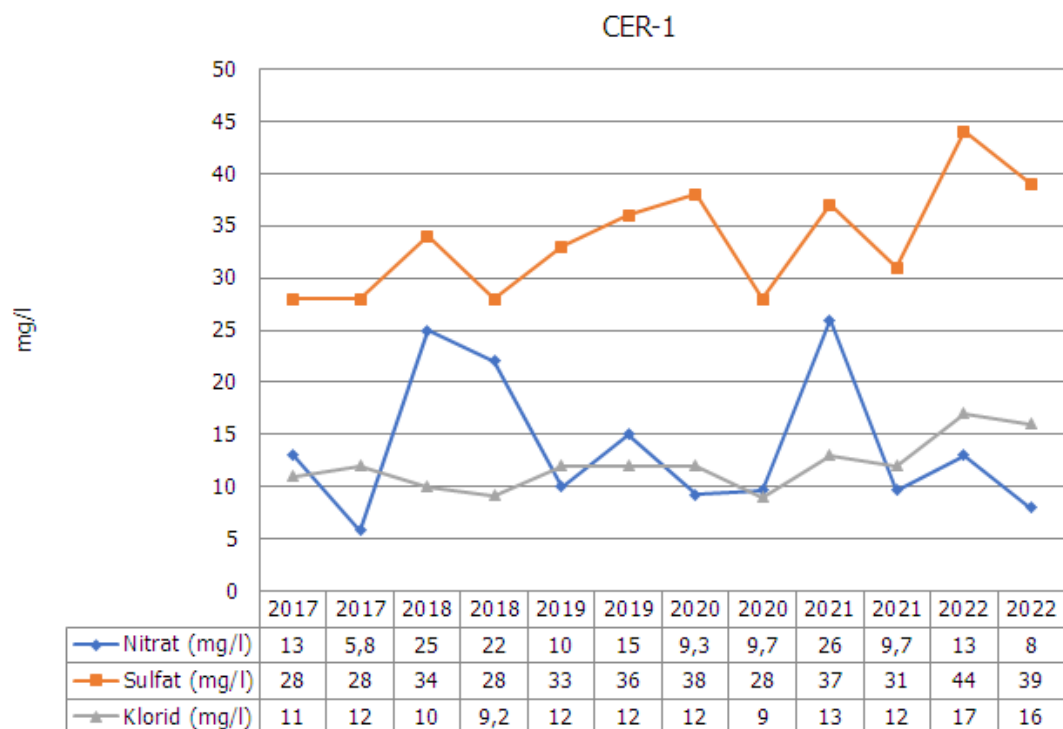
Slika 3-96: Vsebnost nitrata, sulfata in klorida (mg/l) v podzemni vodi na opazovalni vrtini CER-1 v letih 2017-2022
