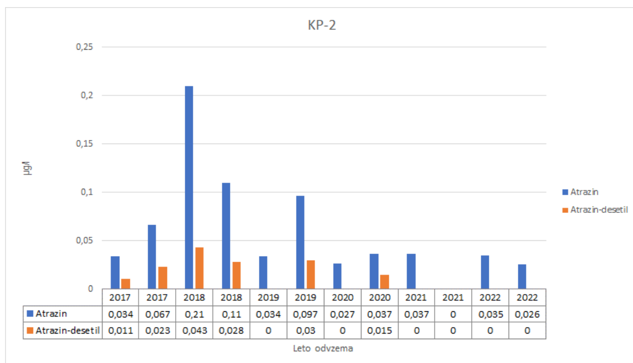
Slika 3-5: Gibanje vsebnosti atrazina in njegovega razgradnega produkta (µg/l) na odzemnem mestu KP-2 v letih 2017-2022
