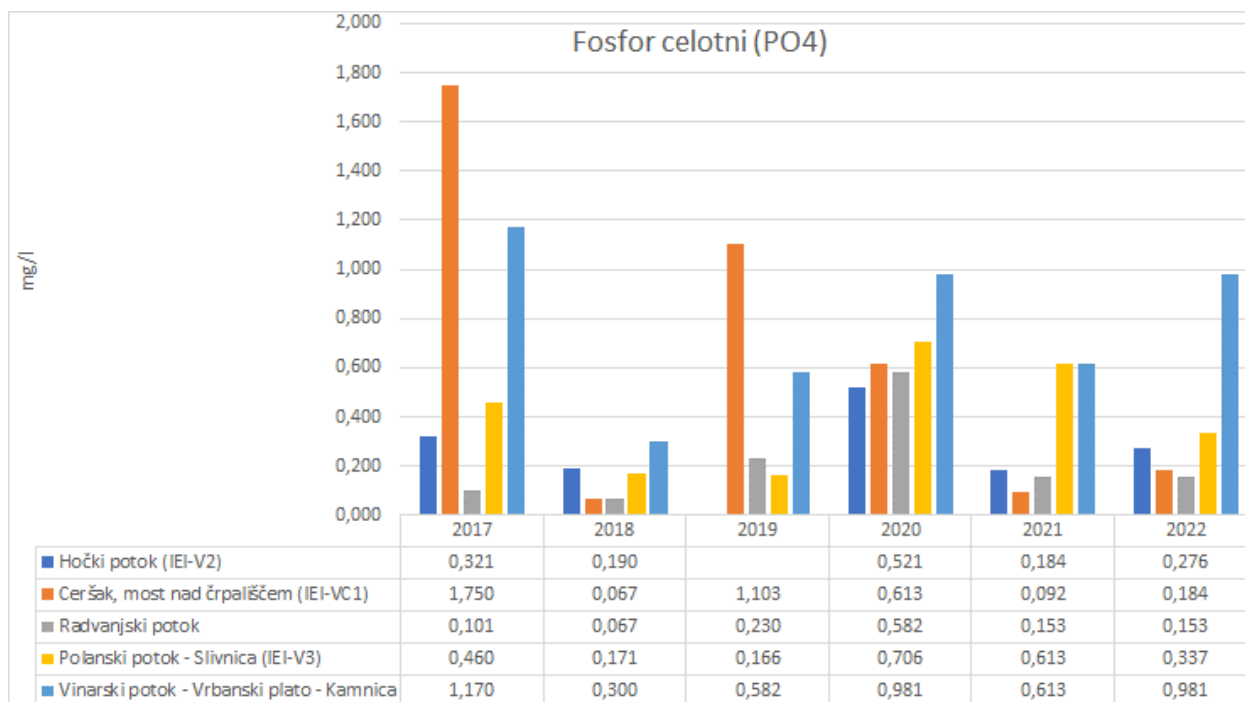
Slika 5-3: Prikaz obremenitev površinskih voda s skupnim fosforjem v letih 2017-2022
