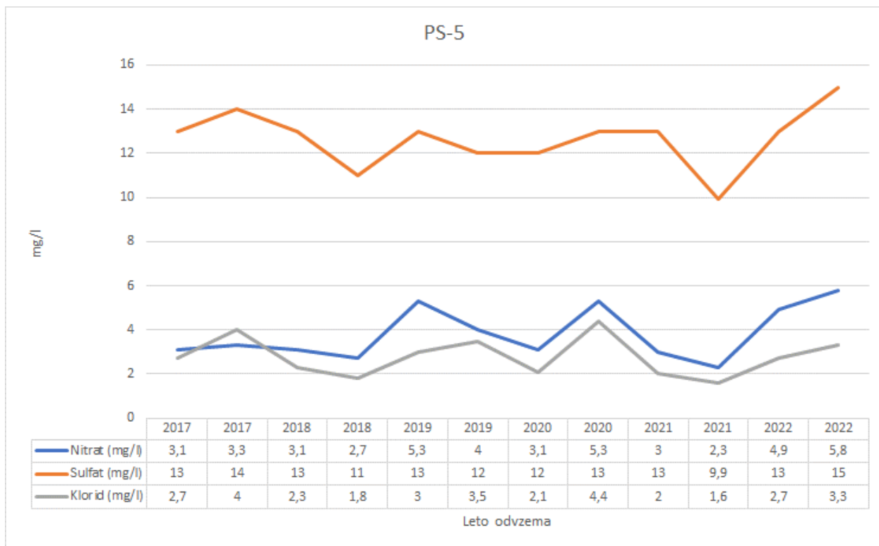
Slika 3-14: Vsebnost nitrata, sulfata in klorida (mg/l) v podzemni vodi v letih 2017-2022 na območju Selniške dobrove
