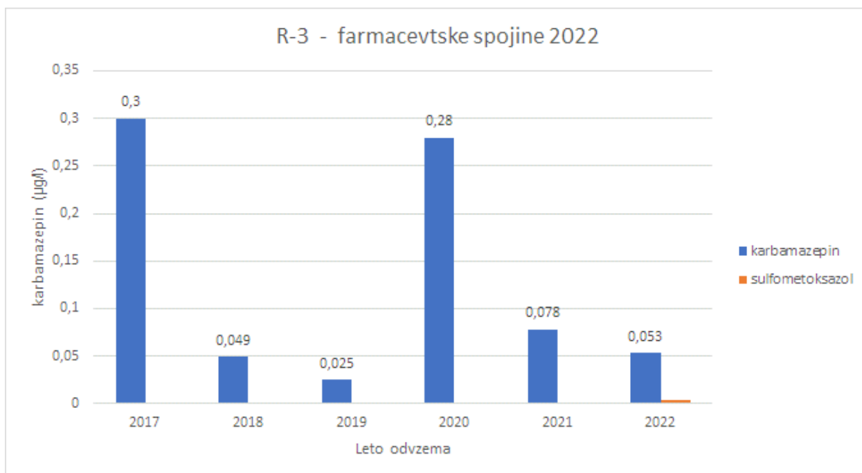
Slika 3-16: Vsebnosti karbamazepina in sulfometoksazola na odvzemnem mestu R-3 v letih 2017-2022
