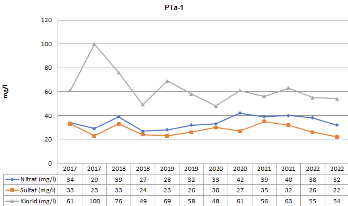
Slika 3-48: Nihanje vsebnosti nitrata in klorida (mg/l) na merilnem mestu PTa-1 v letih 2017-2022
