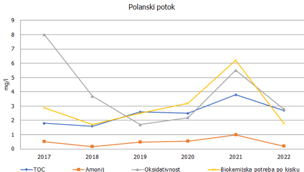
Slika 5-6: Prikaz nihanja osnovnih kemijskih parametrov na odvzemnem mestu Polanski potok v letih 2017-2022
