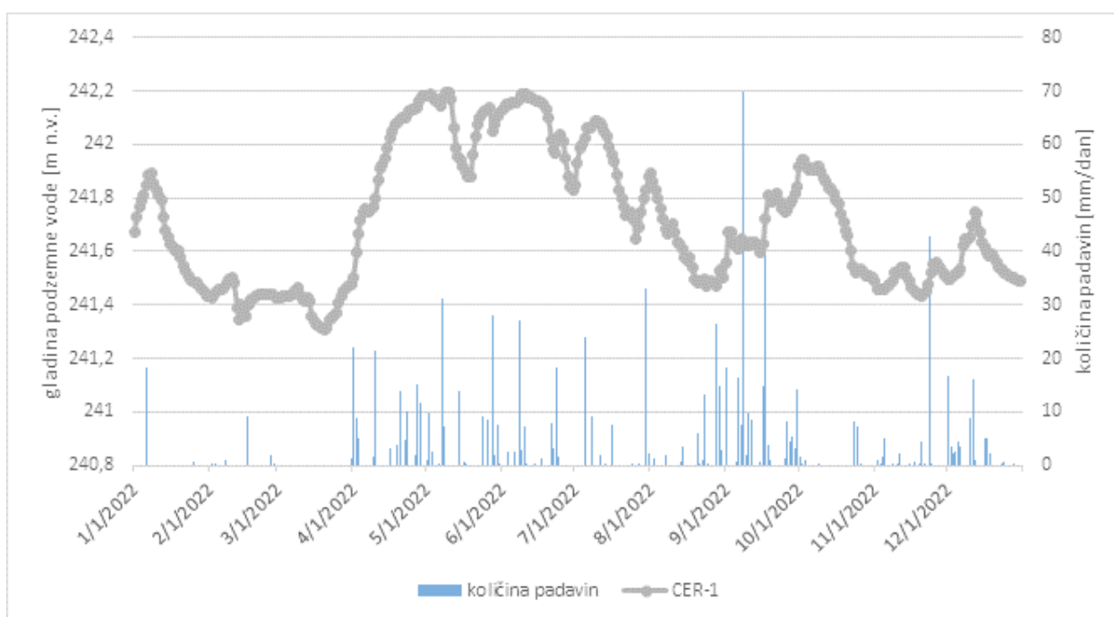
Slika 3-91: Grafični prikaz avtomatskih meritev gladin podzemne vode na merilnem mestu CER-1 (Ceršak) ter količina padavin izmerjenih na meteorološki postaji Vrbanski plato v letu 2022
