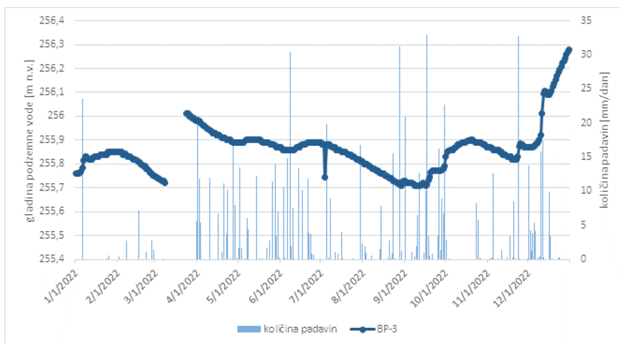
Slika 3-87: Grafični prikaz avtomatskih meritev gladin podzemne vode na merilnem mestu BP-3 (Bohova) ter količine padavin izmerjenih na meteorološki postaji letališče Vrbanjski plato v letu 2022
