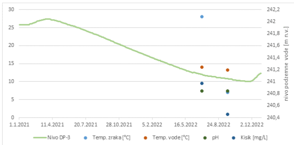
Slika 3-70: Grafični prikaz avtomatskih meritev nivojev podzemne vode na merilnem mestu DP3 ter osnovnih parametrov podzemne vode na merilnem mestu VP-22 (temperatura vode, temperatura zraka, pH, kisik)
