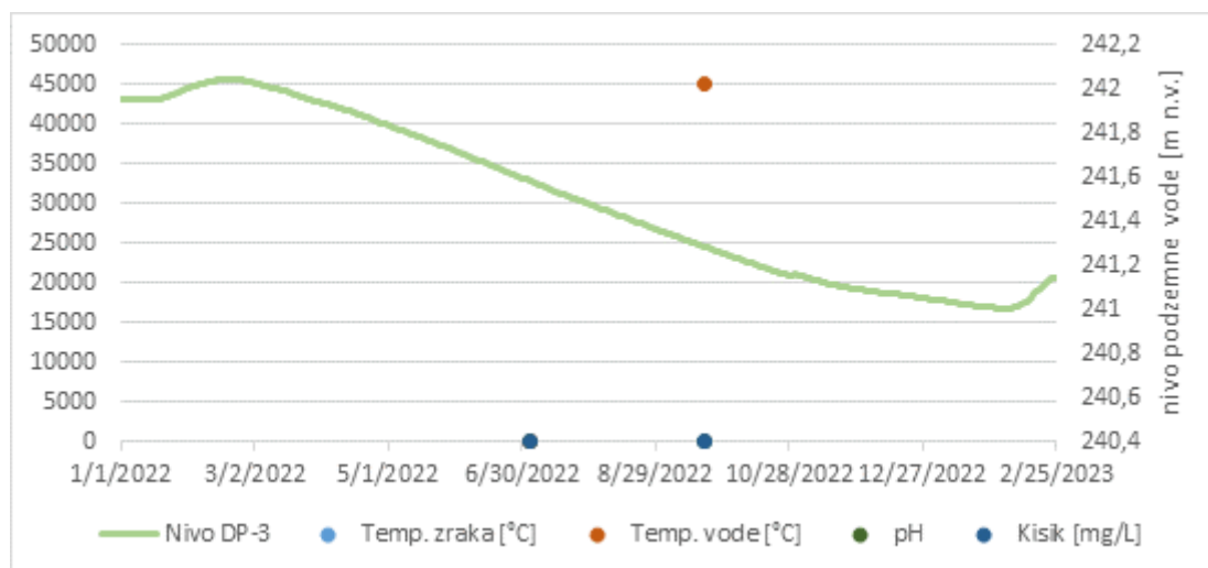
Slika 3-68: Grafični prikaz avtomatskih meritev nivojev podzemne vode na merilnem mestu DP3 ter osnovnih parametrov podzemne vode (temperatura vode, temperatura zraka, pH, kisik)
