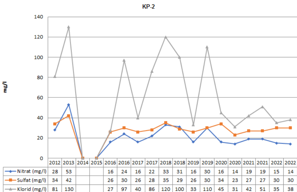
Slika 3-41: Vsebnost nitrata, sulfata in klorida (mg/l) v podzemni vodi na piezometru KP-2 v letih 2012-2022
