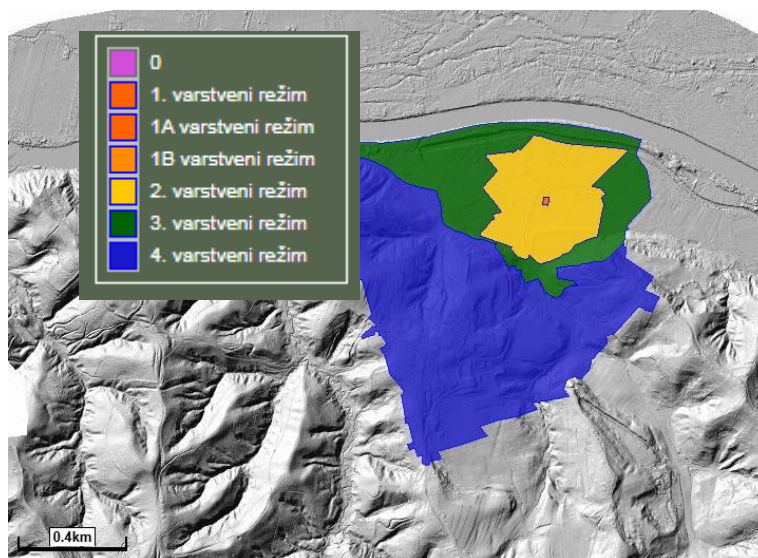
Slika 3-89: Črpališče Ceršak in vodovarstvena območja (vir: ARSO, Atlas okolja)
