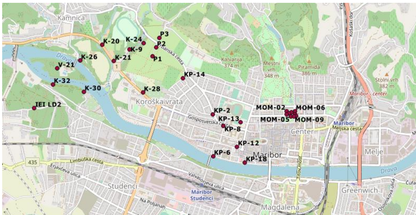
Slika 3-22: Prikaz merilnih mest podzemne vode na območju Vrbanskega platoja (vir podlage: OpenStreetMap):
