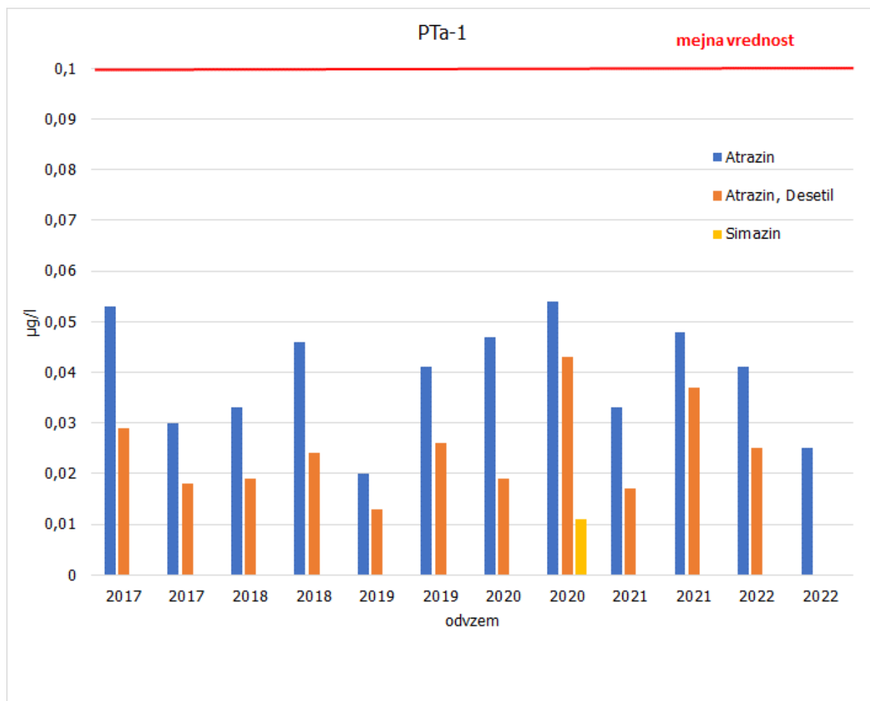
Slika 3-55: Vsebnost pesticidov atrazina, desetil-atrazina in simazina (µg/l) v podzemni vodi na merilnem mestu PTa-1 v letih 2017-2022
