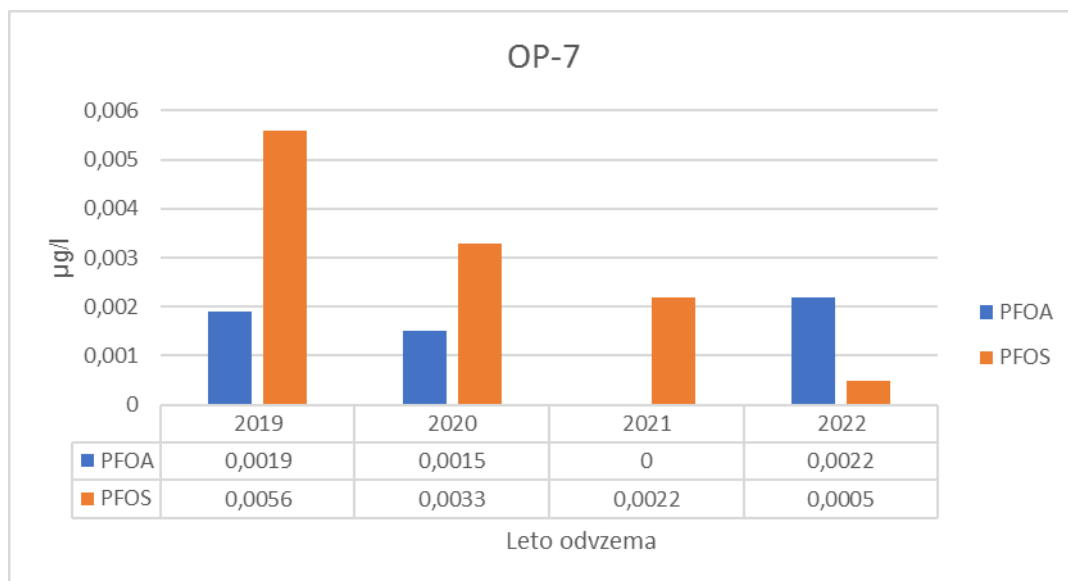
Slika 3-50: Izmerjene koncentracije PFOA in PFOS na odvzemnem mestu OP-7 v letih 2019-2022
