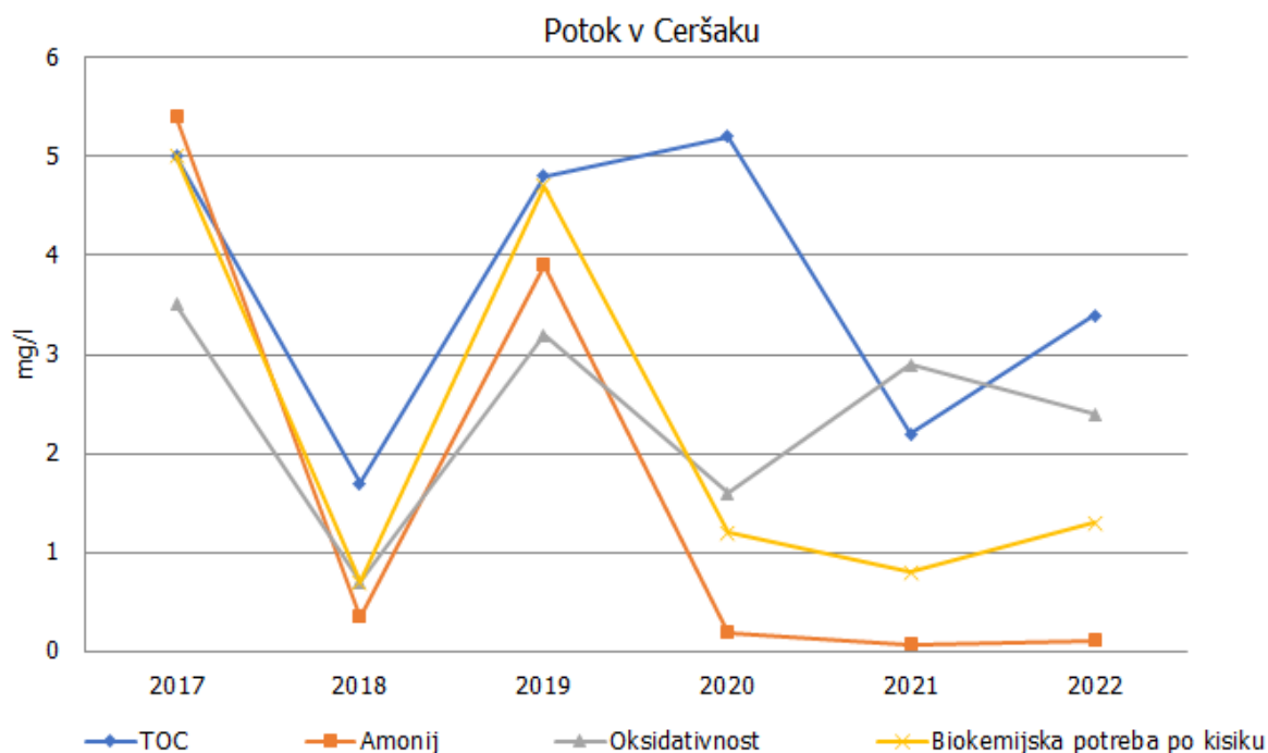
Slika 5-5: Prikaz nihanja osnovnih kemijskih parametrov na odvzemnem mestu Potok v Ceršaku v letih 2017-2022
