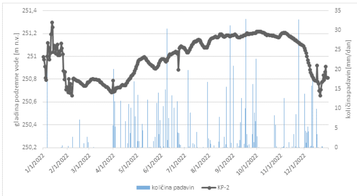
Slika 3-24: Grafični prikaz avtomatskih meritev gladin podzemne vode na merilnem mestu KP-2 ter količine padavin izmerjenih na meteorološki postaji Vrbanski plato v letu 2022
