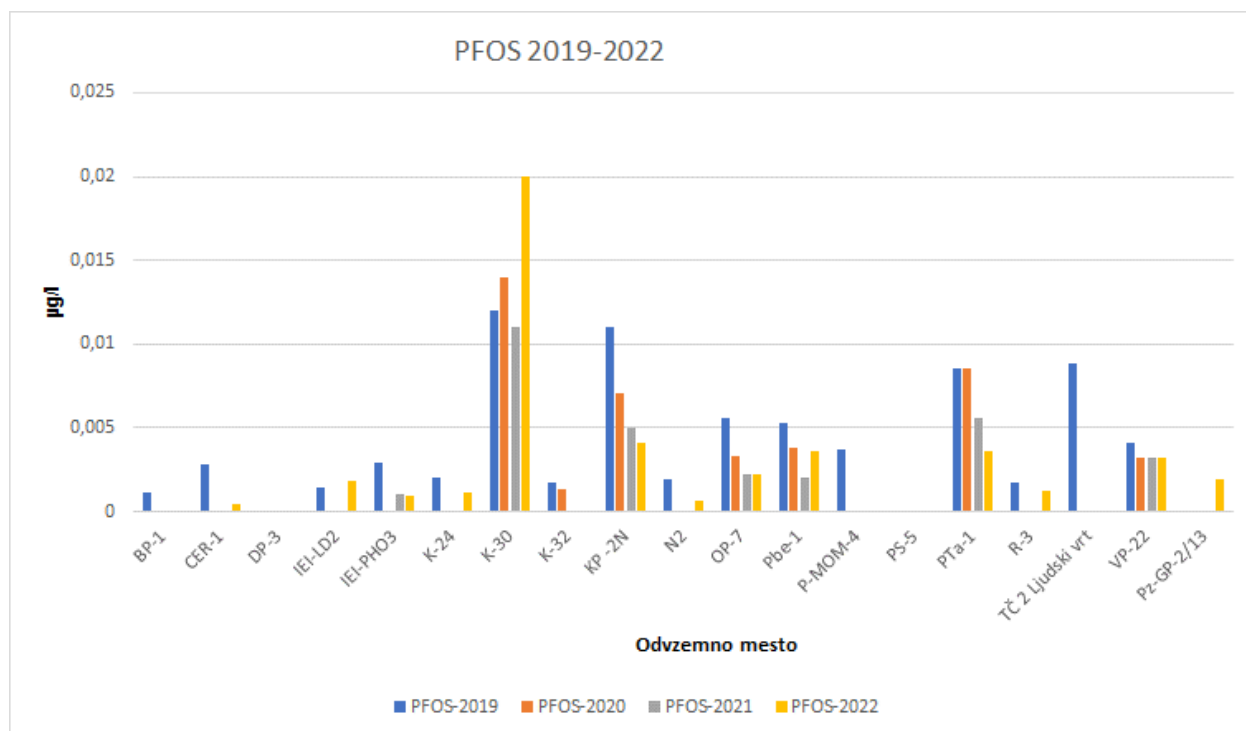
Slika 3-8: Gibanje vrednosti PFOS (µg/l) v letih 2019-2022
