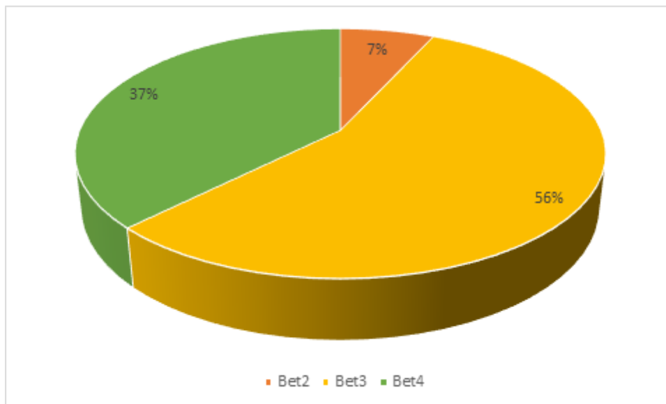
Slika 3-60: Grafični prikaz deleža črpanih količin iz posameznega vodnjaka v letu 2022 na območju črpališča Betnava
