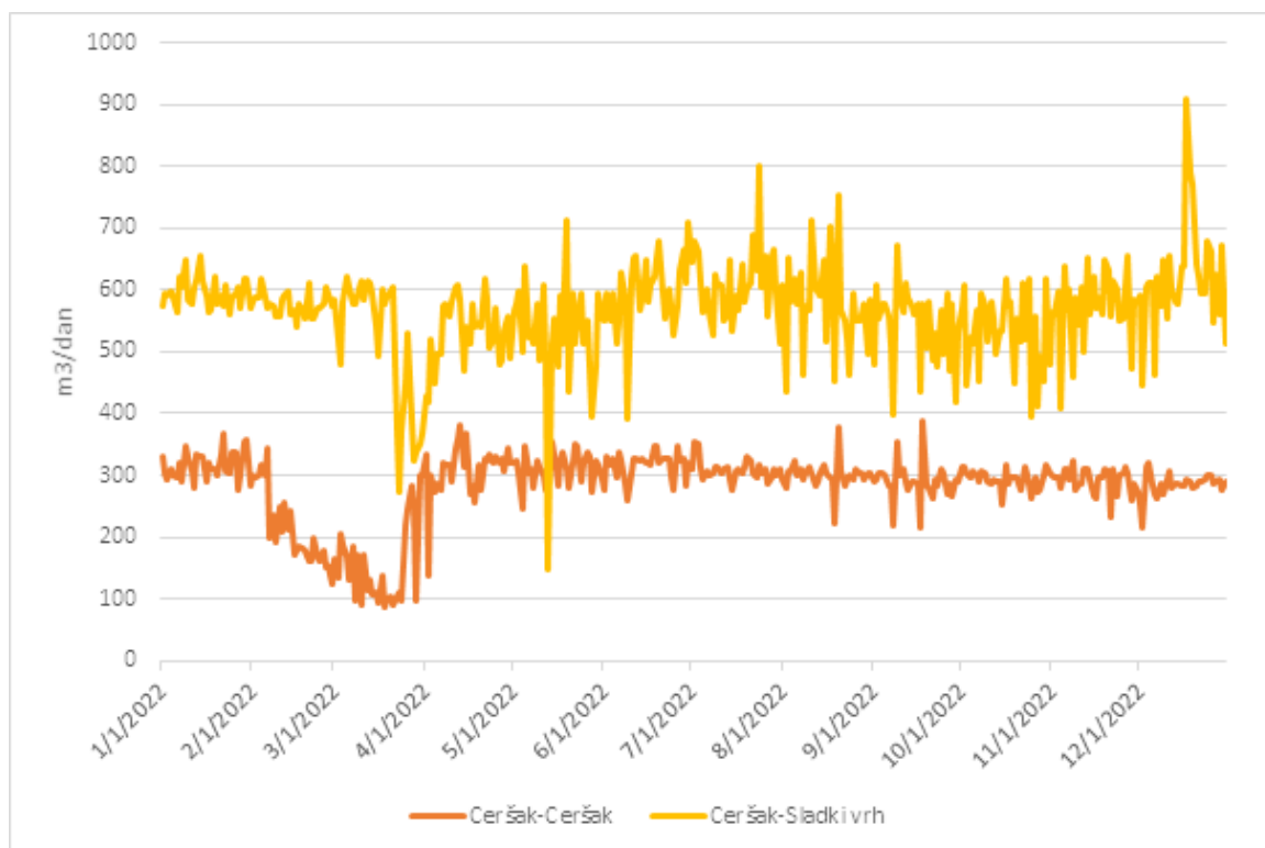
Slika 3-93: Grafični prikaz črpanih količin na območju črpališča Ceršak
