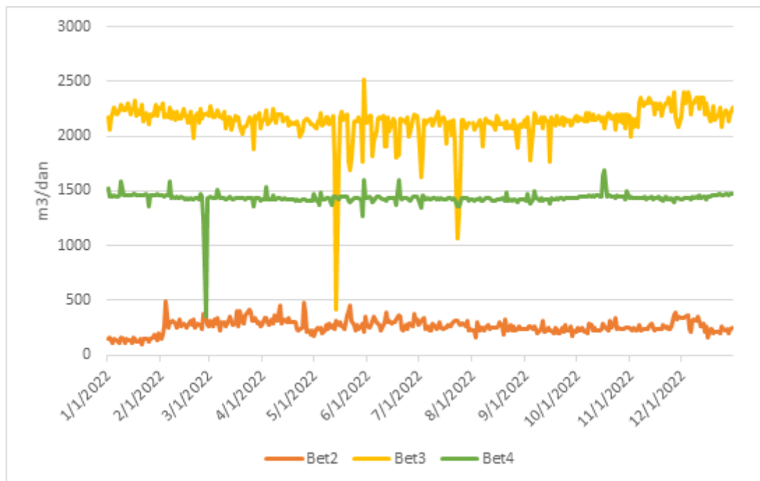
Slika 3-59: Grafični prikaz črpanih količin podzemne vode na območju črpališča Betnava v letu 2022
