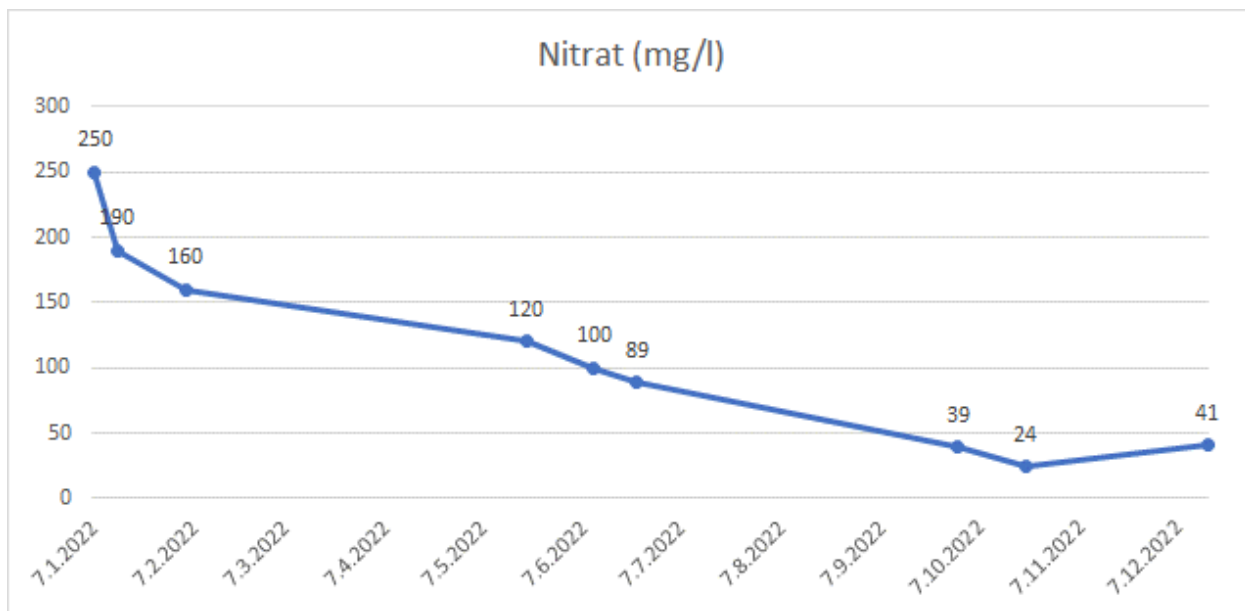
Slika 4-3: izmerjene vsebnosti nitrata (mg/l) v vzorcih odvzetih na lizimeterski postaji Tezno v letu 2022
