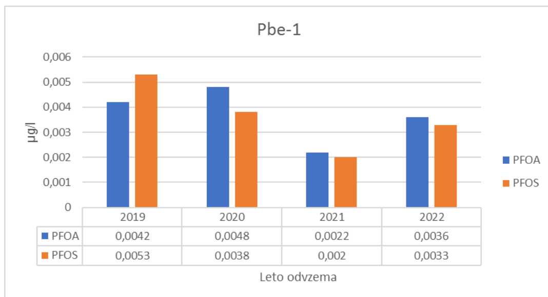
Slika 3-51: Izmerjene koncentracije PFOA in PFOS na odvzemnem mestu Pbe-1 v letih 2019-2022
