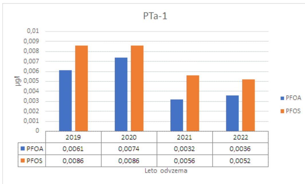
Slika 3-52: Izmerjene koncentracije PFOA in PFOS na odvzemnem mestu PTa-1 v letih 2019-2022
