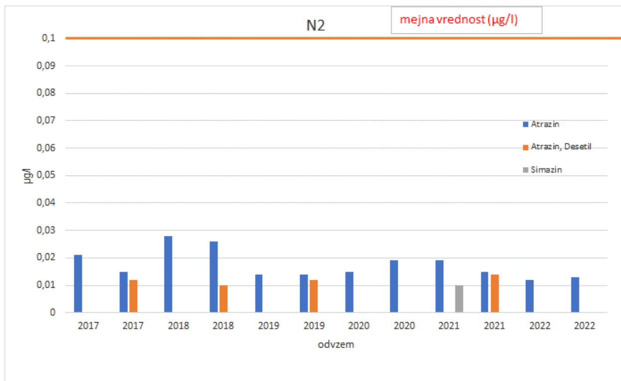
Slika 3-45: Vsebnost pesticidov (µg/l) v podzemni vodi na merilnem mestu N-2 v letih 2017-2022
