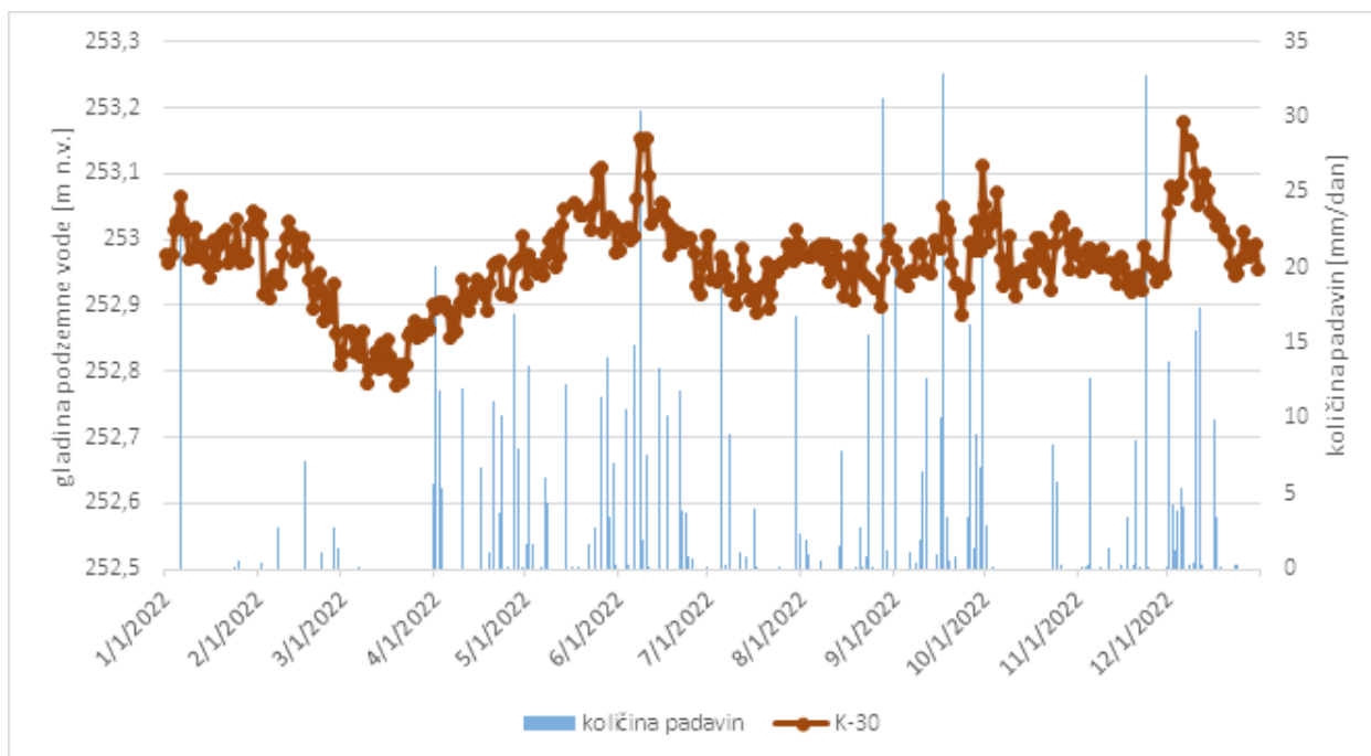
Slika 3-23: Grafični prikaz avtomatskih meritev gladin podzemne vode na merilnem mestu K-30 ter količine padavin izmerjenih na meteorološki postaji Vrbanski plato v letu 2022
