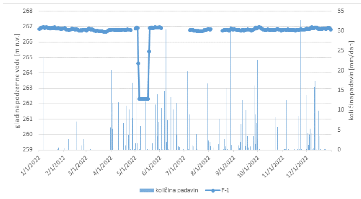
Slika 3-13: Grafični prikaz avtomatskih meritev gladin podzemne vode na merilnem mestu F-1 in količina padavin izmerjenih na meteorološki postaji Vrbanski plato v letu 2022
