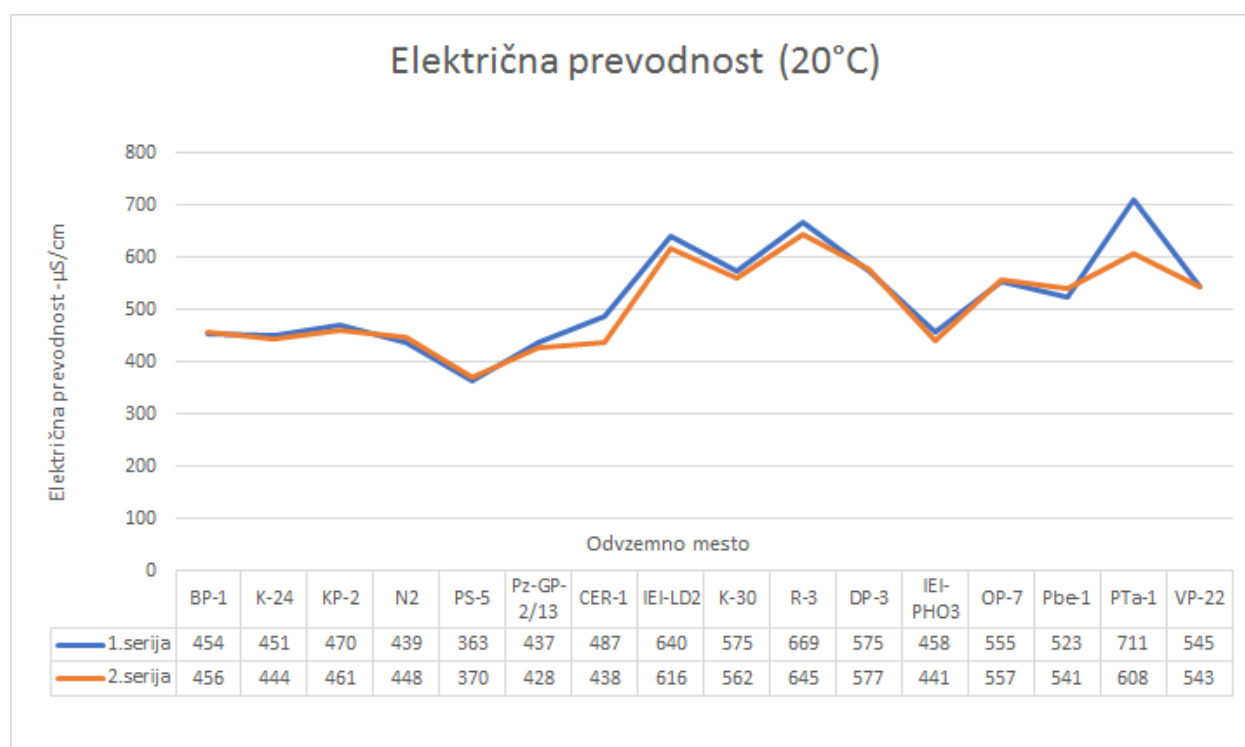
Slika 3-1: Izmerjene vrednosti električne prevodnosti podzemne vode v letu 2022
