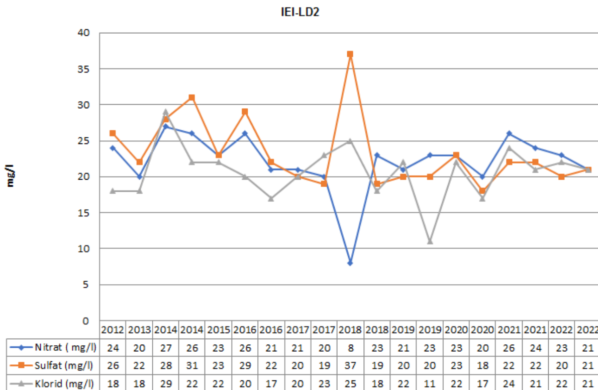
Slika 3-38: Vsebnost nitrata, sulfata in klorida (mg/l) v podzemni vodi na merilnem mestu IEI-LD2 v letih 2012-2022
