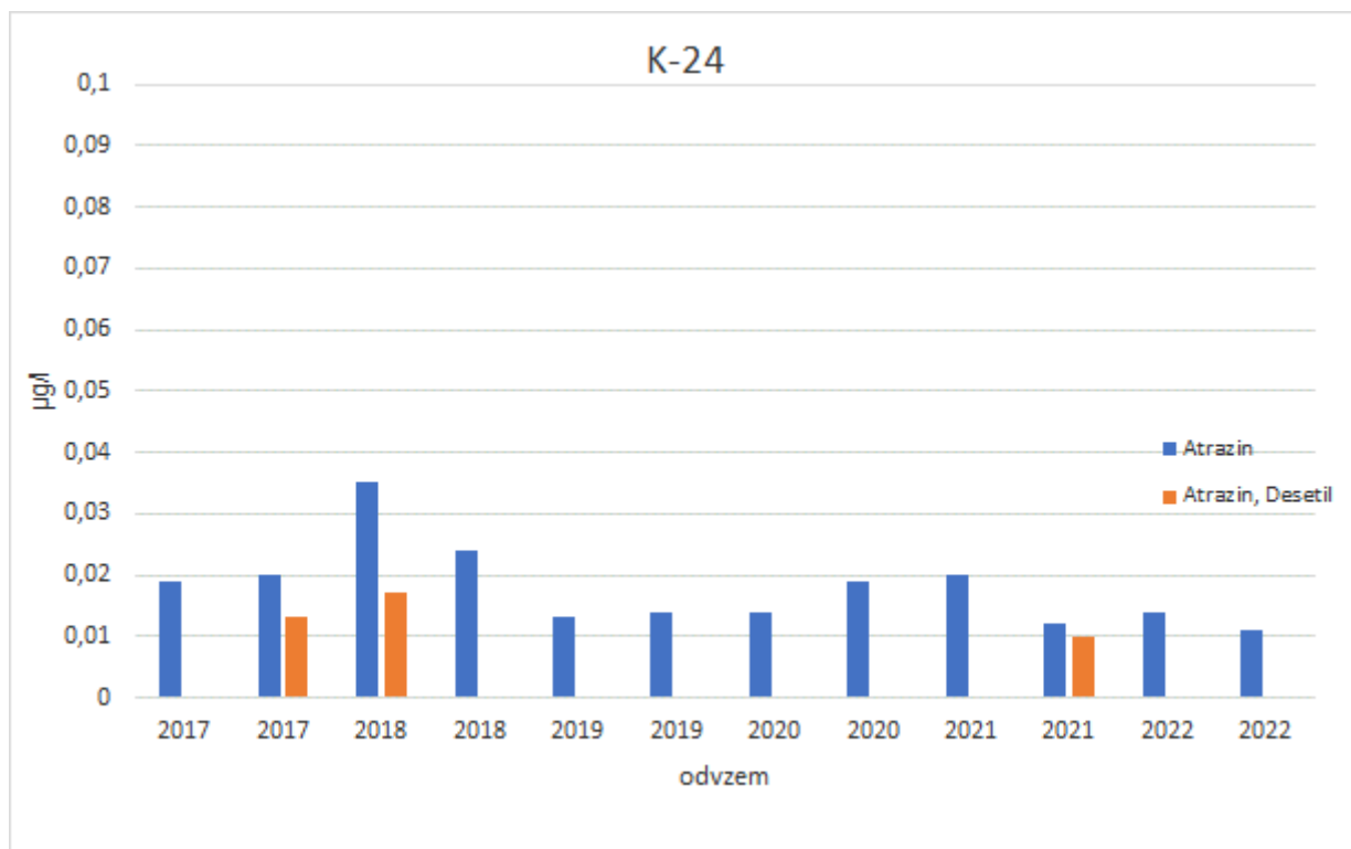
Slika 3-33: Prisotnost pesticidov atrazina in desetil-atrazina v letih 2017-2022 (µg/l) na merilnem mestu K-24
