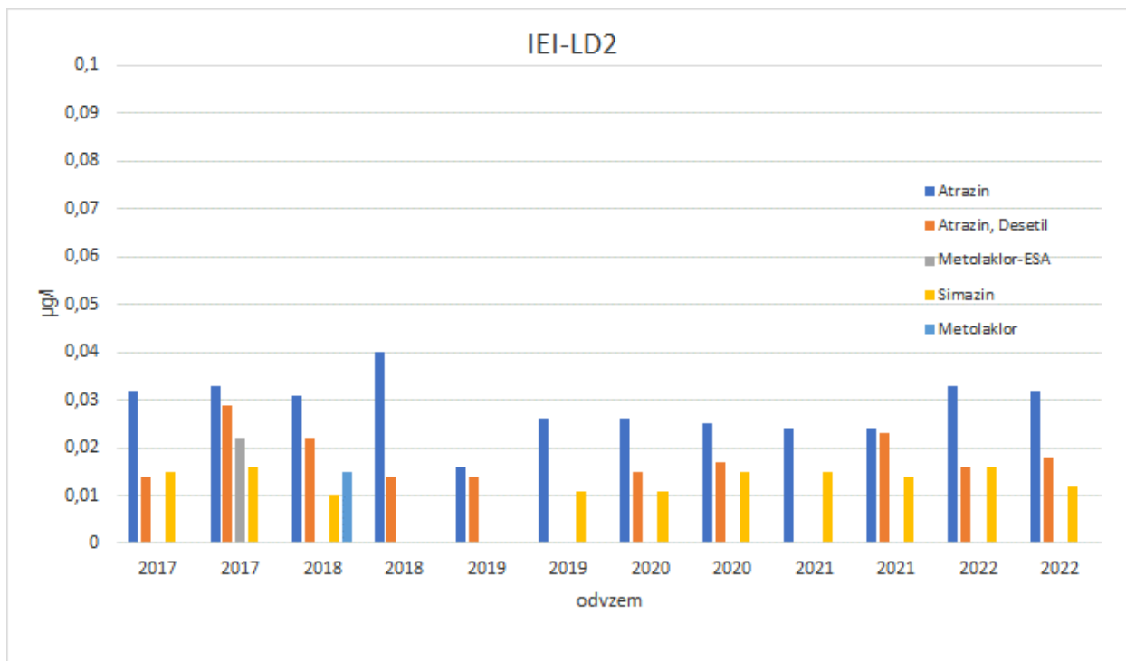
Slika 3-39: Vsebnost pesticidov (µg/l) v podzemni vodi na merilnem mestu IEI-LD2 v letih 2017-2022
