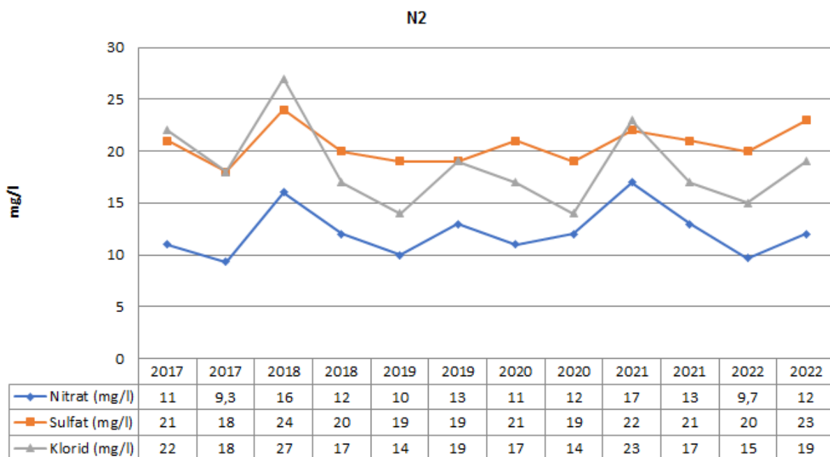
Slika 3-44: Vsebnost nitrata, sulfata in klorida (mg/l) v podzemni vodi na merilnem mestu N-2 v letih 2017-2022
