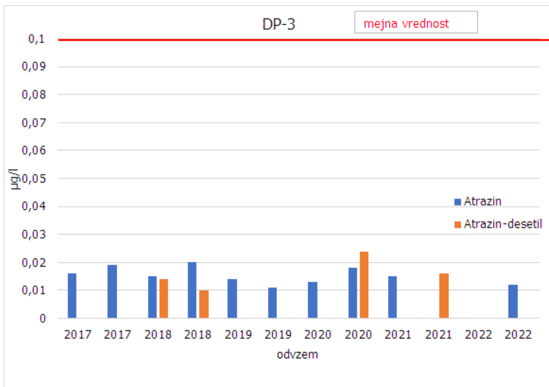
Slika 3-78: Vsebnosti atrazina in atrazin-desetila (µg/l) v podzemni vodi na opazovalni vrtini DP-3 v letih 2017-2022
