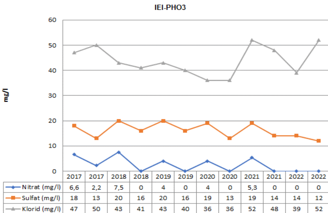
Slika 3-73: Vsebnost nitrata, sulfata in klorida (mg/l) v podzemni vodi na opazovalni vrtini IEI-PHO3 v letih 2017-2022
