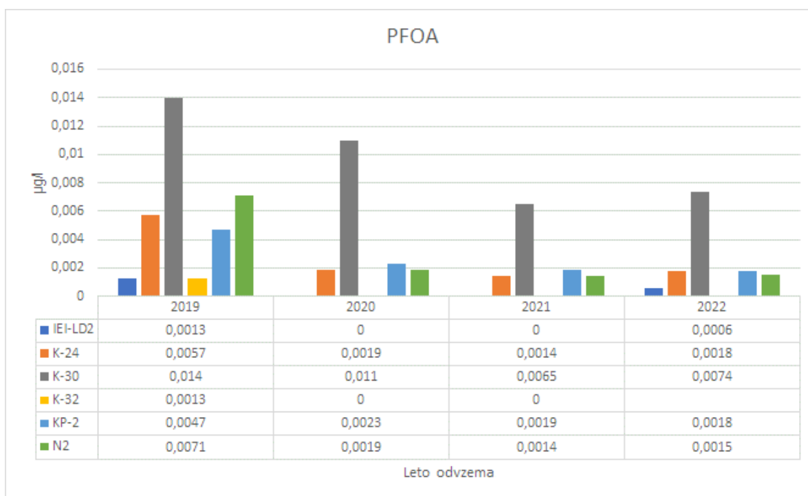
Slika 3-30: Prisotnost PFOA (µg/l) v letih 2019-2022
