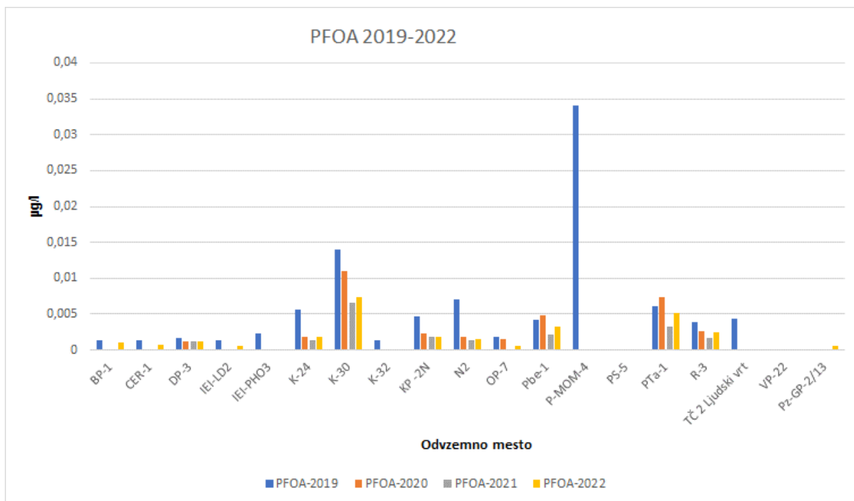
Slika 3-7: Gibanje vrednosti PFOA (µg/l) v letih 2019-2022
