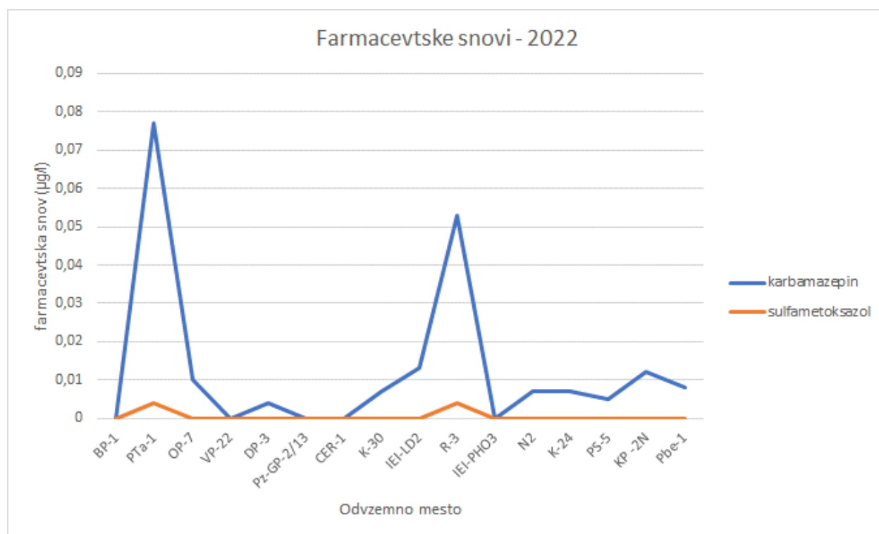
Slika 3-4: Ugotovljene prisotnosti farmacevtskih spojin v letu 2022
