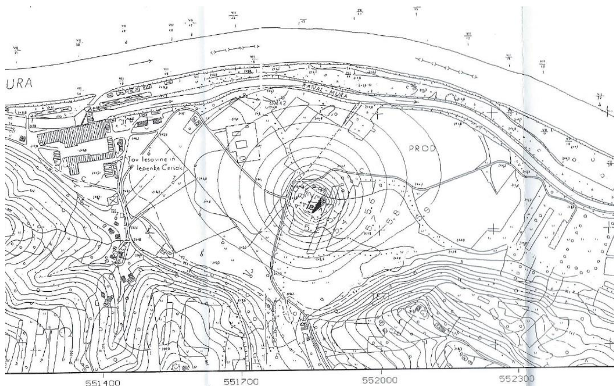
Slika 3-90: Ocenjene hidroizohipse na območju črpališča v Ceršaku
