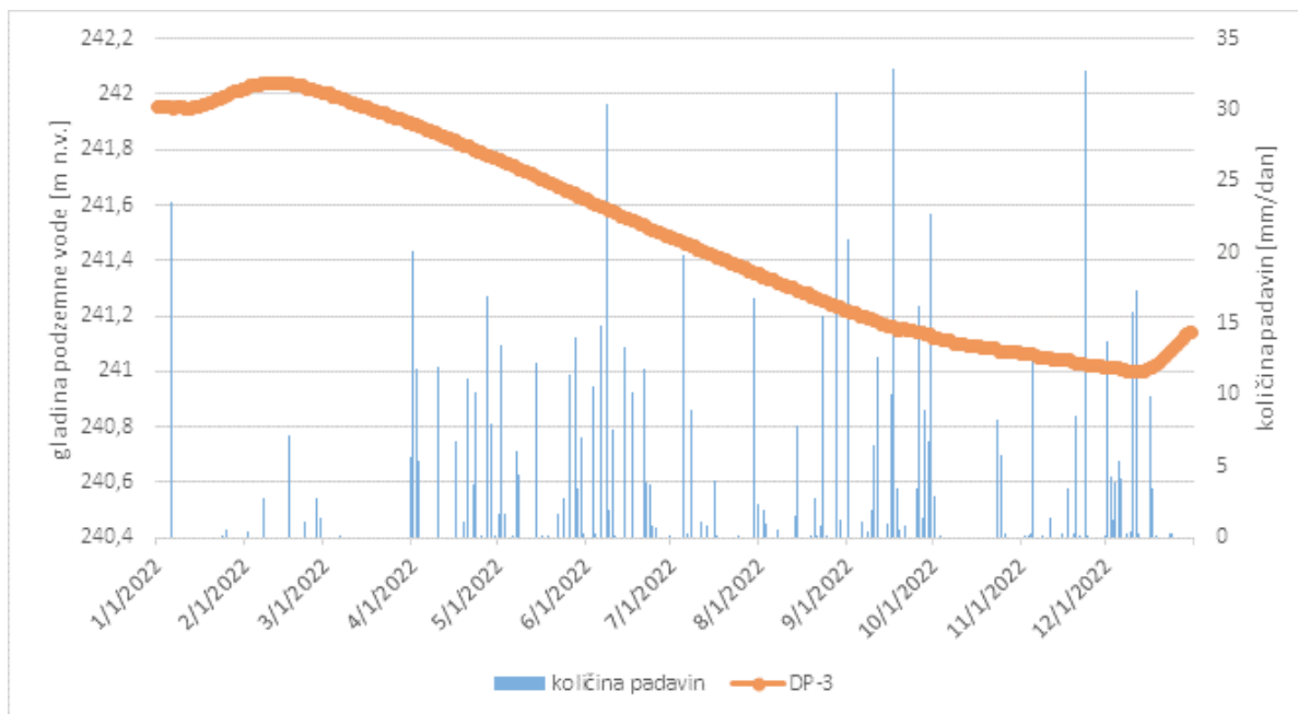
Slika 3-88: Grafični prikaz avtomatskih meritev gladin podzemne vode na merilnem mestu DP-3 (Dobrovce) ter količine padavin izmerjenih na meteorološki postaji Vrbanski plato v letu 2022
