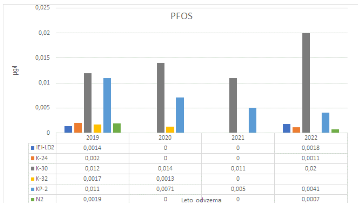
Slika 3-31: Prisotnost PFOS (µg/l) v letih 2019-2022
