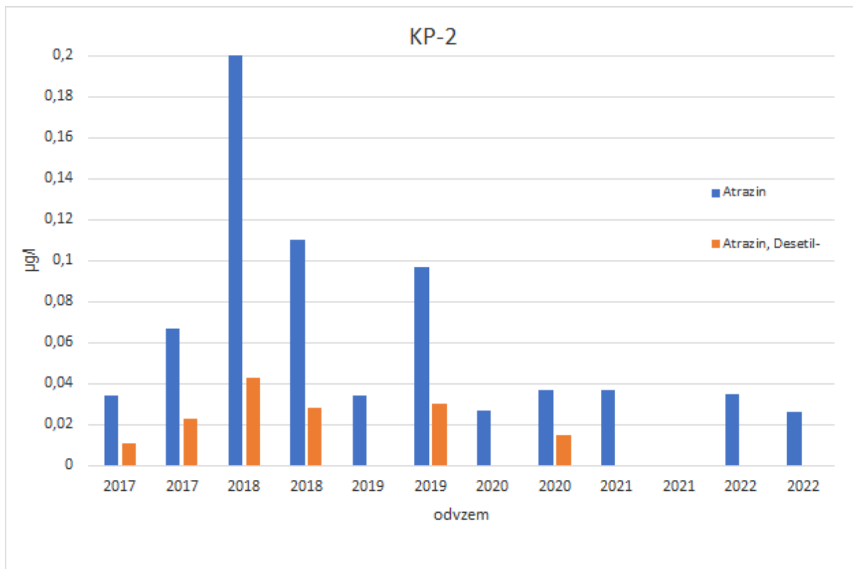
Slika 3-42: Vsebnost pesticidov ( \mu\text{g/l} ) v podzemni vodi na merilnem mestu KP-2 v letih 2017-2022 Lokacija merilnega mesta KP-2 je razvidna iz slike 3-43.
