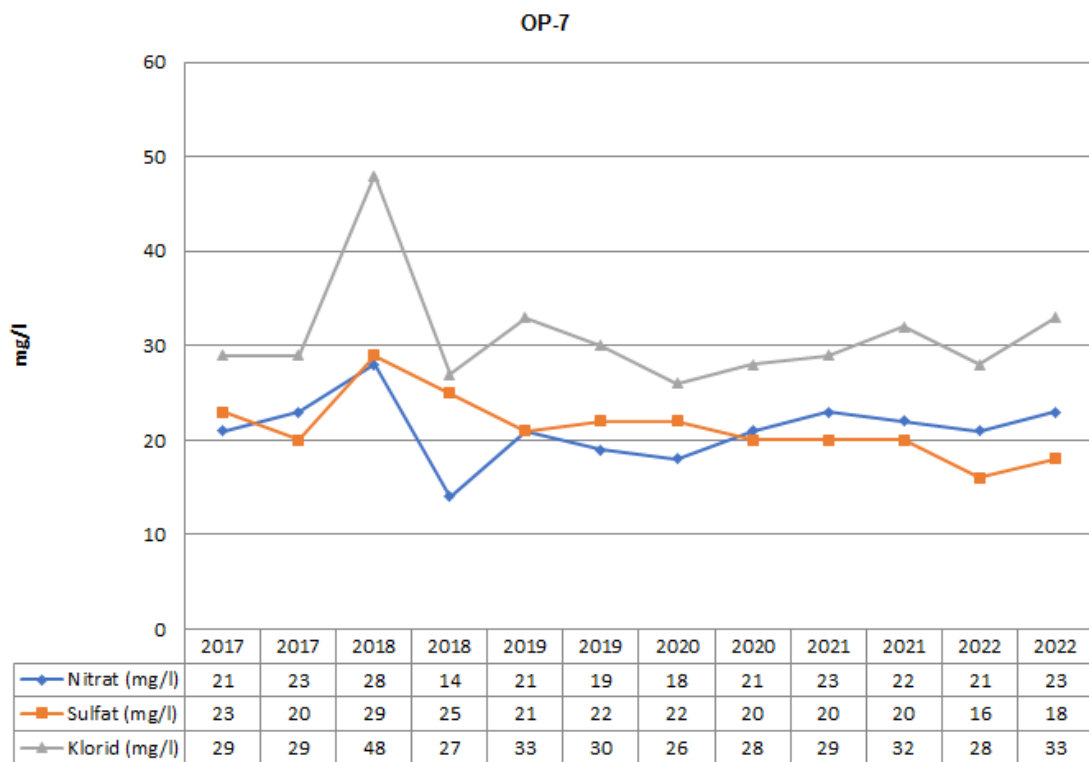
Slika 3-47: Nihanje vsebnosti nitrata, klorida in sulfata (mg/l) na merilnem mestu OP-7 v letih 2017-2022
