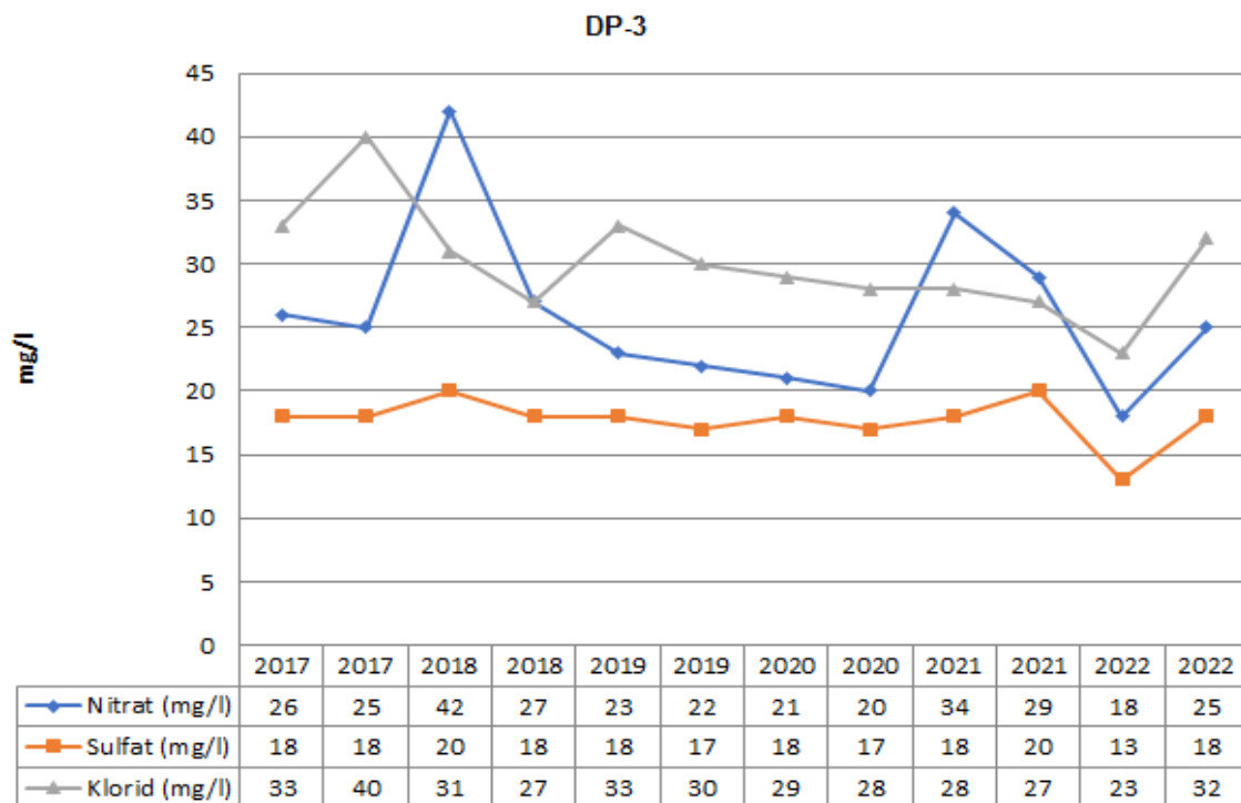
Slika 3-72: Vsebnost nitrata, sulfata in klorida (mg/l) v podzemni vodi na opazovalni vrtini DP-3 v letih 2017-2022
