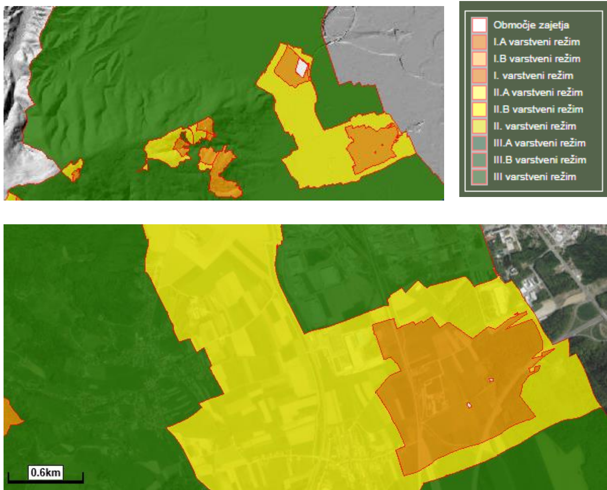
Slika 3-61: Črpališče Bohova s prispevnim območjem (vir: ARSO, Atlas okolja)
