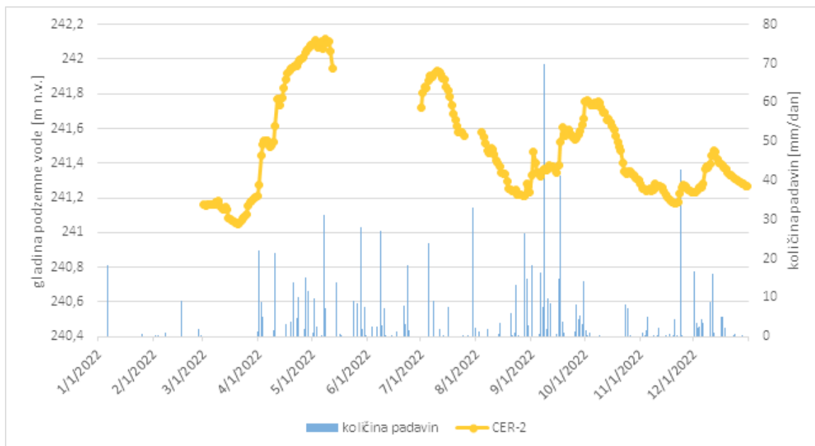
Slika 3-92: Grafični prikaz avtomatskih meritev gladin podzemne vode na merilnem mestu CER-2 (Ceršak) ter količina padavin izmerjenih na meteorološki postaji Vrbanski plato v letu 2022
