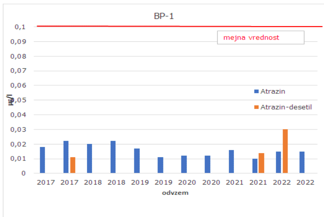
Slika 3-77: Vsebnost atrazina in atrazin-desetila (µg/l) v podzemni vodi na opazovalni vrtini BP-1 v letih 2017-2022
