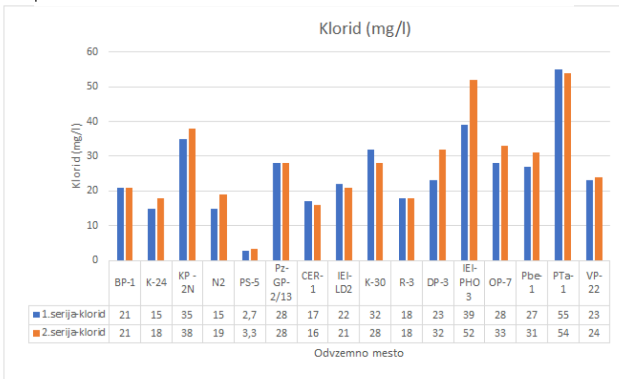
Slika 3-3: Prikaz izmerjenih vsebnosti klorida (mg/l) v letu 2022
