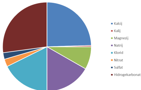
Slika 3-27: Ionska sestava vode na merilnem mestu KP-2
