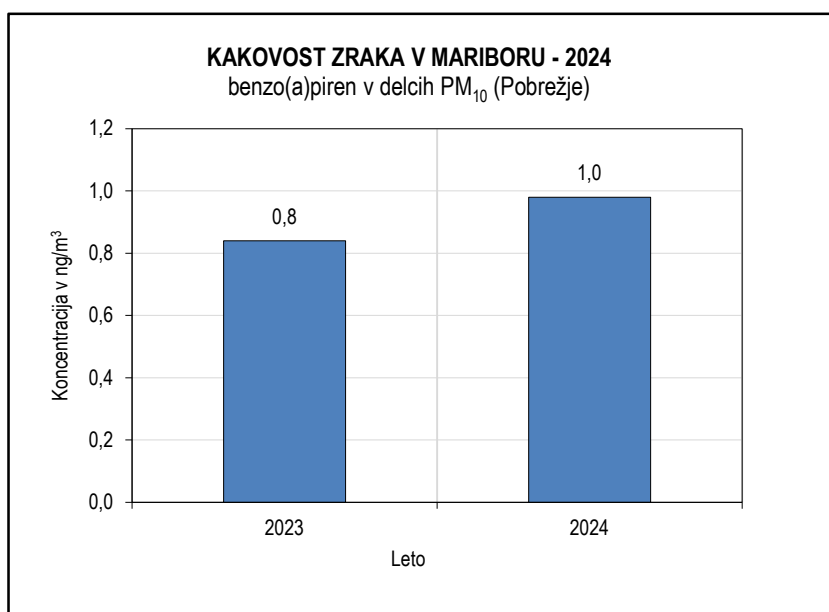
Slika 5.54: Benzo(a)piren v delcih PM 10 2023-2024, merilno mesto Pobrežje
