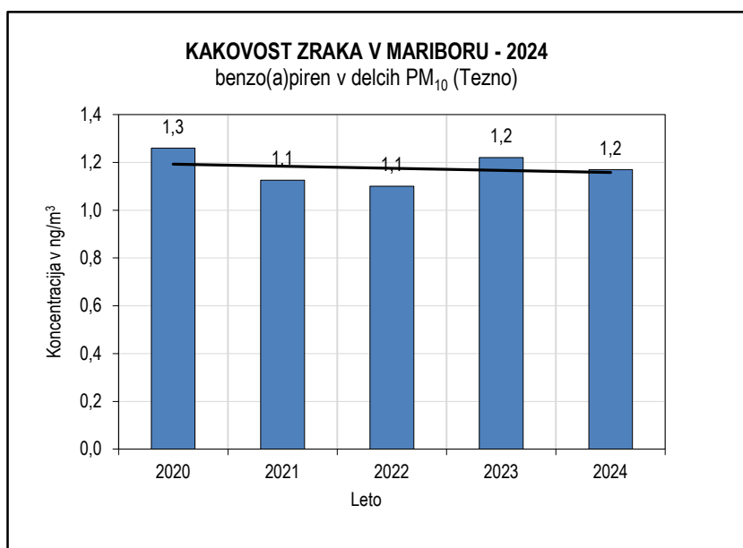
Slika 5.53: Benzo(a)piren v delcih PM 10 2020-2024, merilno mesto Tezno
