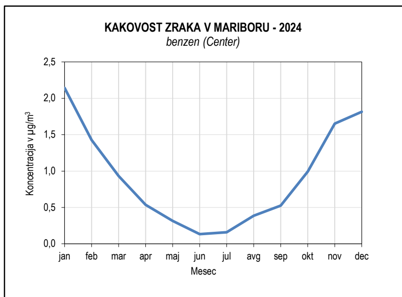
Slika 5.61: Mesečne koncentracije benzena, merilno mesto Center
