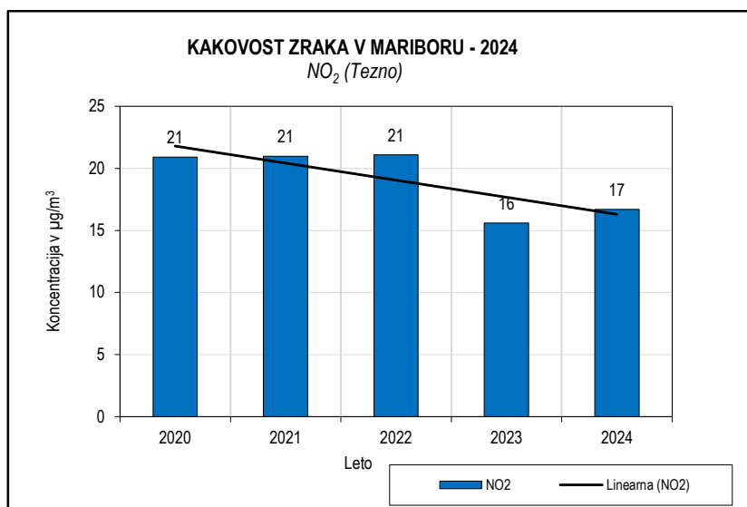
Slika 5.7: Dušikov dioksid 2020-2024, merilno mesto Tezno
