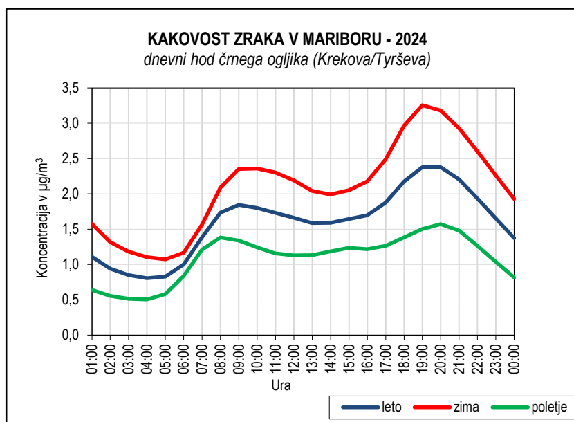
Slika 5.65: Dnevni hodi koncentracij črnega ogljika, merilno mesto Krekova/Tyrševa
