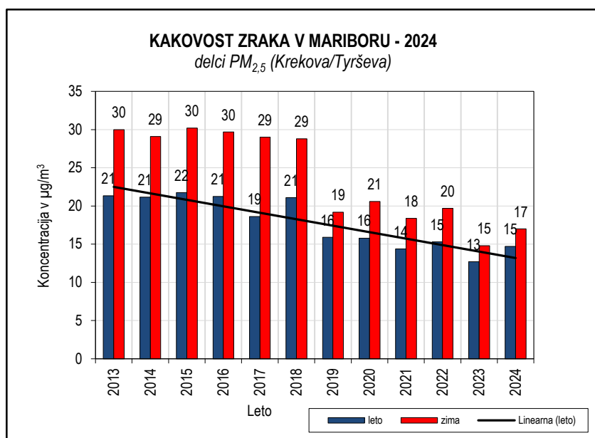
Slika 5.37: Delci PM_{2,5} 2013-2024, merilno mesto Krekova/Tyrševa
