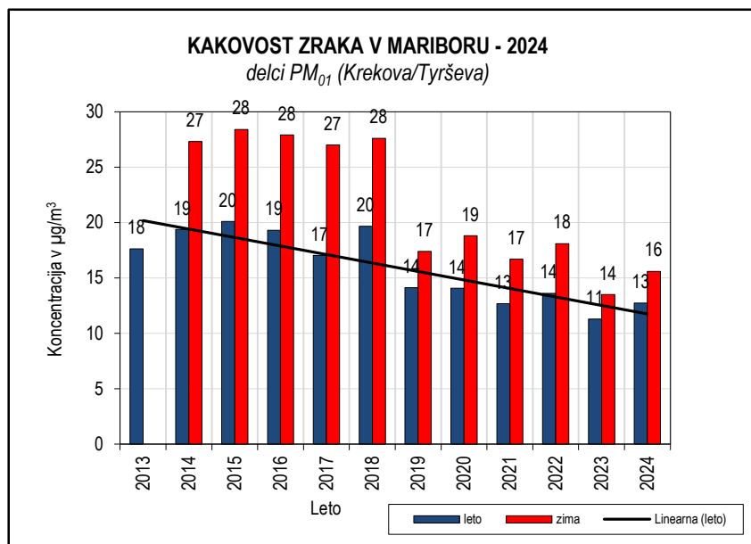
Slika 5.45: Delci PM_{01} 2013-2024, merilno mesto Krekova/Tyrševa
