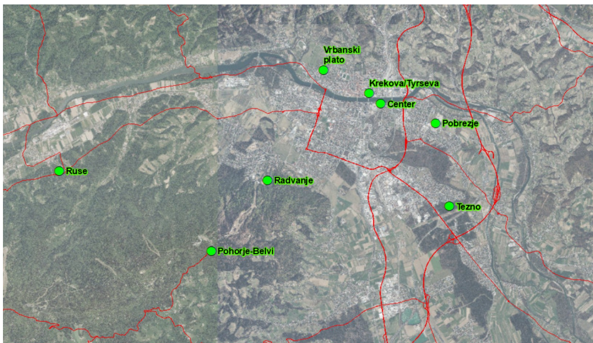
Slika 2.1: Stalna merilna mesta za spremljanje kakovosti zunanjega zraka v letu 2024
