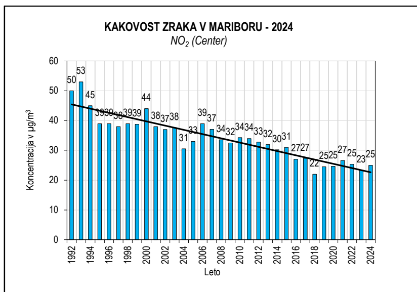
Slika 5.5: Dušikov dioksid 1992-2024, merilno mesto Center
