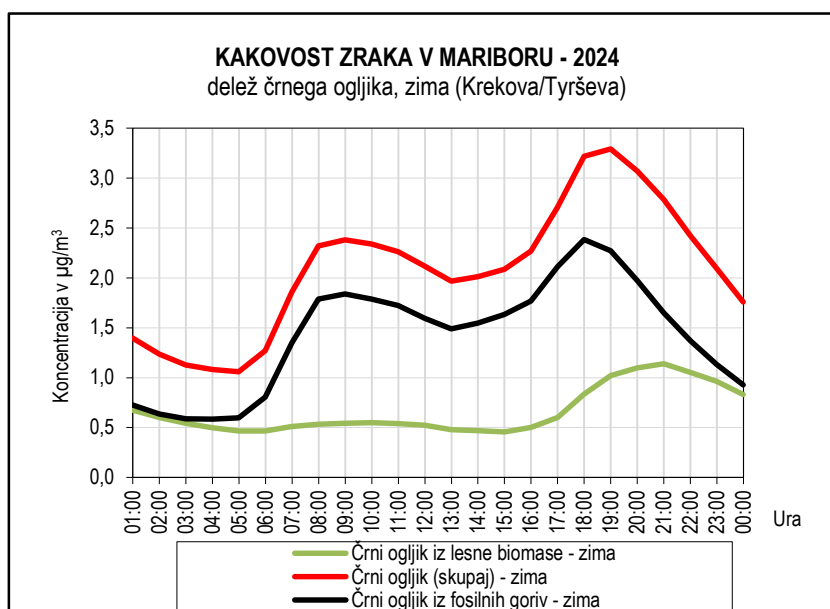
Slika 5.66: Dnevni hodi koncentracij skupnega črnega ogljika, črnega ogljika iz fosilnih goriv in črnega ogljika iz lesne biomase, pozimi, merilno mesto Krekova/Tyrševa
