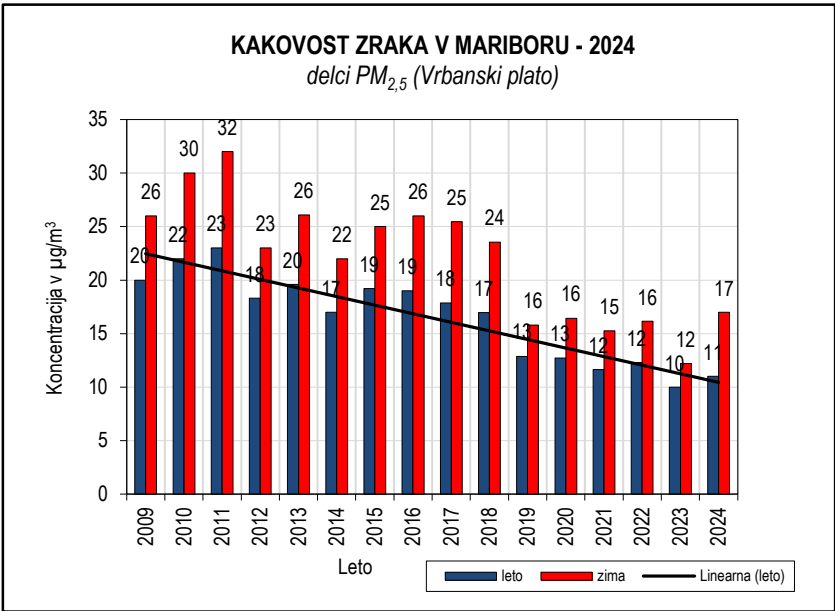
Slika 5.35: Delci PM 2,5 2009-2024, merilno mesto Vrbanski plato
