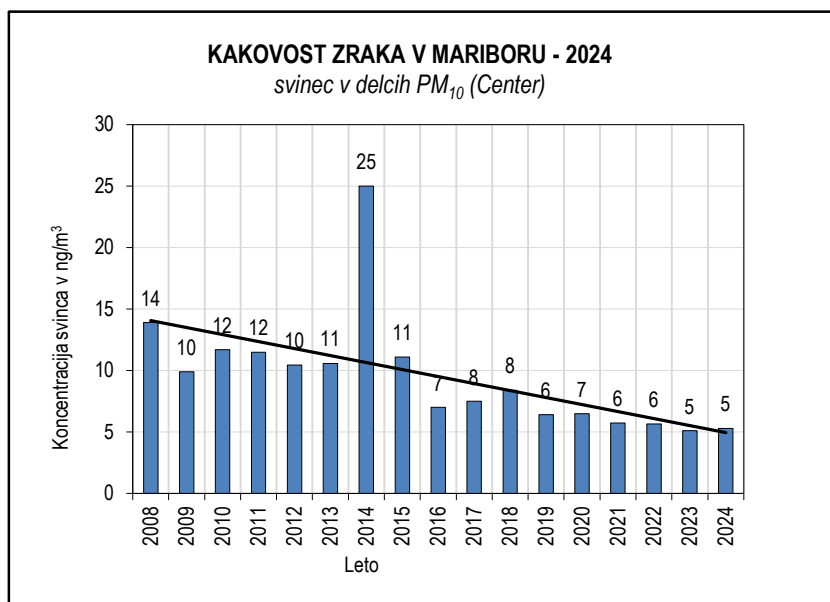
Slika 5.57: Svinec v delcih PM 10 2008-2024, merilno mesto Center
