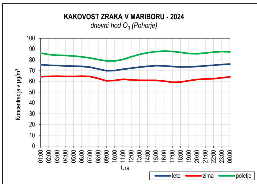
Slika 5.18: Dnevni hodi O_3 , merilno mesto Pohorje
