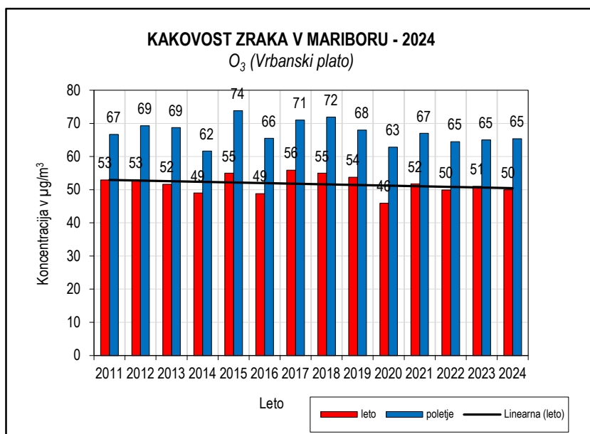
Slika 5.19: Ozon 2011-2024, merilno mesto Vrbanski plato
