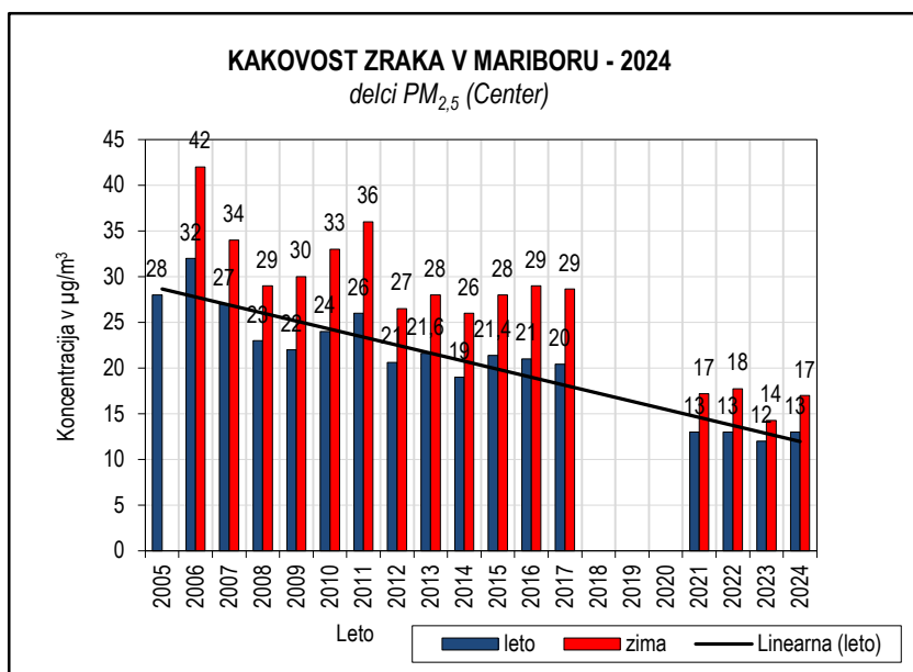
Slika 5.36: Delci PM_{2,5} 2005-2024, merilno mesto Center
