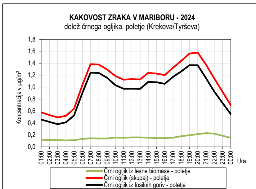
Slika 5.67: Dnevni hod koncentracij skupnega črnega ogljika, črnega ogljika iz fosilnih goriv in črnega ogljika iz lesne biomase, poleti, merilno mesto Krekova/Tyrševa
