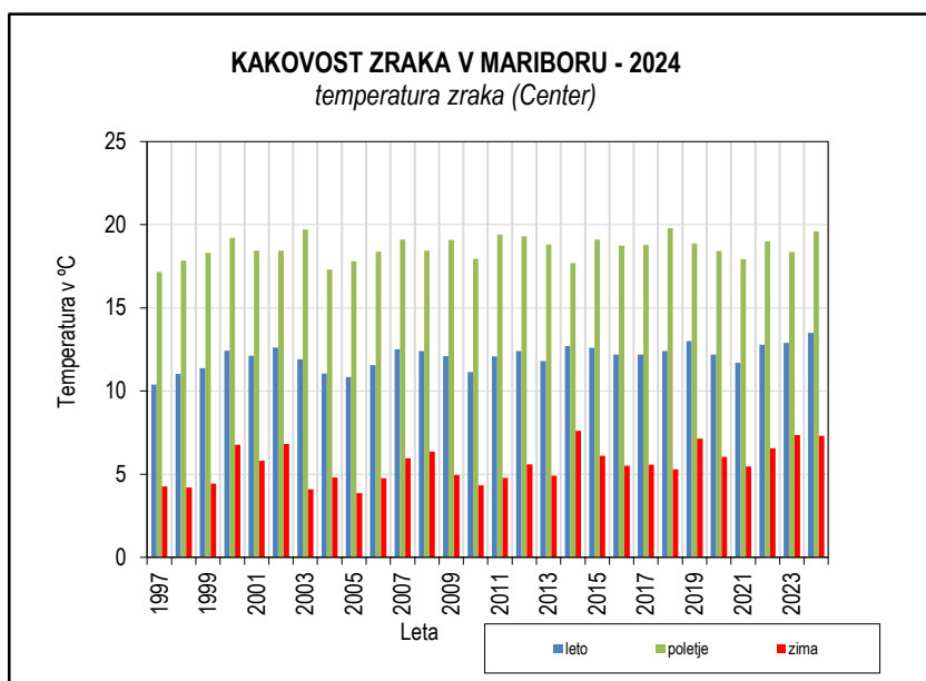
Slika 5.70: Temperatura zraka 1997-2024, merilno mesto Center
