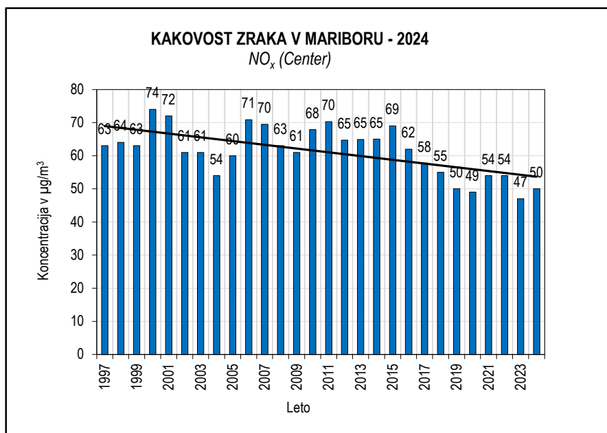
Slika 5.12: Dušikovi oksidi 1997-2024, merilno mesto Center
