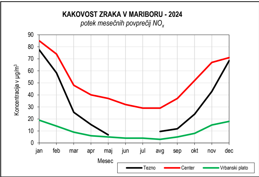
Slika 5.8: Koncentracije NO x , merilna mesta Center, Urbanski plato in Tezno
