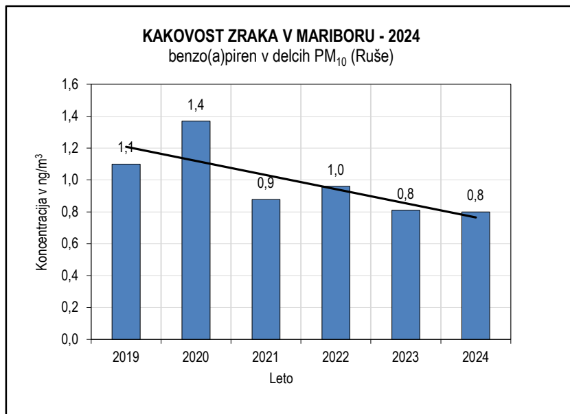
Slika 5.51: Benzo(a)piren v delcih PM 10 2019-2024, merilno mesto Ruše
