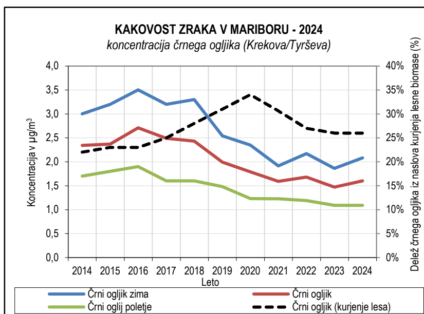
Slika 5.68: Skupni črni ogljik ter črni ogljik v zimskem in poletnem času, črni ogljik iz naslova kurjenja lesne biomase (BC (WB)), merilno mesto Krekova/Tyrševa
