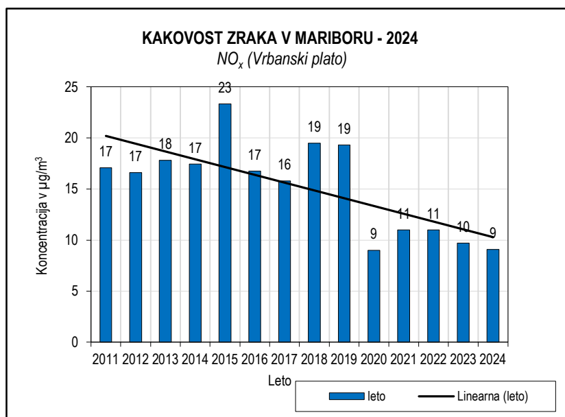
Slika 5.13: Dušikov oksidi 2011-2024, merilno mesto Vrbanski plato
