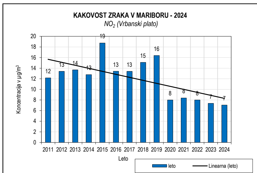
Slika 5.6: Dušikov dioksid 2011-2024, merilno mesto Vrbanski plato
