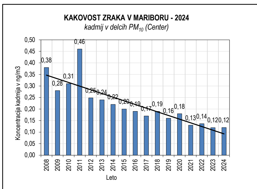
Slika 5.59: Kadmij v delcih PM 10 2008-2024, merilno mesto Center
