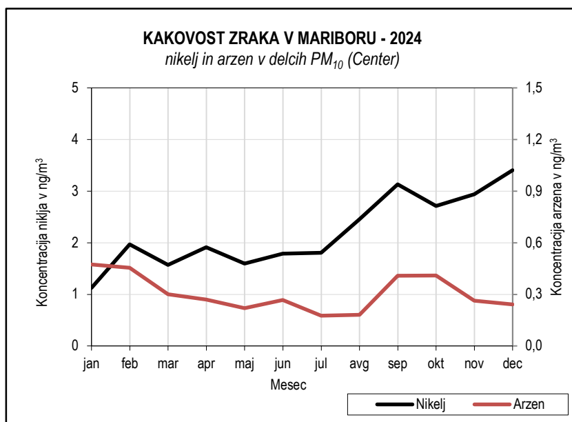
Slika 5.56: Mesečne koncentracije niklja in arzena v delcih PM 10 , merilno mesto Center
