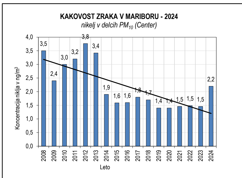
Slika 5.58: Nikelj v delcih PM 10 2008-2024, merilno mesto Center
