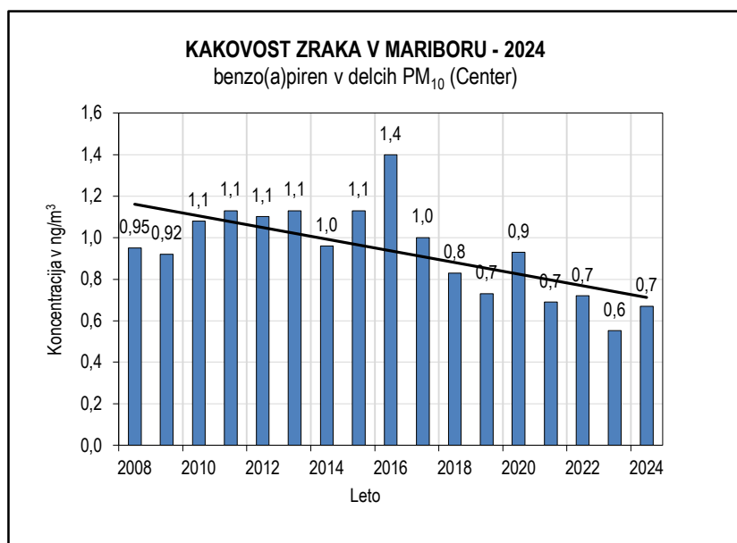
Slika 5.50: Benzo(a)piren v delcih PM 10 2008-2024, merilno mesto Center
