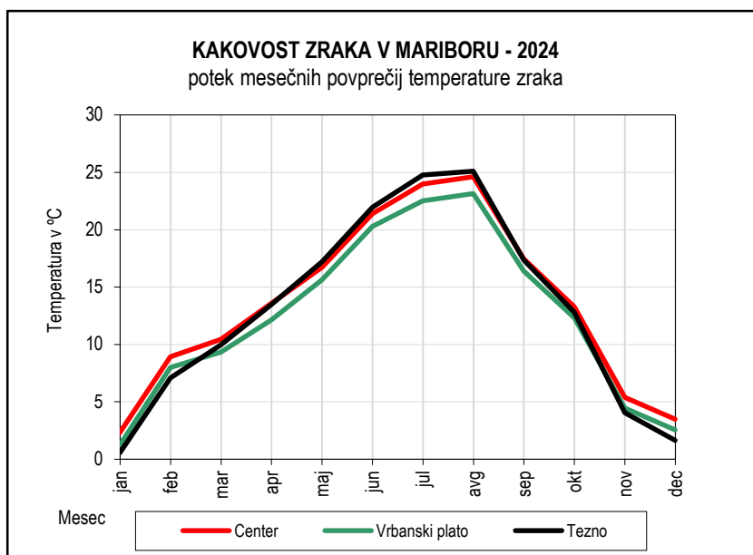
Slika 5.69: Mesečne temperature zraka, merilna mesta Center, Vrbanški plato in Tezno
