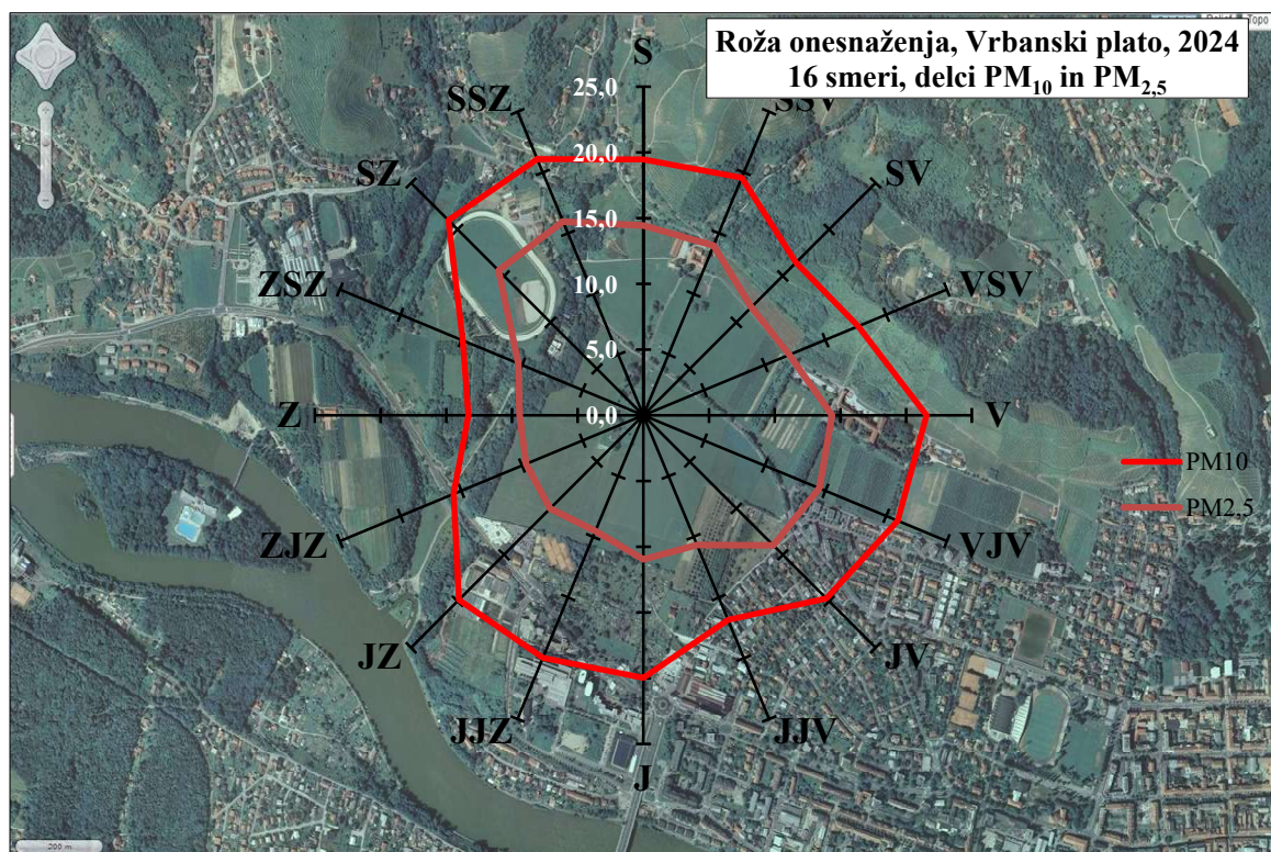
Slika 5.74: Roža onesnaženja zunanjega zraka z delci \text{PM}_{10} in \text{PM}_{2,5} v letu 2024, merilno mesto Vrbanski plato
