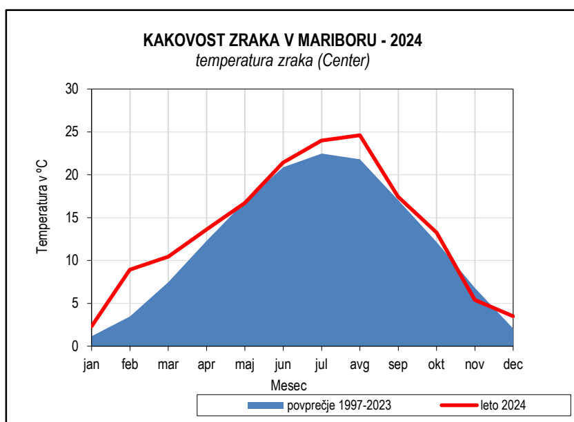
Slika 5.71: Odstopanje mesečne temperature zraka v letu 2024 od povprečja 1997-2023, merilno mesto Center
