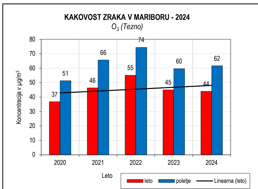
Slika 5.21: Ozon 2020-2024, merilno mesto Tezno
