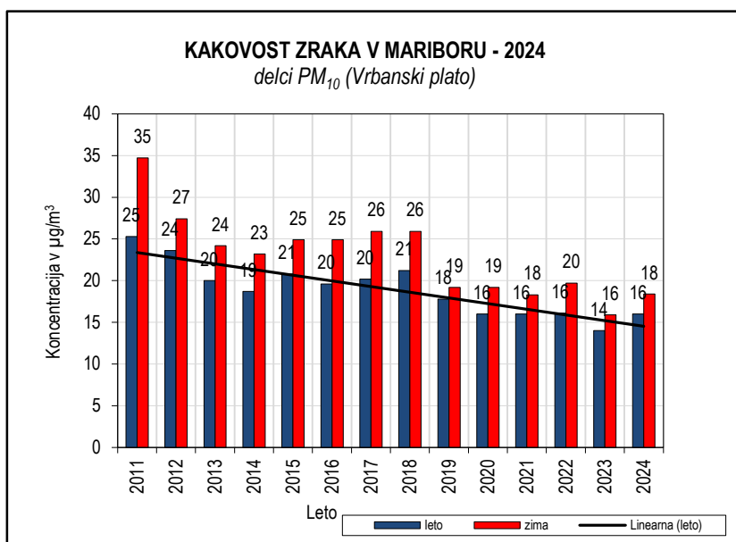
Slika 5.29: Delci PM_{10} 2011-2024, merilno mesto Vrbanski plato
