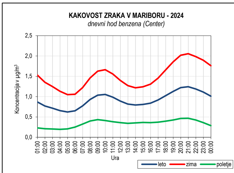
Slika 5.62: Dnevni hodi koncentracij benzena, merilno mesto Center
