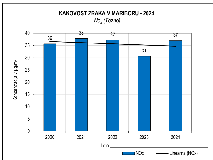
Slika 5.14: Dušikov oksidi 2020-2024, merilno mesto Tezno
