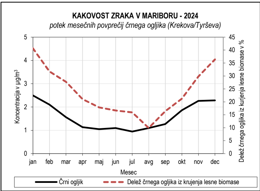
Slika 5.64: Mesečne koncentracije črnega ogljika in njegov delež iz kurjenja lesne biomase, merilno mesto Krekova/Tyrševa
