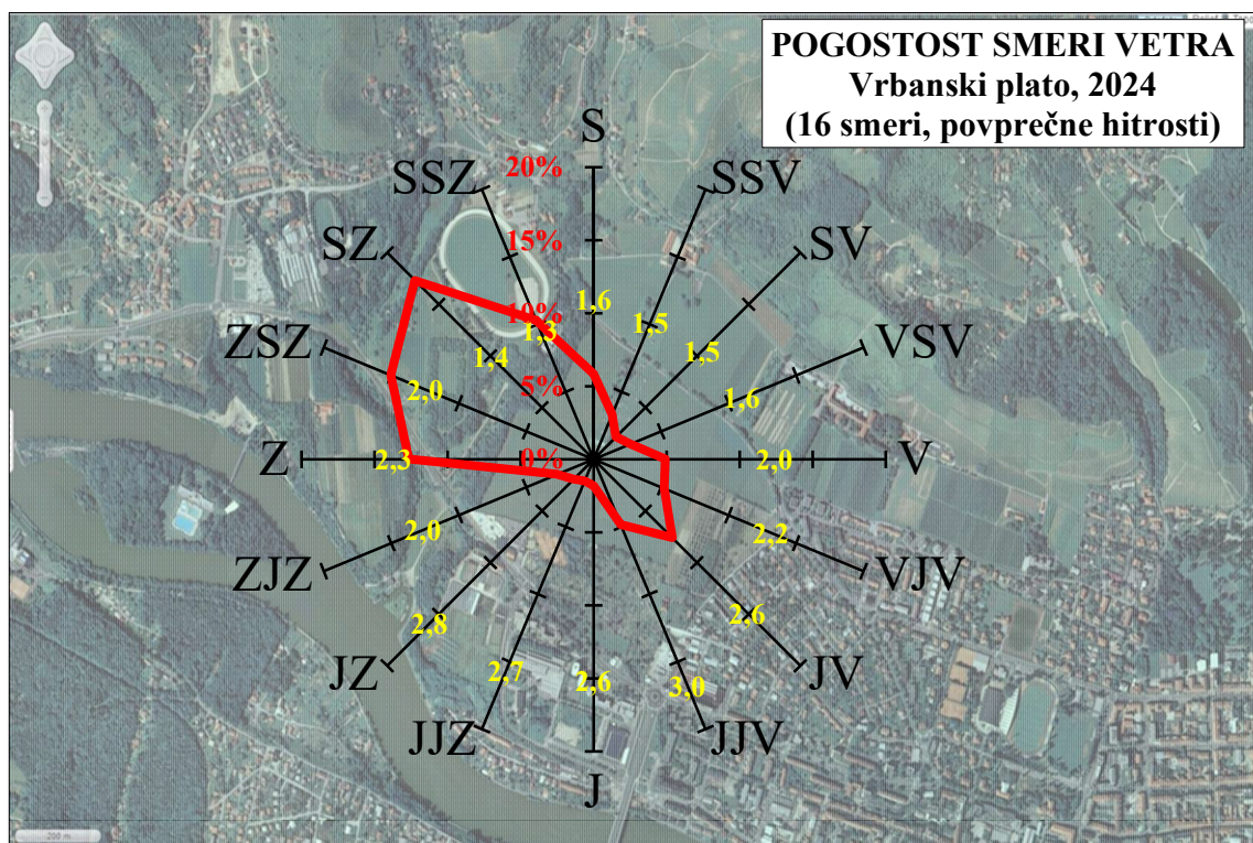
Slika 5.72: Pogostost pojavljanja smeri vetra in povprečna hitrost po smereh, leto 2024, merilno mesto Vrbanski plato
