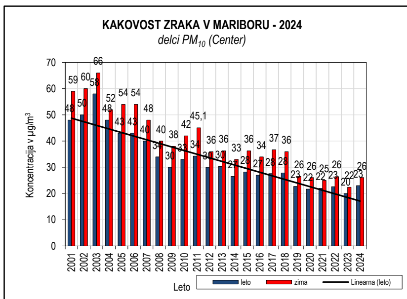
Slika 5.28: Delci PM_{10} 2001-2024, merilno mesto Center (DMKZ)
