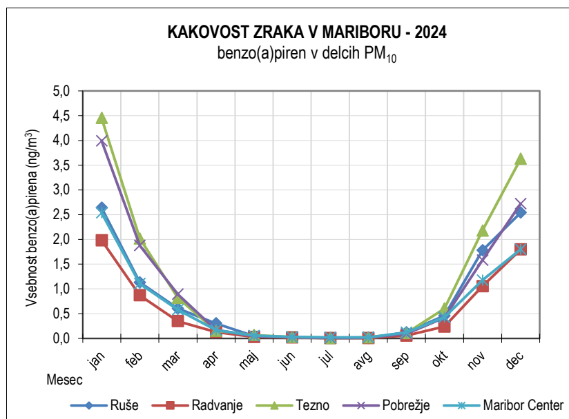
Slika 5.49: Benzo(a)piren v delcih PM 10 , merilna mesta Center, Radvanje, Tezno, Ruše ter Pobrežje
