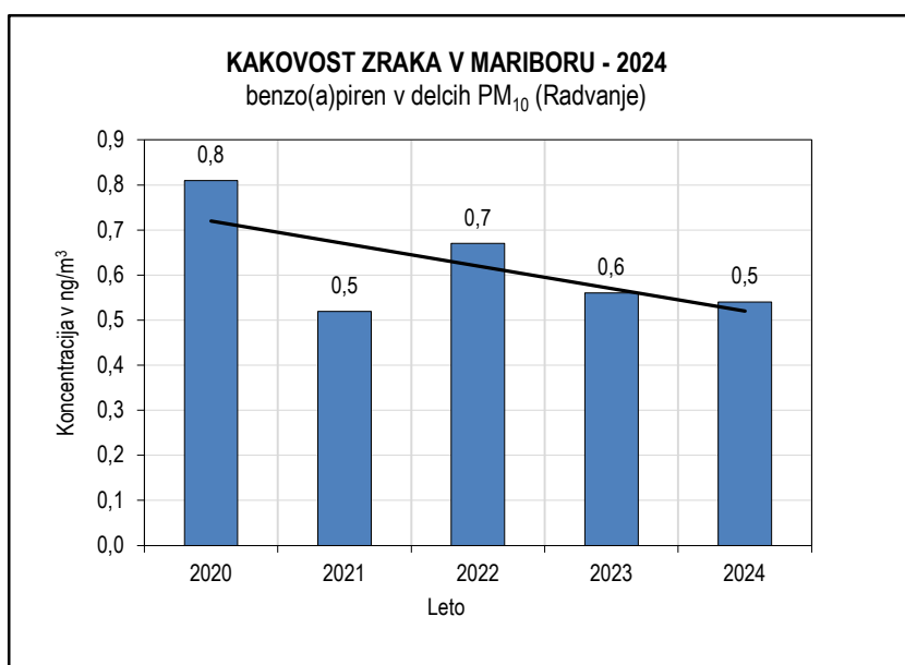
Slika 5.52: Benzo(a)piren v delcih PM 10 2020-2024, merilno mesto Radvanje
