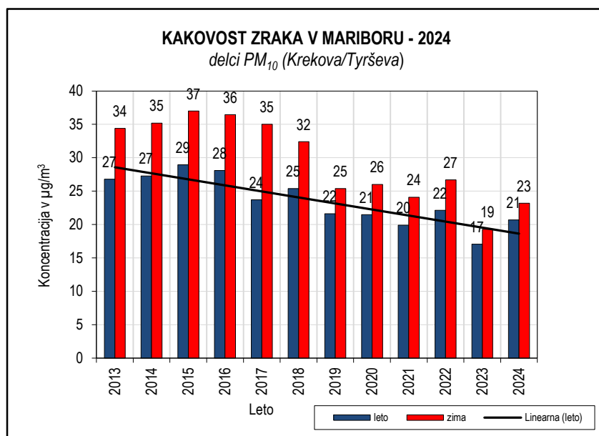
Slika 5.32: Delci PM_{10} 2013-2024, merilno mesto Krekova/Tyrševa
