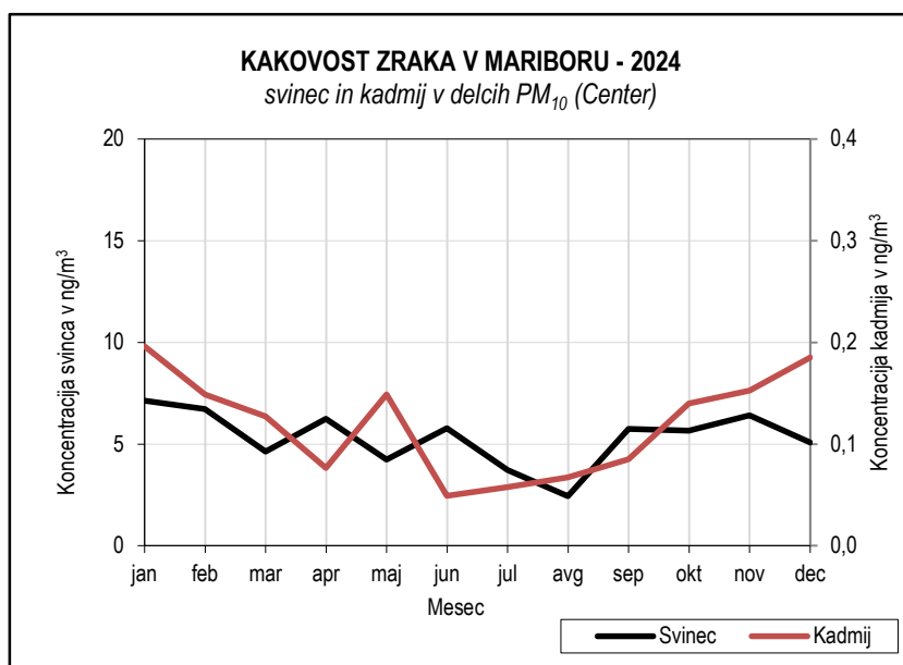
Slika 5.55: Mesečne koncentracije svinca in kadmija v delcih PM 10 , merilno mesto Center
