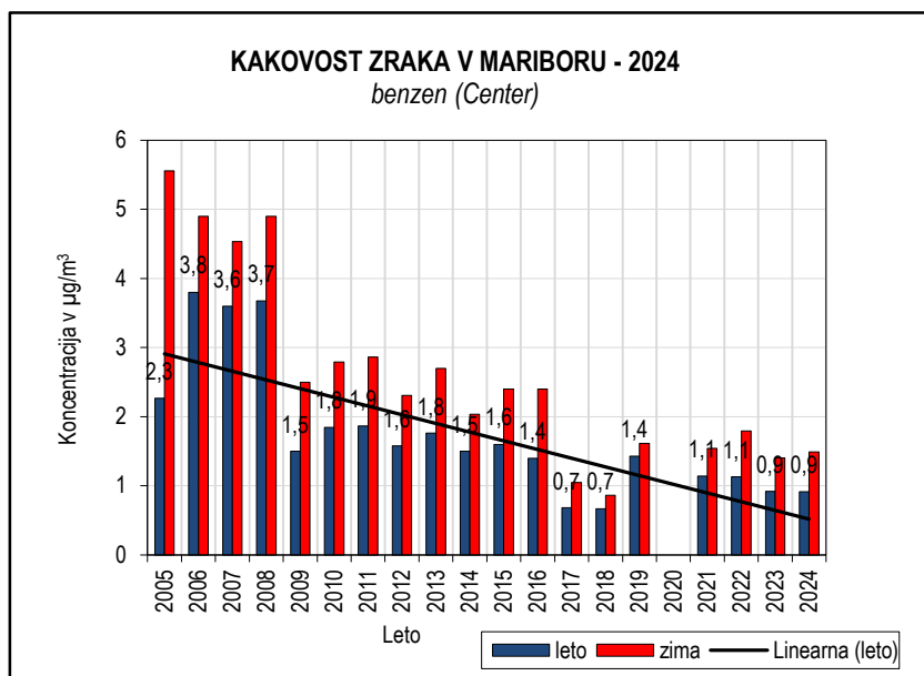
Slika 5.63: Benzen 2005-2024, merilno mesto Center
