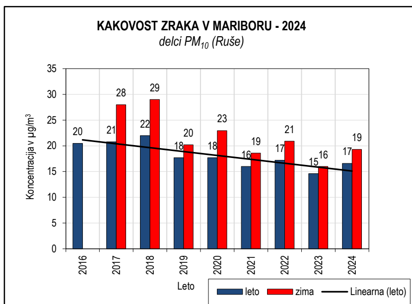
Slika 5.30: Delci PM_{10} 2016-2024, merilno mesto Ruše
