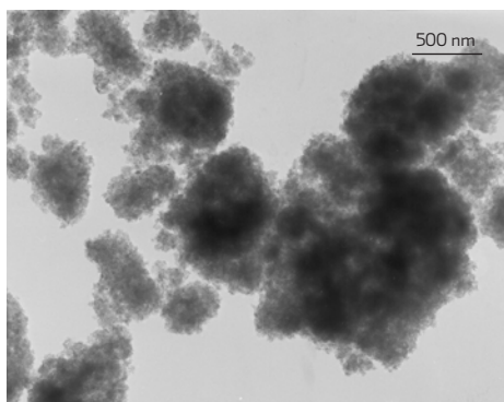
Slika 20: \text{TiO}_2 v anatasni obliki. Visokoločljivostna presevoelektronsko-mikroskopska slika posameznega nanodelca (levo); spontana aglomeracija nanodelcev v velike gručice (desno). (avtorica: Maja Remškar, IJS)
