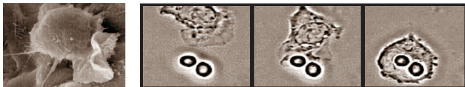
Slika 6: Vrstičnoelektronmikroskopska slika površine celice makrofaga s premerom 20 mm in jasno vidnimi podolgovatimi izrastki (leva slika); proces ujetja dveh delcev in njuna imobilizacija znotraj celice makrofaga (desna slika) (avtor: Jonathan Grigg, University of Leicester, Velika Britanija)
