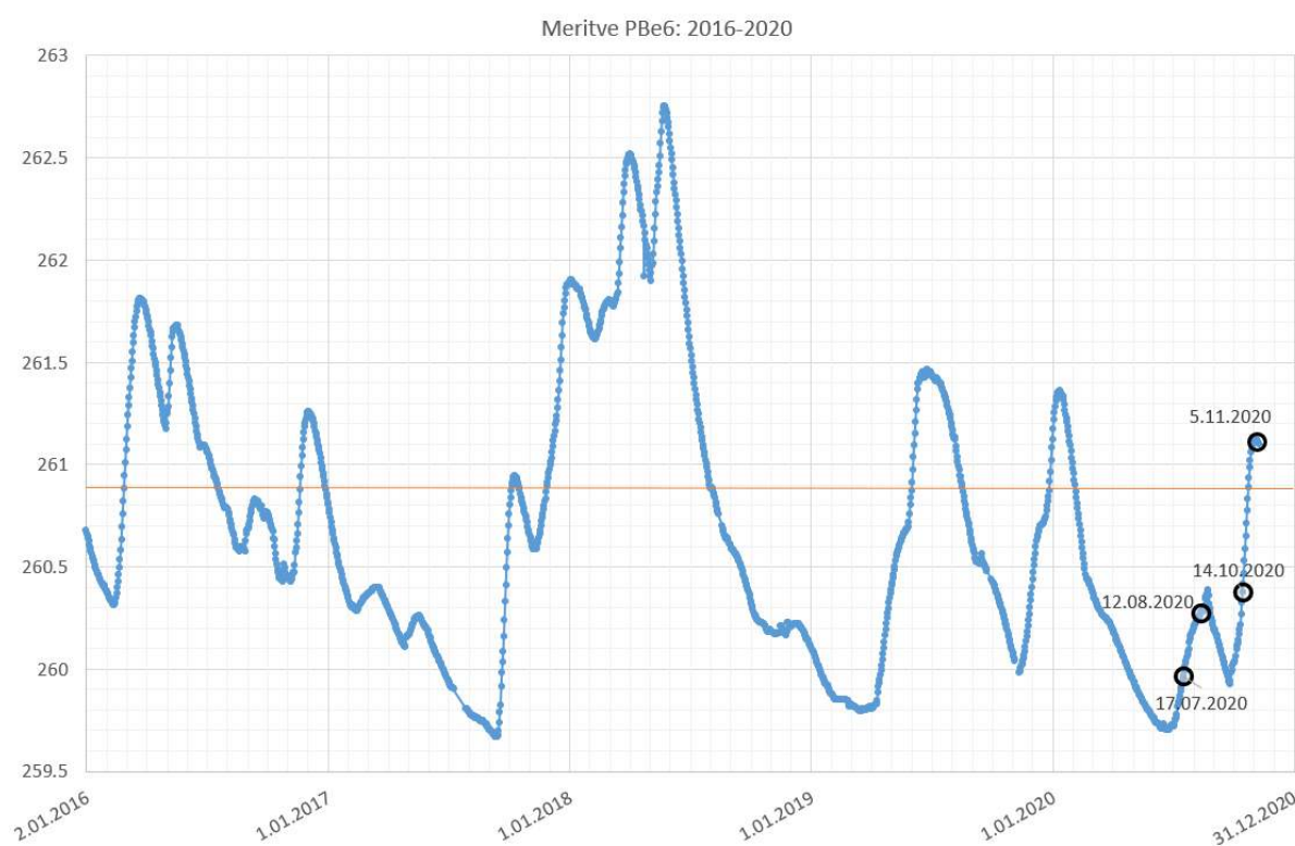
Slika 9. Meritve GPV na piezometru PBe6 v zaledju Stražunskega gozda med leti 2016-2020, prikaz srednje vrednosti (oranžna črta) in obdobja izvajanja terenskih meritev v letu 2020.
