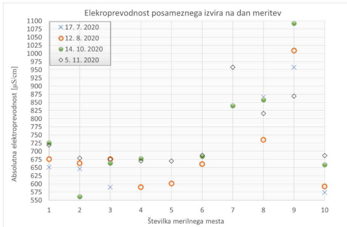
Slika 22. Meritve elektroprevodnosti (na y skali) in temperature (oznake podatkov) na dan meritev.
