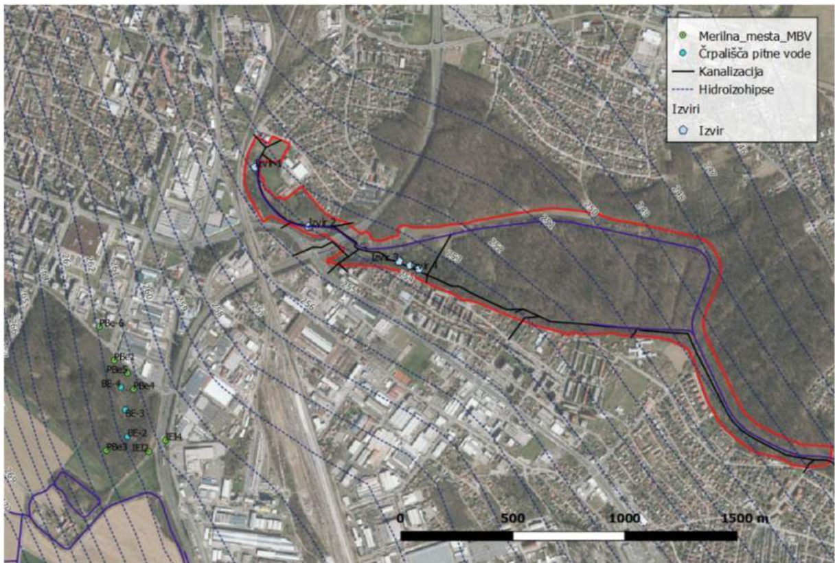
Slika 2. Prikaz merilnih mest z arhivskimi podatki o gladinah podzemne vode v zaledju Stražunskega gozda.
