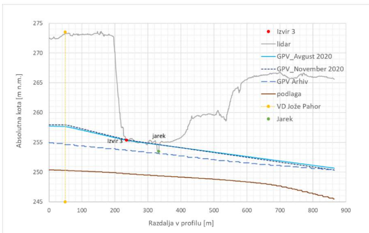
Slika 15. Profil 2 (smer: jug-sever)
