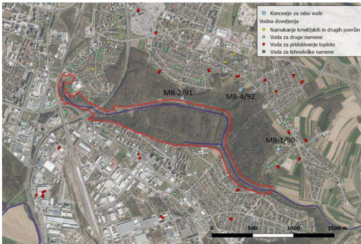
Slika 4. Prikaz vrtin s koncesijo in vodnimi dovoljenji.
