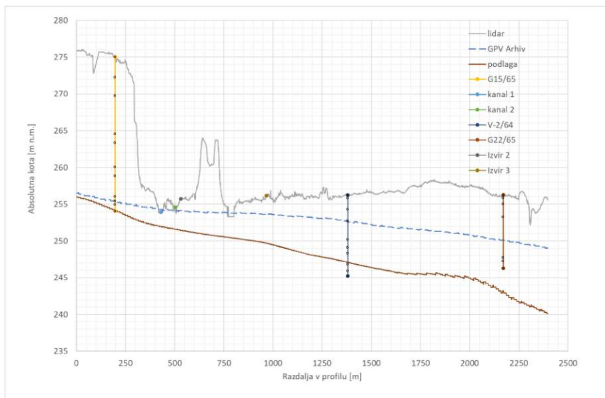
Slika 18. Vzdolžni profil (smer: zahod-vzhod)
