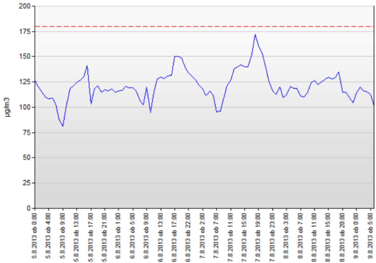
Graf: Koncentracije ozona na lokaciji Maribor Pohorje v obdobju od 5.8.-9.8.2013
