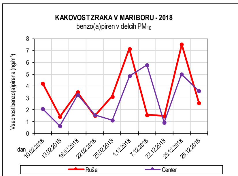
Slika 5.40: Benzo(a)piren v delcih PM 10 , merilni mesti Ruše in Center
