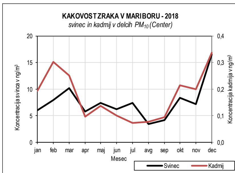
Slika 5.41: Mesečne koncentracije svineca in kadmija v delcih PM 10 , merilno mesto Center
