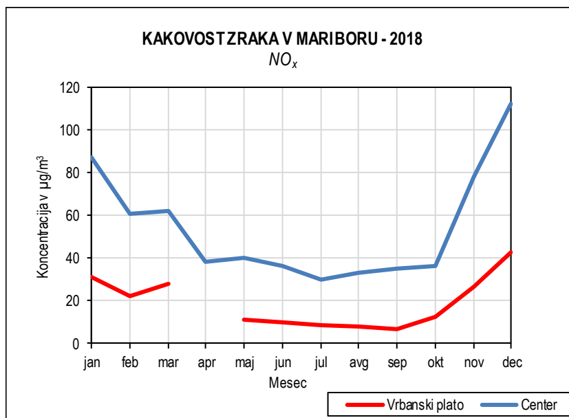
Slika 5.6: Koncentracije NO x , merilni mesti Center in Vrbanški plato
