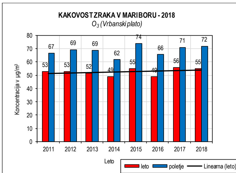
Slika 5.14: Ozon 2011-2018, merilno mesto Vrbanski plato
