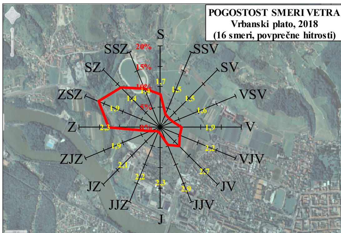
Slika 5.61: Pogostost pojavljanja smeri vetra in povprečne hitrosti po smereh, leto 2018, merilno mesto Vrbanski plato
