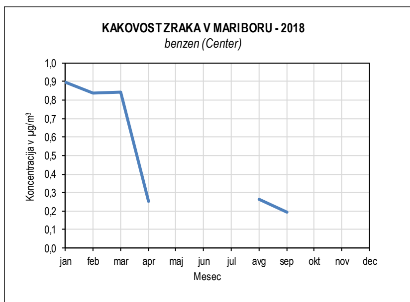
Slika 5.50: Mesečne koncentracije benzena, merilno mesto Center
