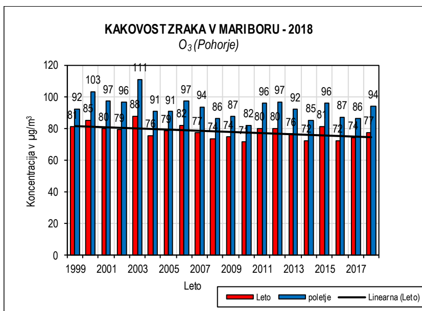
Slika 5.15: Ozon 1999-2018, merilno mesto Pohorje
