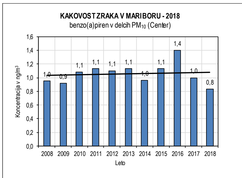
Slika 5.38: Benzo(a)piren v delcih PM 10 2008-2018, merilno mesto Center
