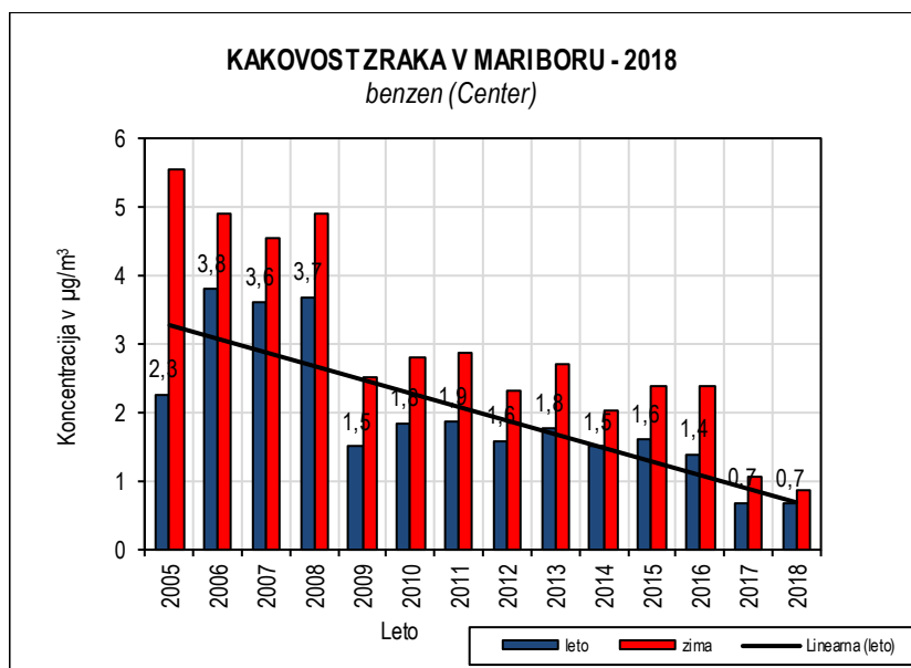
Slika 5.52: Benzen 2005-2018, merilno mesto Center
