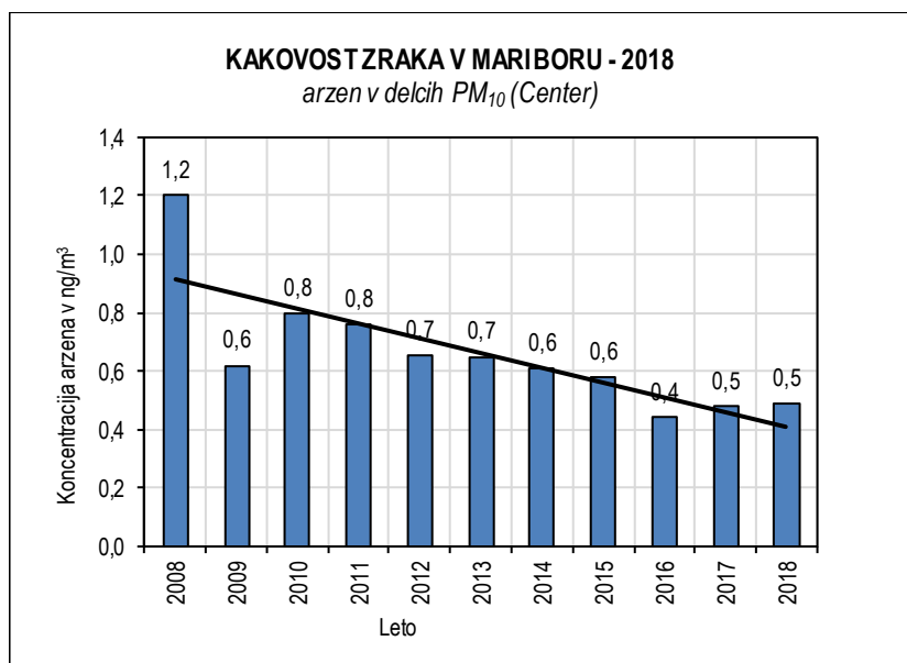
Slika 5.46: Arzen v delcih PM 10 2008-2018, merilno mesto Center
