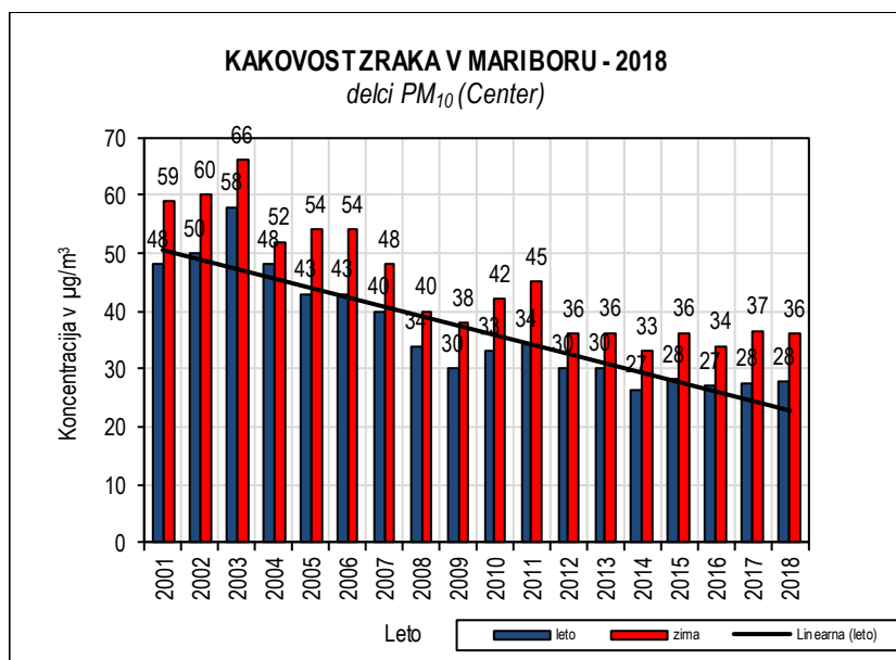
Slika 5.22: Delci PM_{10} 2001-2018, merilno mesto Center (DMKZ)
