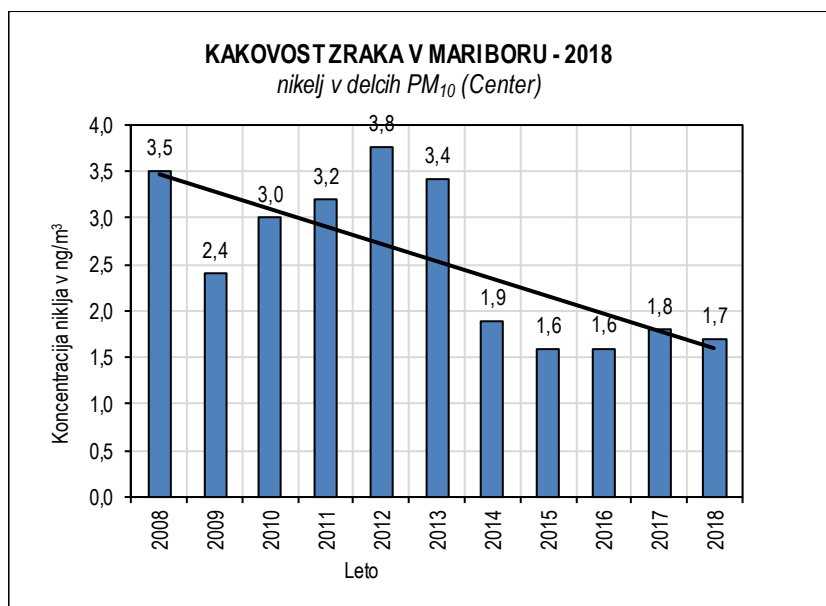
Slika 5.44: Nikelj v delcih PM 10 2008-2018, merilno mesto Center
