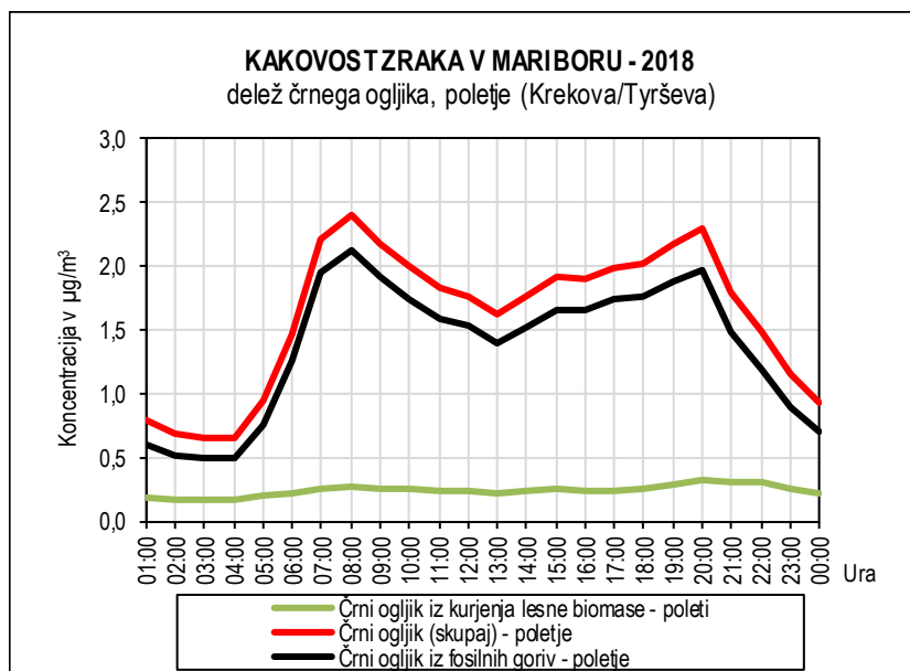
Slika 5.56: Dnevni hod koncentracij črnega ogljika iz fosilnih goriv in lesne biomase, poleti, merilno mesto Krekova/Tyrševa
