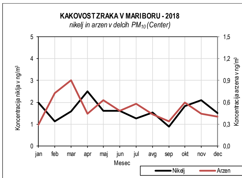
Slika 5.42: Mesečne koncentracije niklja in arzena v delcih PM 10 , merilno mesto Center
