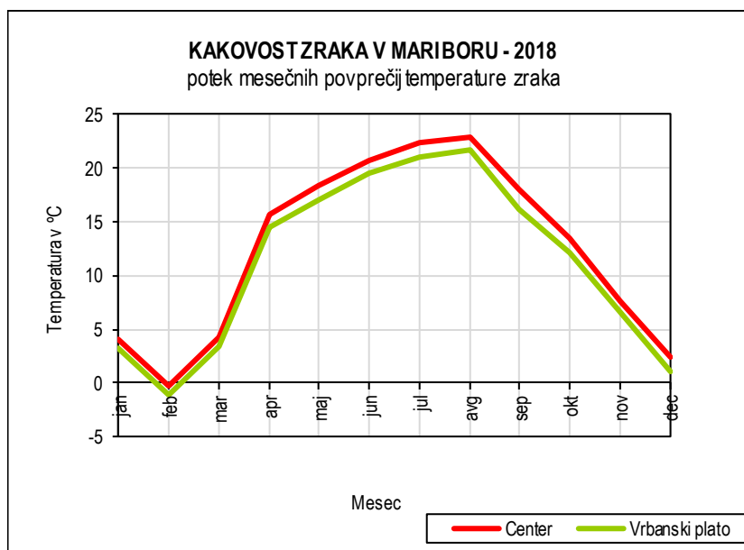
Slika 5.58: Mesečne temperature zraka, merilni mesti Center in Vrbanski plato
