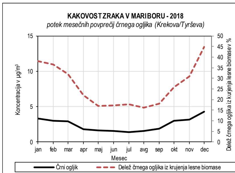
Slika 5.53: Mesečne koncentracije črnega ogljika in njegov delež iz kurjenja lesne biomase, merilno mesto Center
