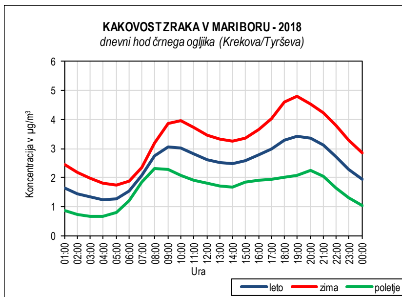
Slika 5.54: Dnevni hodi koncentracij črnega ogljika, merilno mesto Krekova/Tyrševa
