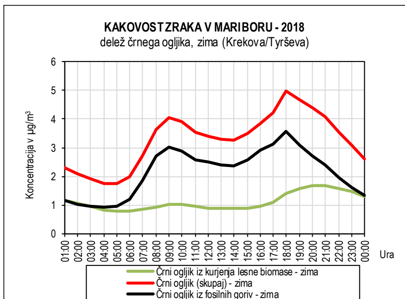
Slika 5.55: Dnevni hodi koncentracij črnega ogljika iz fosilnih goriv in lesne biomase, pozimi, merilno mesto Krekova/Tyrševa
