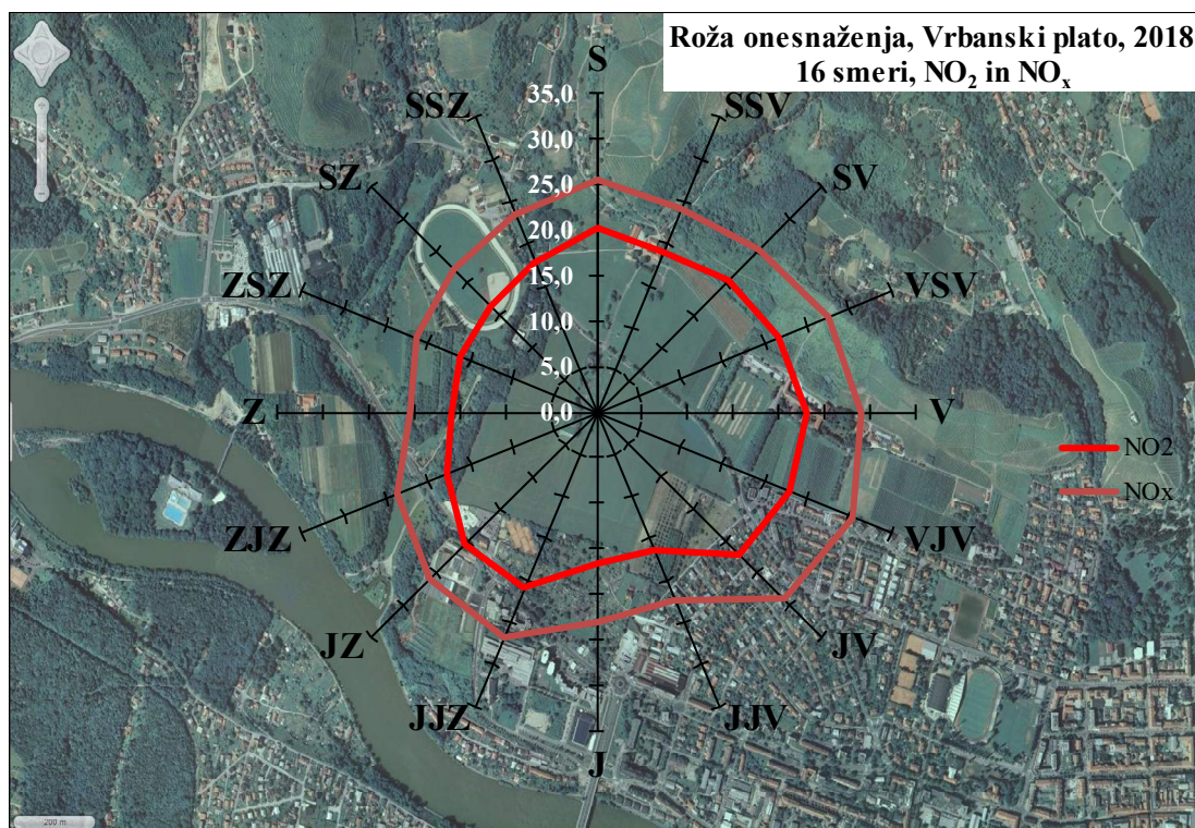
Slika 5.62: Roža kakovosti zraka za NO x in NO 2 v letu 2018, merilno mesto Vrbanski plato
