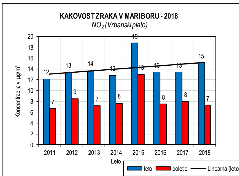
Slika 5.5: Dušikov dioksid 2011-2018, merilno mesto Vrbanjski plato
