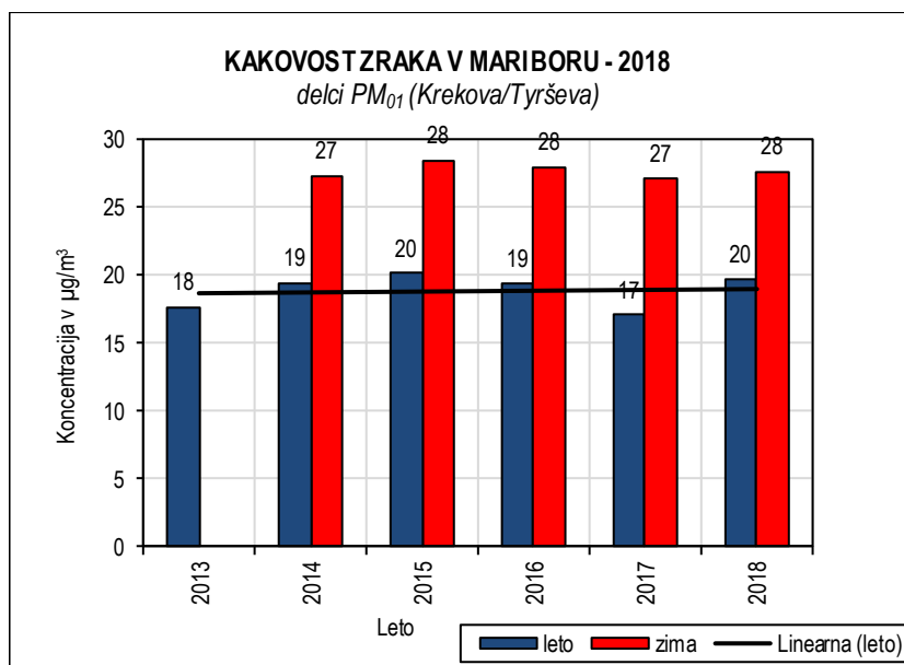
Slika 5.34: Delci PM_{01} 2013-2018, merilno mesto Krekova/Tyrševa
