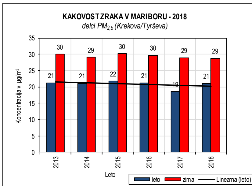
Slika 5.30: Delci PM_{2,5} 2009-2018, merilno mesto Krekova/Tyrševa
