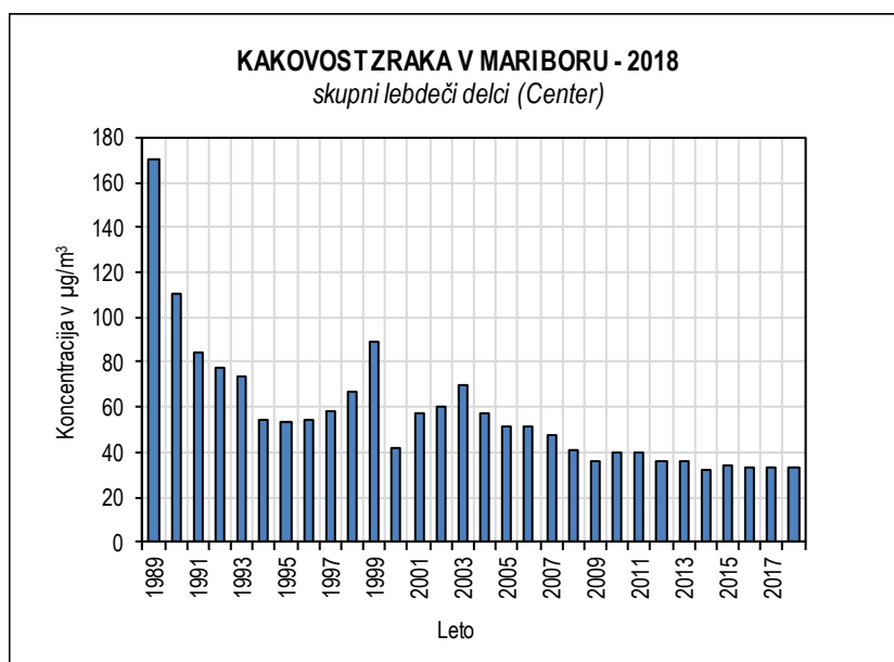
Slika 5.21: Skupni lebdeči delci 1989-2018, merilni mesti Center (ZZV (NLZOH) in DMKZ)
