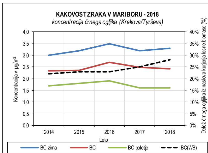
Slika 5.57: Skupni črni ogljik, črni ogljik iz naslova fosilnih goriv in lesne biomase ter delež črnega ogljika iz naslova kurjenja lesne biomase (BC (WB)), merilno mesto Krekova/Tyrševa
