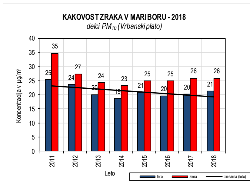
Slika 5.23: Delci PM_{10} 2011-2018, merilno mesto Vrbanski plato
