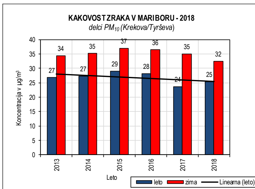
Slika 5.27: Delci PM 10 2013-2018, merilno mesto Krekova/Tyrševa
