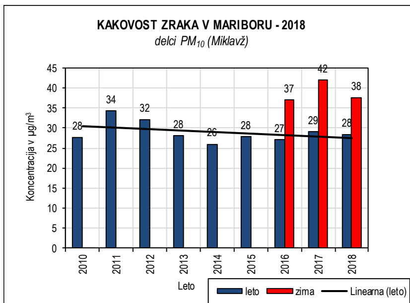
Slika 5.24: Delci PM_{10} 2010-2018, merilno mesto Miklavž
