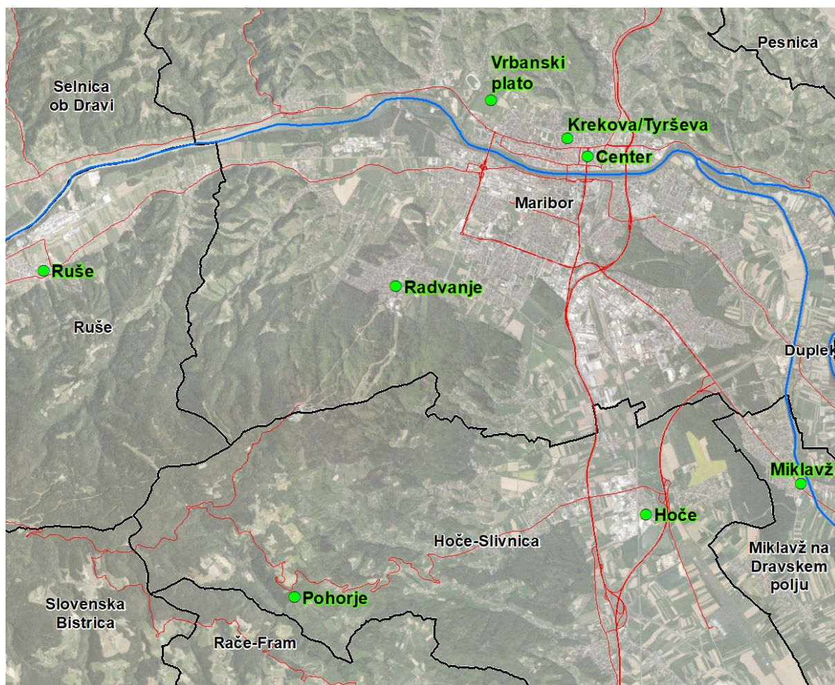
Slika 2.1: Stalna merilna mesta za spremljanje kakovosti zraka v letu 2018
