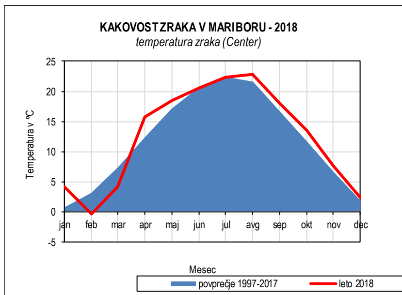
Slika 5.60: Odstopanje mesečne temperature zraka v letu 2018 od povprečja 1997-2017, merilno mesto Center
