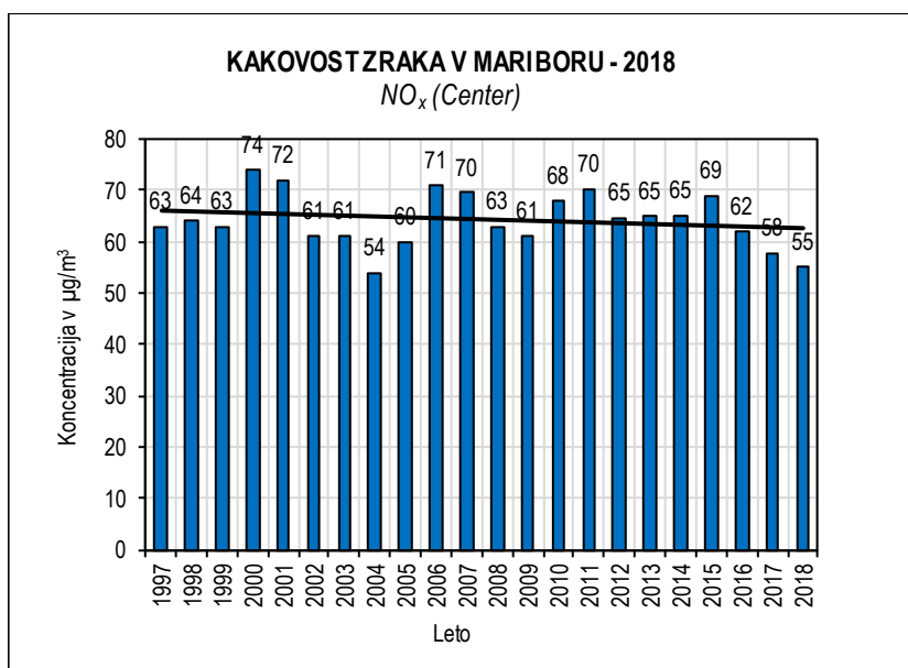
Slika 5.9: Dušikovi oksidi 1997-2018, merilno mesto Center
