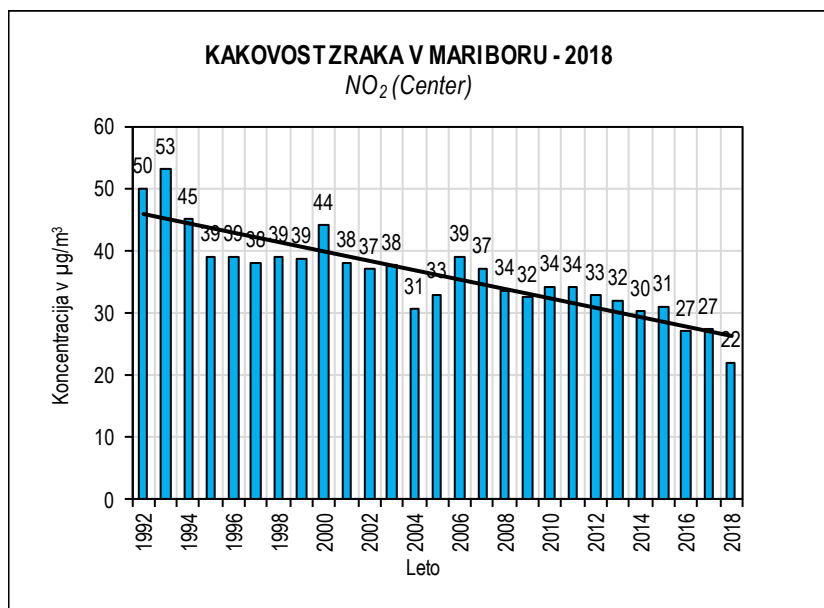
Slika 5.4: Dušikov dioksid 1992-2018, merilno mesto Center
