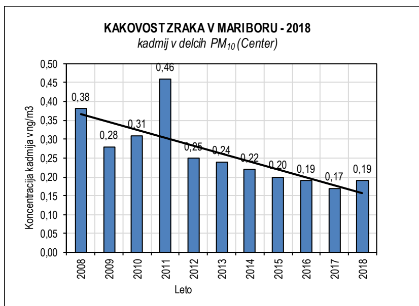
Slika 5.45: Kadmij v delcih PM 10 2008-2018, merilno mesto Center
