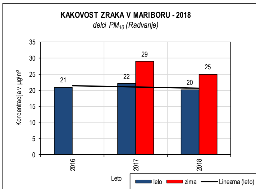
Slika 5.26: Delci PM 10 2016-2018, merilno mesto Radvanje
