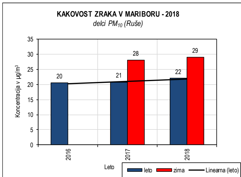
Slika 5.25: Delci PM_{10} 2016-2018, merilno mesto Ruše
