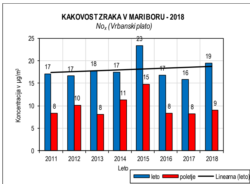
Slika 5.10: Dušikov dioksid 2011-2018, merilno mesto Vrbanski plato
