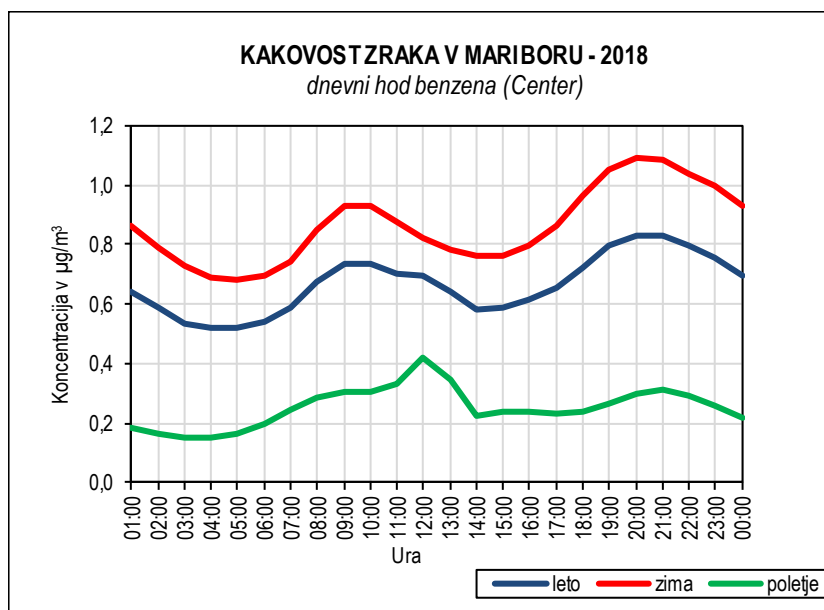
Slika 5.51: Dnevni hodi koncentracij benzena, merilno mesto Center
