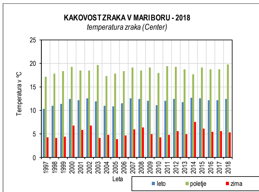
Slika 5.59: Temperatura zraka 1997-2018, merilno mesto Center
