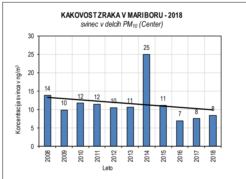
Slika 5.43: Svinec v delcih PM 10 2008-2018, merilno mesto Center
