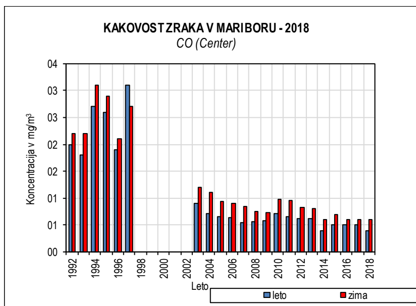
Slika 5.49: Ogljikov monoksid 1992-2018, merilno mesto Center
