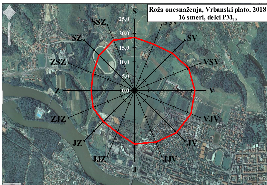
Slika 5.63: Roža kakovosti zraka za delce PM 10 v letu 2018, merilno mesto Vrbanski plato
