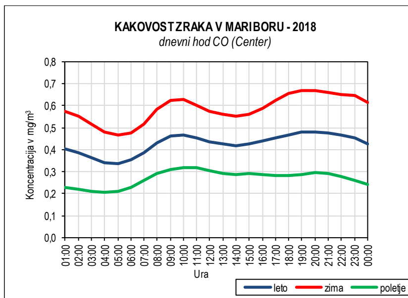
Slika 5.48: Dnevni hodi koncentracij ogljikovega monoksida, merilno mesto Center
